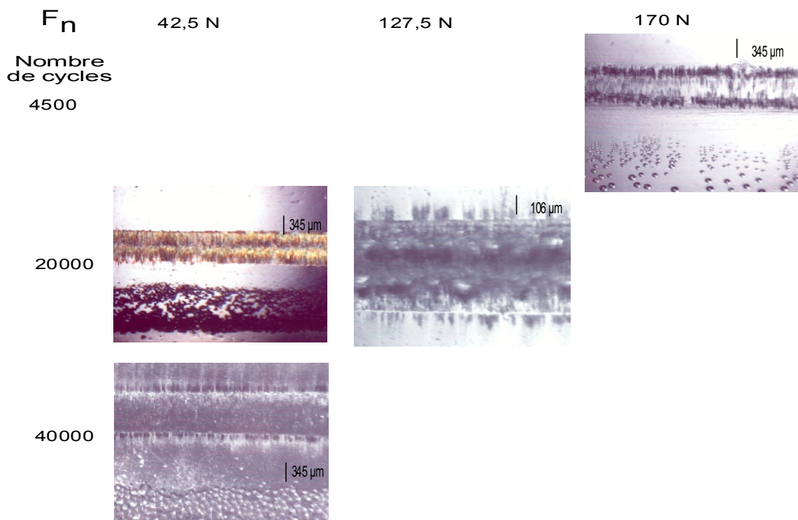
figure 107 : Images CCD de la zone de contact 316L/PMMA, F_n = 42,5\text{N} ; 127,5 \text{ N} et 170 N, nombre de cycles compris entre 4500 et 40000.
