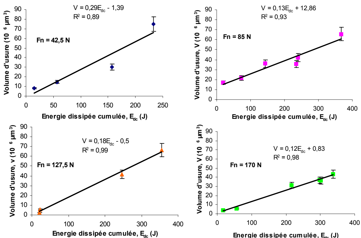
figure 57 : Variations du volume d'usure en fonction de l'énergie dissipée pour quatre forces normales différentes : 42,5 N ; 85 N ; 127,5 N ; 170 N ; f = 1 Hz ; d_{\text{réel}} = \pm 40 \mu\text{m} .
