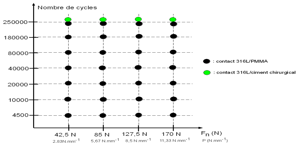
figure 87 : Matrice de tests pour l'étude du fretting en solution de Ringer, à potentiel libre, du contact 316L/PMMA et 316L/ciment chirurgical ; f = 1 Hz ; d_{réel} = \pm 40 \mu m .
