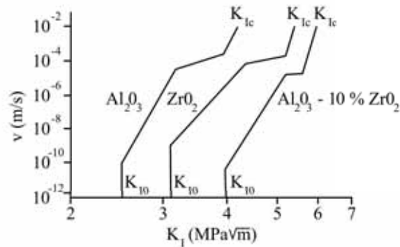
Figure I.21 : Comparaison des courbes v - K_I de l'alumine ( Al_2O_3 ), de la zirconne ( ZrO_2 ), et d'une céramique composite à matrice d'alumine renforcée par 10 %vol de zirconne ( Al_2O_3 - 10\% ZrO_2 ). Ces test ont été réalisés sous chargement statique et sous air (De Aza et al. 2002).
