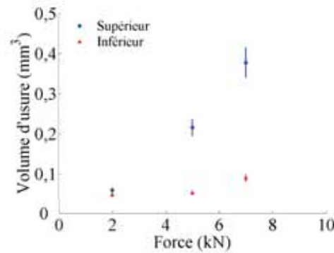
Figure III.20 : Volumes d'usure supérieur et inférieur de têtes en zircone, après 10^6 chocs, en fonction de la force appliquée. Les barres d'incertitude représentent \pm 10\% du volume calculé.
