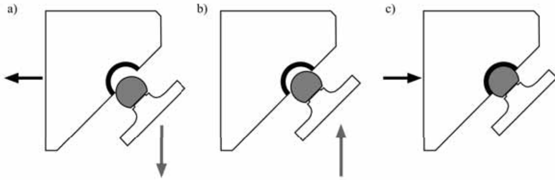
Figure II.14 : Vue en coupe du montage lors des essais avec décoaptation. a) Position initiale : la tête a été translattée verticalement vers le bas et le porte-cupule a donc été poussé horizontalement vers la gauche, à cause du contact entre la tête et la cupule. b) Phase de choc : la tête est translattée verticalement vers le haut en 11 ms et, du fait que le porte-cupule n'a pas le temps de se déplacer, le contact a lieu sur le bord de la cupule. c) Fin du cycle : le porte-cupule se translate horizontalement vers la droite grâce à l'effet de ressort du palier glissant, et un nouveau cycle peut commencer.
