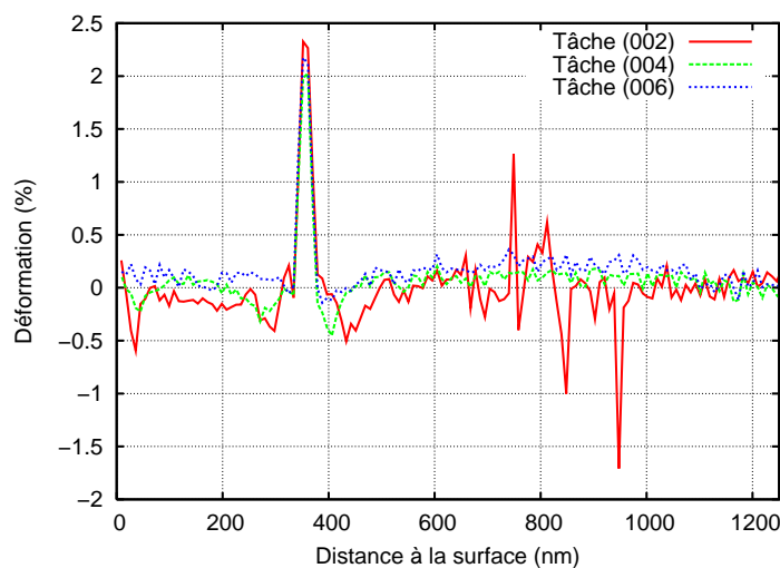
FIGURE V.10: Graphe des déformations dans la direction x d'une couche de \text{SiGe} enterrée en fonction de la tache de diffraction choisie.
