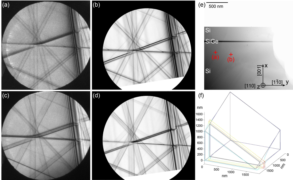
FIGURE IV.8: Comparaison entre clichés expérimentaux et simulés pour un échantillon composé d'une couche de Si_{0.69}Ge_{0.31} de 28,5 nm recouverte par 325 nm de silicium et préparé par clivage (axe [8,11,0] à 300 kV). Les phénomènes de relaxation en 3D sont bien reproduits par une modélisation de l'échantillon par éléments finis. (a) et (b) Images représentant les clichés expérimentaux et simulés pour une position de 540 nm sous la surface et une épaisseur de 730 nm. (c) et (d) Images représentant les clichés expérimentaux et simulés pour une position de 600 nm sous la surface et une épaisseur de 615 nm. (e) Cliché HAADF expérimental (contraste inversé) dans lequel les positions des clichés acquis sont reportées. Les variations d'épaisseur de la structure sont nettement visibles (variation du contraste dans l'image). (f) Structure éléments finis ayant servi à la modélisation des clichés CBED. Les phénomènes de relaxation (champ de déplacement amplifié 30 fois) sont visibles sur les bords libres de la lame.
