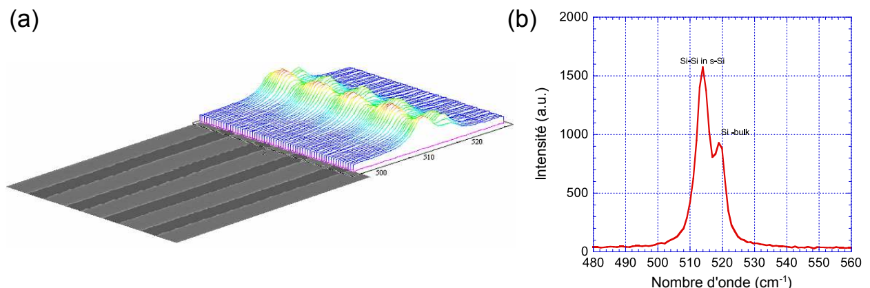
FIGURE I.2: Figures obtenues par Denis Rouchon. (a) Série de spectres Raman acquis sur des lignes de silicium contraintes ( sSi ) déposées sur un substrat SOI. (b) Détail d'un spectre sur une ligne : deux pics sont clairement visibles, l'un correspondant au silicium relaxé du substrat, l'autre au silicium contraint. La distance entre les deux pics est liée à la déformation dans le matériau.
