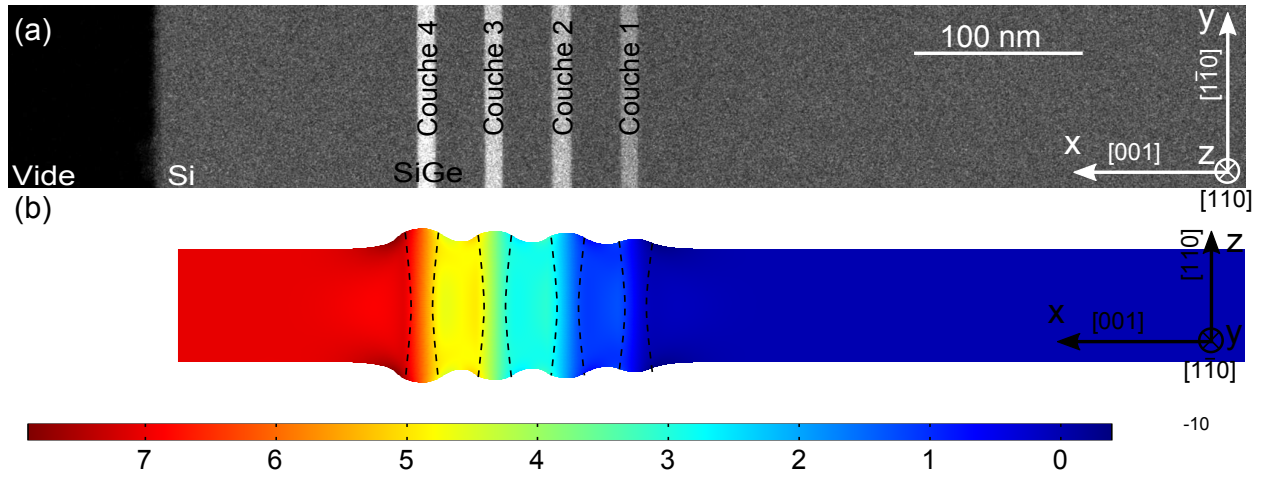
FIGURE V.14: (a) Image STEM HAADF de l'échantillon multicouches SiGe. Les différentes couches sont numérotées de 1 à 4, de la moins concentrée à la plus concentrée en germanium. (b) Champ de déplacement dans la direction x de la lame mince modélisée par éléments finis en prenant en compte les effets de relaxation de lame mince (déplacements amplifiés d'un facteur 50).
