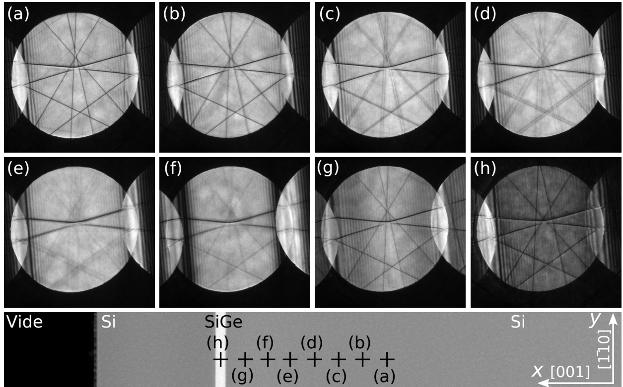
FIGURE IV.2: Evolution d'une série de clichés CBED dans un échantillon composé d'une couche de \text{Si}_{0.69}\text{Ge}_{0.31} enterrée dans une matrice de silicium (image STEM HAADF). L'élargissement des lignes de HOLZ est parfaitement visible sur les images (c), (d) et (e). Le contraste de certaines lignes de HOLZ disparaît alors presque totalement avant qu'une nouvelle série de lignes fines ne se forme : (f) et (g). La position des lignes de HOLZ est sensible à la composition et au paramètre de maille du matériau, comme on peut le constater en faisant la comparaison entre l'image (a) prise dans le silicium et l'image (h) prise dans la couche de SiGe. L'ensemble des clichés a été réalisé en axe [8,11,0] à 300 kV sur un échantillon d'épaisseur 410 \pm 10 nm.
