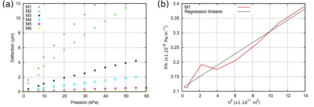
FIGURE IV.19: (a) Graphes de la déflexion en fonction de la pression pour chaque membrane étudiée. (b) Courbe \frac{P}{h} = f(h^2) et sa régression linéaire pour la membrane M1.
