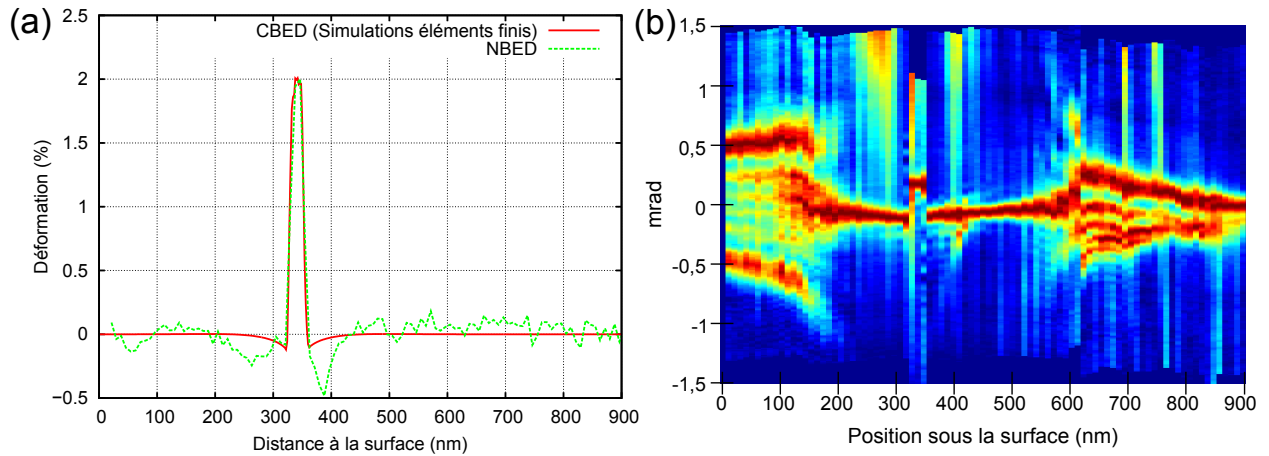
FIGURE VI.13: (a) Comparaison des profils de déformation dans la direction x perpendiculaire à la couche de SiGe entre les mesures par CBED (profils issus de simulation par éléments finis) et par nano-diffraction. (b) Carte de splitting expérimentale de la ligne (6,-4,10) associée à la couche de SiGe. Les clichés CBED nécessaires à l'obtention de cette carte ont été acquis à 300 kV en axe [8,11,0] .
