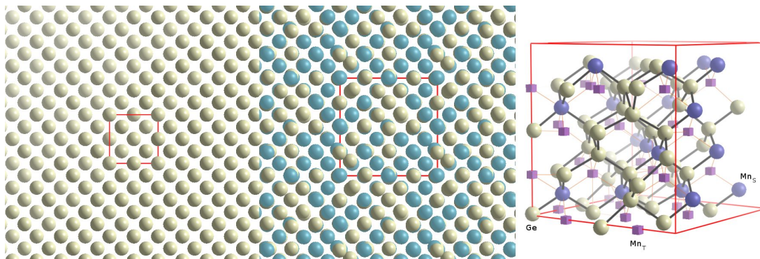
FIG. V.17 – A gauche, comparaison des mailles du germanium pur et nTmS selon la direction [001] . A droite, une image en perspective de la boîte utilisée dans la simulation du XAS du nTmS. Les cubes représentent les interstitiels tétraédriques.
