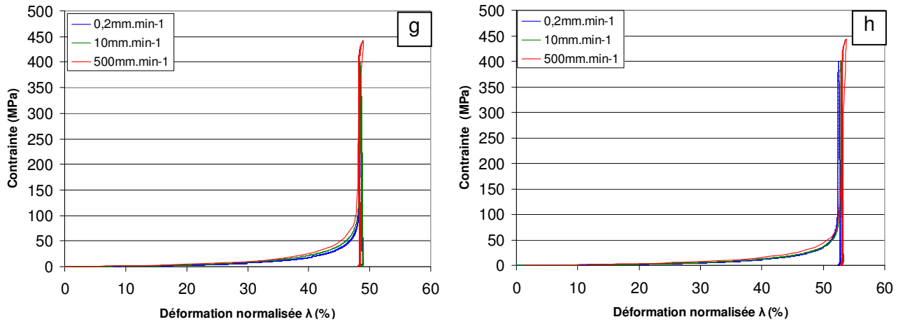
Figure 131 : Courbe de contrainte en fonction du déplacement normalisé de l'alumine SM8 (a), du PVA (b), du PS13 (c), du MHPC (d), du PEG1500 (e), du PEG4000 (f), du PEG6000 (g) et du PEG10000 (h).
