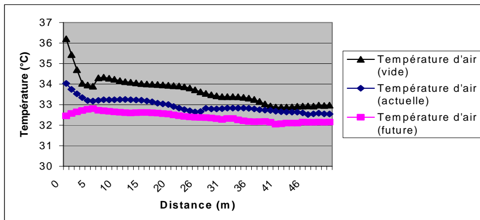
Figure 148 : Température d'air à 1 mètre du sol au milieu de la place du Millénaire
