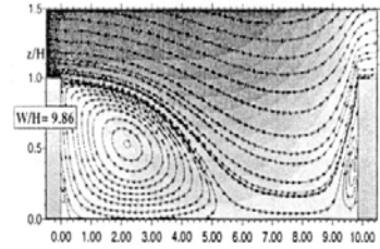
Figure 77 : Ecoulements aérauliques obtenus avec le code CHENSI [Sini et al. 1996]
