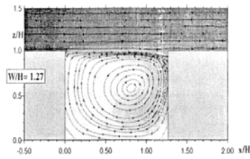
Figure 77 : Ecoulements aérauliques obtenus avec le code CHENSI [Sini et al. 1996]
