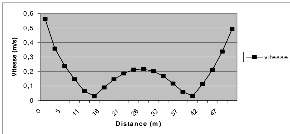
Figure 131 : Vitesse du vent au milieu de la place du Millénaire (vent de nord-ouest)
