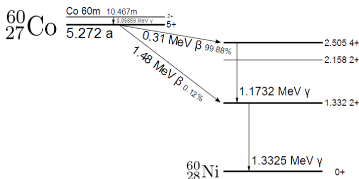
Figure III-29 : Schéma de désintégration du cobalt 60 [NUT]
