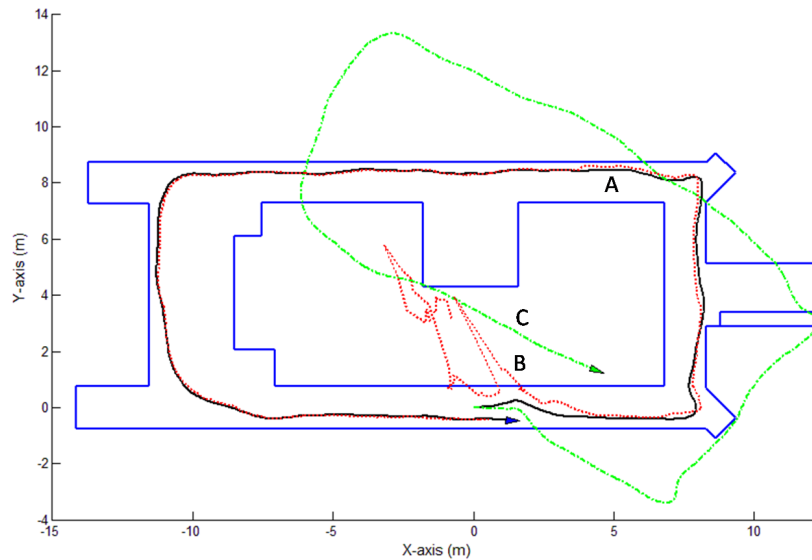
Figure C.3: La localisation globale utilisant MCL dans un couloir quasi-symétrique.
