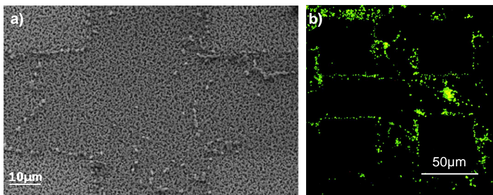
Figure 5.19. Image MEB 15 (a) et en fluorescence (b) des spores Bacillus Cereus après incubation avec les surfaces de nanofils de silicium renfermant des zones superhydrophiles de 50 μm 2 entourées de zones superhydrophobes.
