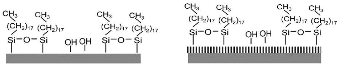
Figure 5.16. Schéma d'une surface plane de silicium avec des régions hydrophiles (terminaison OH) et des régions hydrophobes (terminaison \text{Si}-(\text{CH}_2)_{17}-\text{CH}_3 ) à gauche, et d'une surface de nanofils de silicium avec des régions superhydrophiles (terminaison OH) et des régions superhydrophobes (terminaison \text{Si}-(\text{CH}_2)_{17}-\text{CH}_3 ) à droite.
