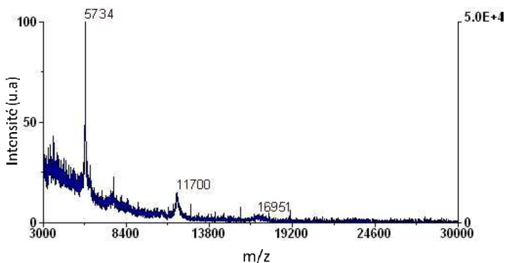
Figure 3.4. Spectre d'analyse du mélange de l'insuline bovine (5734 Da), la thioredoxine (protéine de Escherichia coli , 11700 Da), et l'apomyoglobine (16952 Da) par LDI-MS sur nanofils de silicium silanisés par OTS puis exposés à l'UV/ozone.
