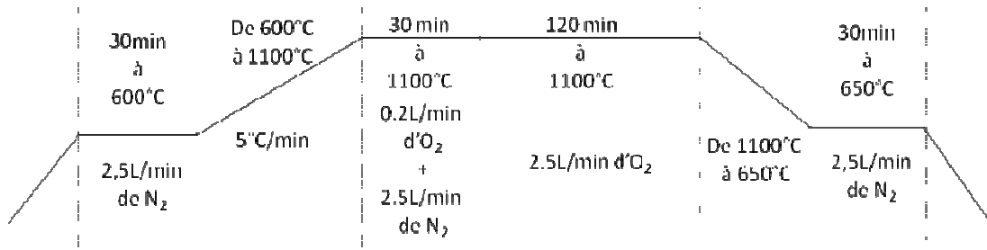
Figure 3.11. Procédé d'oxydation thermique exposant les différentes étapes de montées en température, de paliers et de recuits successifs.
