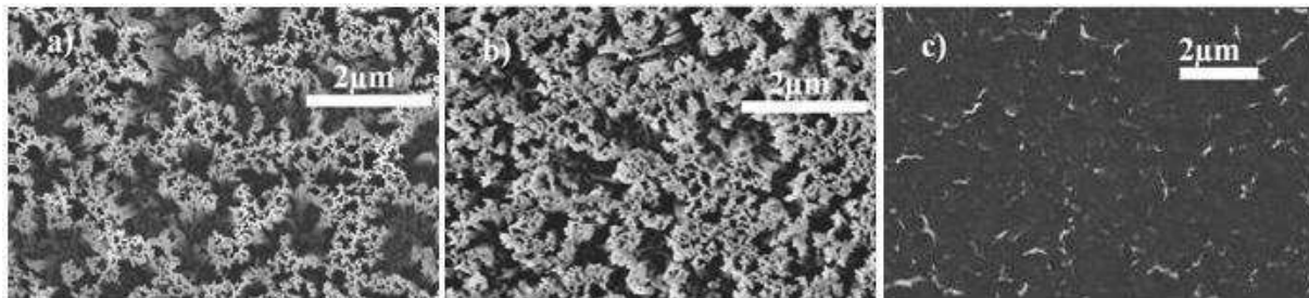
Figure 3.12. Image MEB du support de nanofils de silicium optimisé pour les analyses LDI-MS avant oxydation a), après oxydation oxydation thermique complète des nanofils de silicium b), et après oxydation et attaque HF c).
