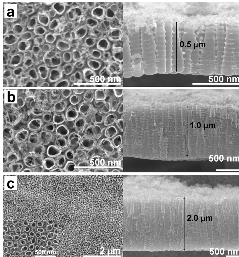
Figure 3.21. Images MEB des différents supports de nanotubes de TiO 2 testés pour les analyses LDI-MS.
