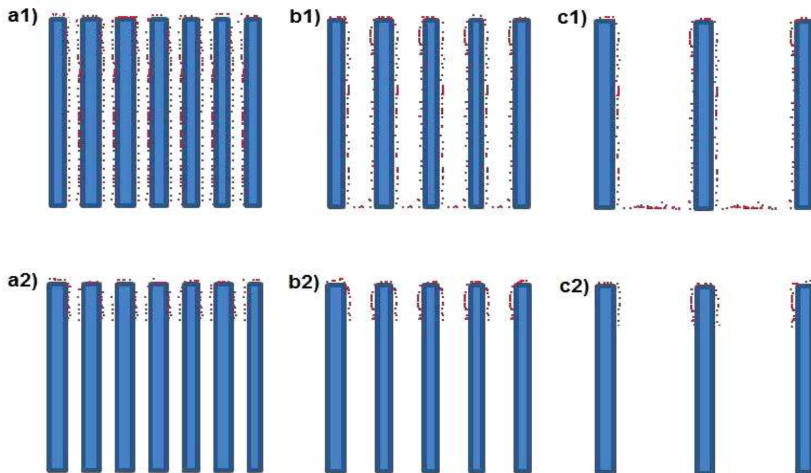
Figure 3.13. Schéma de différentes densités de nanofils de silicium (a, espacement des fils de 10 à 30 nm ; b, espacement des fils de 30 à 50 nm ; c, espacement des fils de 50 nm à 2 \mu\text{m} ) et de l'infiltration des peptides selon que les nanofils sont modifiés avec un silane hydrophobe (2) ou non (1).
