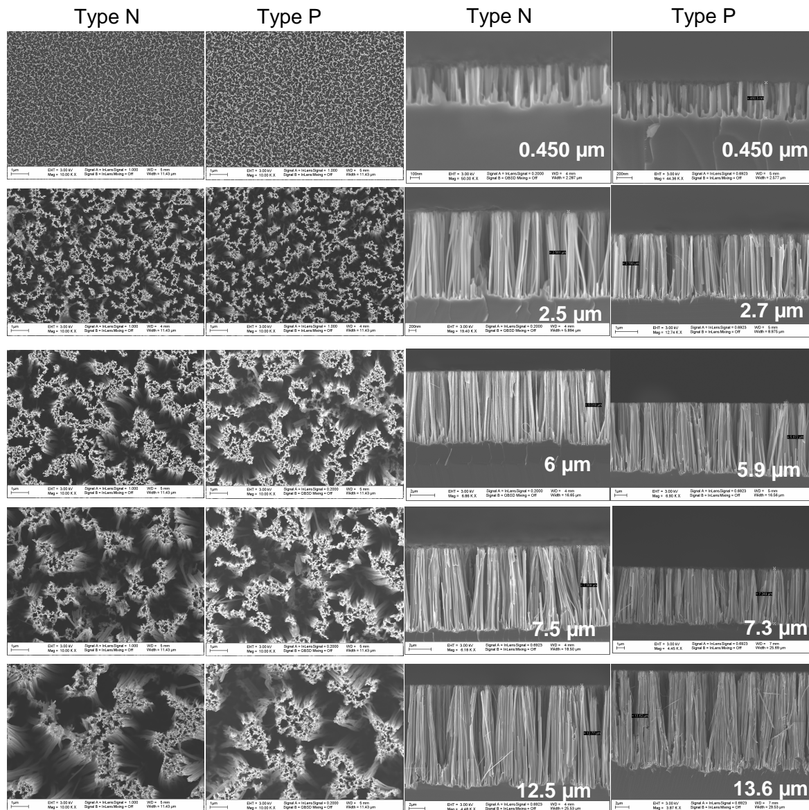
Figure 2.7. Images MEB : Vues de dessus (grossissement 10KX) et en coupe des nanofils de silicium synthésés par voie chimique en fonction du temps de la réaction (de haut en bas : 5, 10, 30, 60 et 120 minutes) et du type de dopage (N ou P, resistivité 1-10 Ω.CM) du substrat de silicium attaqué (orientation <100>).
