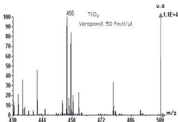
Figure 3.25. Spectres de masse obtenus en LDI-MS sur nanotubes de TiO 2 pour la détection du Verapamil (m/z = 455) à 50 fmol/μl.
