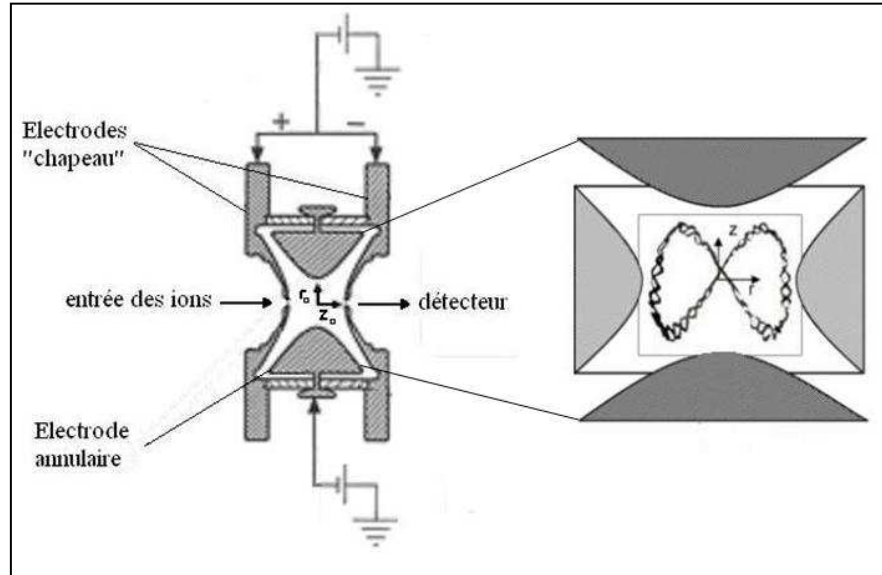
Figure 1.11. Schéma d'une trappe ionique
