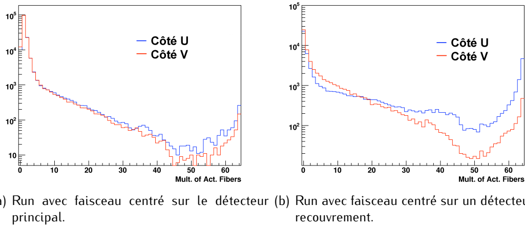
FIGURE 6.14: Distribution de la multiplicité moyenne des plans U et V pour configurations de runs différentes.
