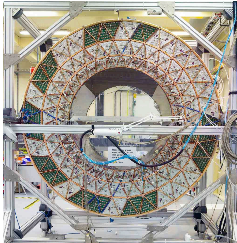
FIGURE 1.8: Le détecteur à transition de radiation.
