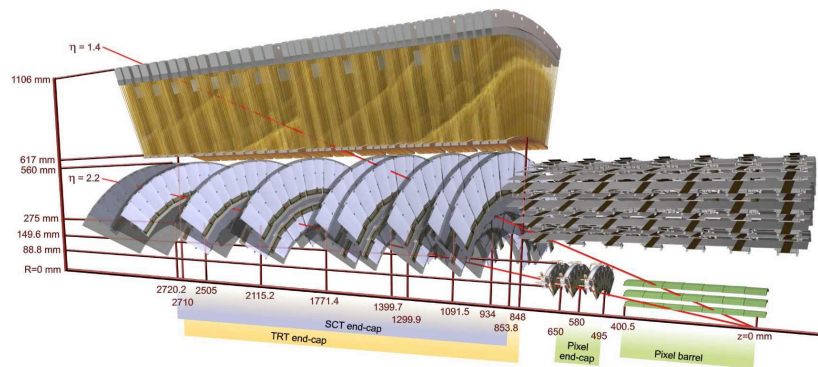
(c) Vue en coupe de la partie end-cap du détecteur interne.
