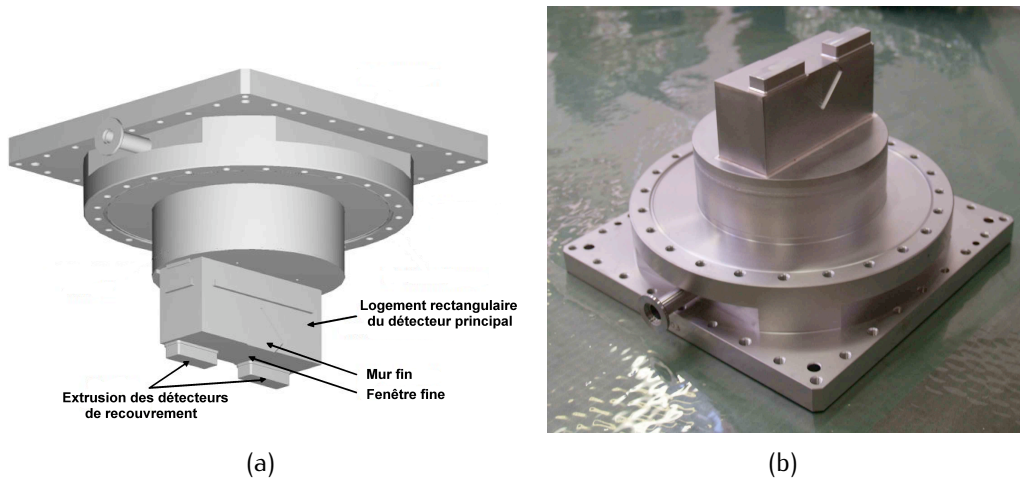
FIGURE 4.4: Schéma et réalisation d'un pot romain. La fenêtre inférieure est amincie pour diminuer l'approche au faisceau. Le mur faisant face à la partie active du détecteur principal l'est aussi afin de limiter la quantité de matière en amont du détecteur. Les deux extrusions permettent de loger les détecteurs de recouvrement.
