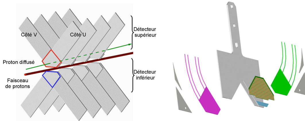
(a) Représentation de la géométrie UV. Les sur- faces actives des détecteurs haut et bas per- mettant de reconstruire la position (x,y) sont soulignées en rouge et bleu. (b) Vue explosée d'un plan UV. Les fibres sont collées sur un support en titane et sur un substrat de G10 pour la partie active.
