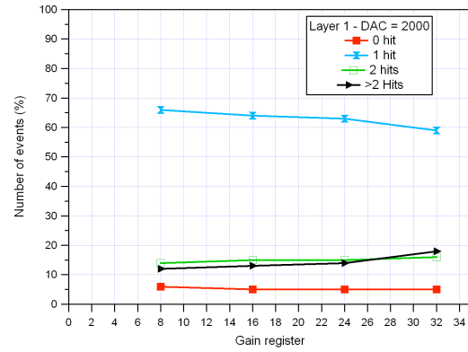
(b) Balayage du gain MAROC2 avec HV=950 V et DAC=2000.
