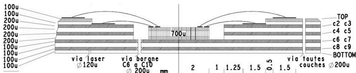
FIGURE 4.19: Vue en coupe de la carte active. Les couches supérieures sont évidées pour permettre l'insertion de la puce MAROC. Le bonding s'effectue à partir des deux couches supérieures. Le FPGA situé sur la face arrière n'est pas représenté sur la figure.
