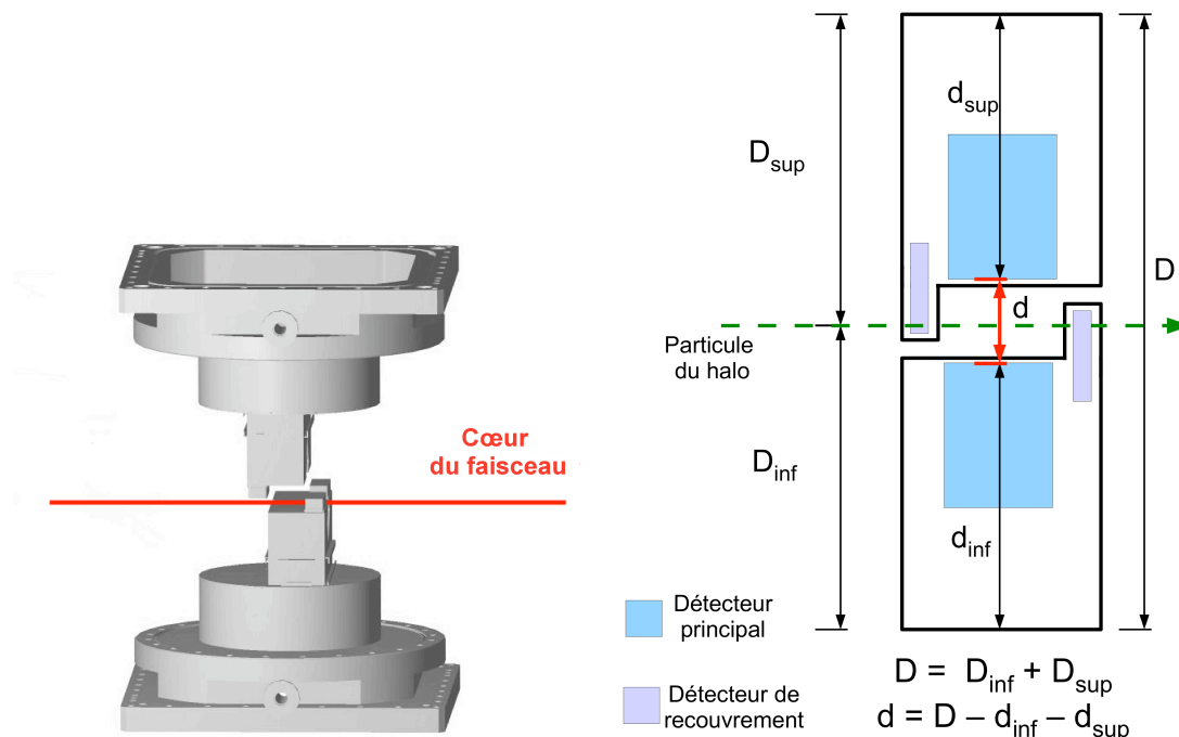
(a) Vue tridimensionnelle de deux pots pour illustrer le concept des détecteurs de recouvrement. La partie principale du faisceau passe entre les détecteurs de recouvrement qui n'interceptent que la partie externe du halo du faisceau. (b) La distance verticale entre les détecteurs est la distance d du schéma ci-dessus.
