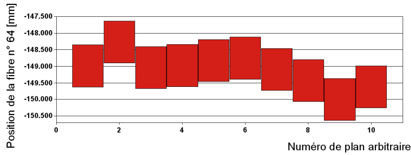
FIGURE 6.30: Position de la dernière fibre des plans du côté U pour le pro type testé en faisceau. On constate qu'à mesure que l'on ajoute des fibres on s'éloigne du décalage initial que l'on peut observer sur la figure 6.27(b).
