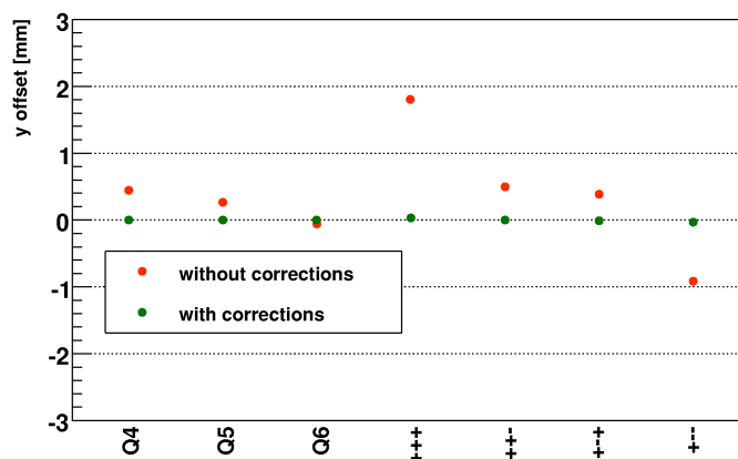
FIGURE 3.37: Déplacement vertical de la position des protons dans les pots romains avant et après correction de l'orbite fermée.
