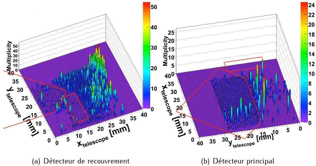
FIGURE 6.18: Multiplicités moyennées sur tous les plans observés dans le détecteur ALFA en fonction de la position du point d'impact des particules. A nouveau les traits rouges soulignent la forme des scintillateurs de déclenchement du détecteur ALFA. On retrouve sur la figure de gauche la forme de la bride qui relie le support au tube à vide de l'accélérateur.
