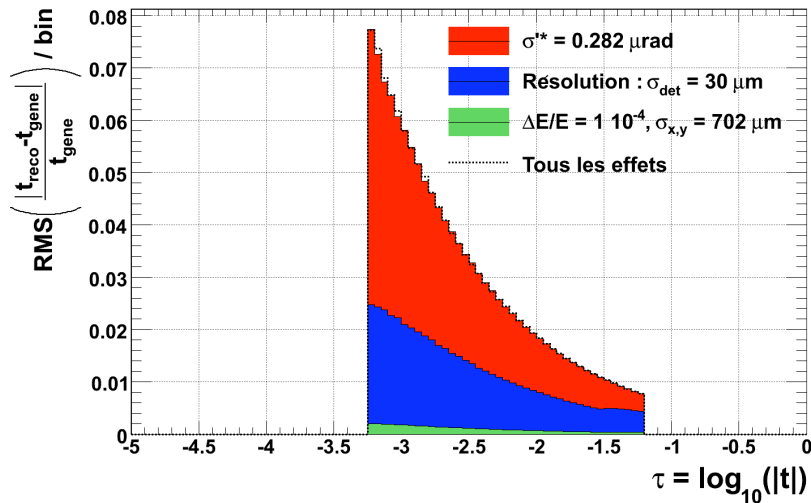
FIGURE 3.29: Impact sur la valeur de t reconstruite des paramètres du faisceau.
