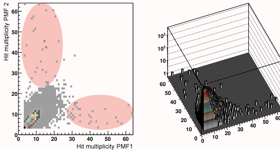
FIGURE 6.3: Multiplicité de la PMF1 en fonction de la PMF2. Les événements dans les ellipses rouges montrent que les larges multiplicités ne sont pas observées pour tous les plans en même temps.
