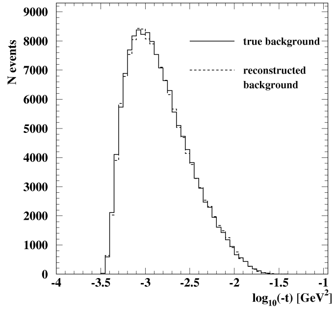
FIGURE 2.15: Comparaison entre le spectre du bruit de fond généré et le spectre obtenu en calculant la contribution du bruit de fond symétrique par symétrie miroir. Figure extraite de [46]
