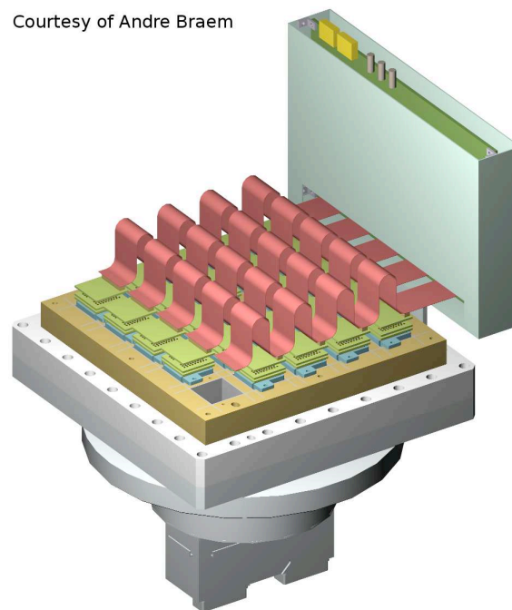
FIGURE 4.13: Vue de dessus d'un pot romain. Les rangées de PMFs sont reliées via les câbles kaptons souples à la carte mère ici insérée dans un cache de protection.
