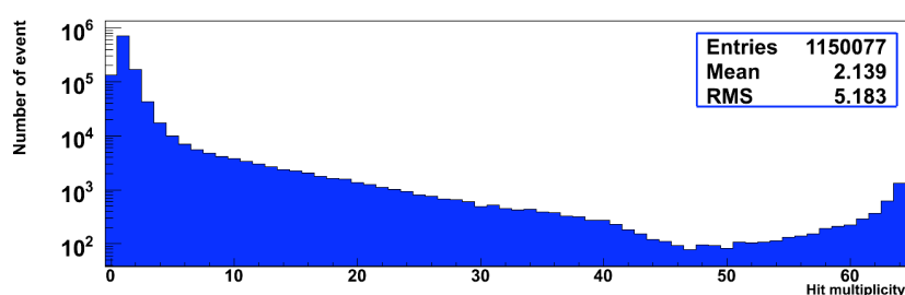
FIGURE 6.9: Distribution de la multiplicité moyennée sur l'ensemble des plans pour HV=900 V, DAC=2000 et tous les gains de la puce MAROC2 à 16.
