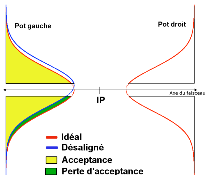
FIGURE 3.35: Illustration de la baisse de l'acceptance due au déplacement du faisceau. La convolution des distributions enregistrées dans les pots gauches et droites ne peut que réduire l'acceptance globale.
