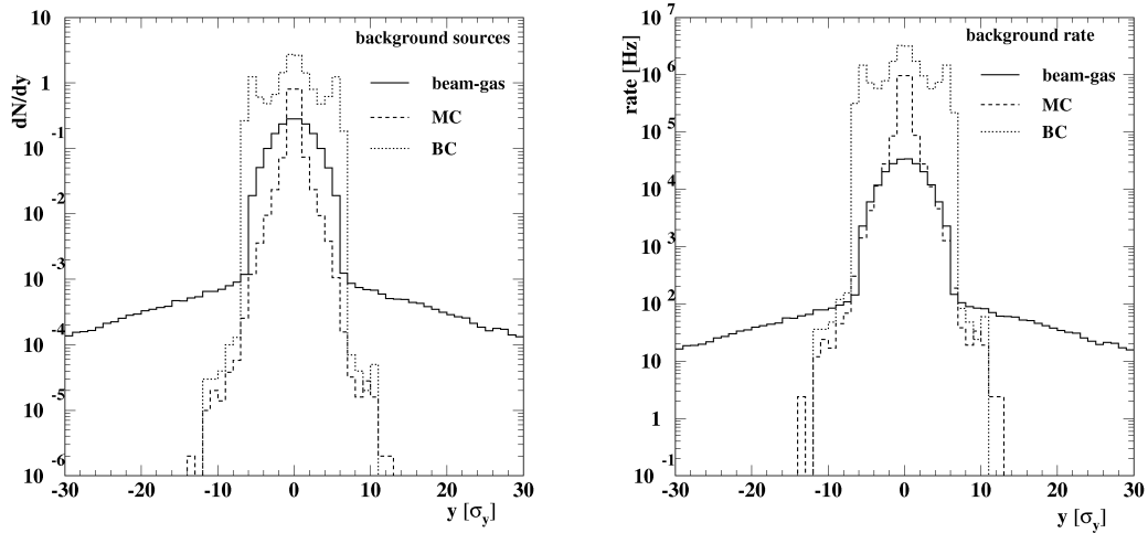
(a) Distribution des positions verticales des différents événements de bruit de fond machine. (b) Taux des différents événements non simultanés de bruit fond machine.
