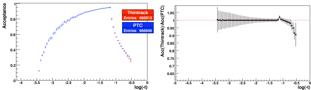
(a) Acceptances calculées avec ThinTrack (rouge) et MadXP (bleu). (b) Rapport entre l'acceptance obtenue avec ThinTrack et celle obtenue avec MadXP .
