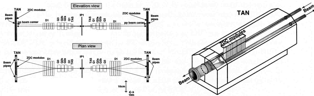
FIGURE 1.25: Vue de la ligne de faisceau couvrant \pm 140 m autour du point d'interaction (à gauche). Les modules du ZDC sont situés dans le TAN dont une vue est présentée sur la figure de droite.
