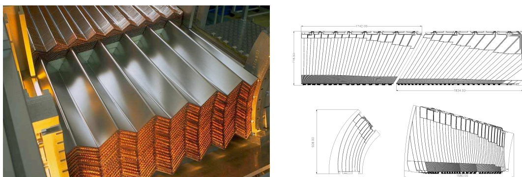
(a) Géométrie en accordéon de la partie barrel (b) Les quatre types d'électrodes du calorimètre électromagnétique avant pliage. Les deux électrodes du hauts appartiennent au barrel et celle du bas aux end-cap électromagnétique.
