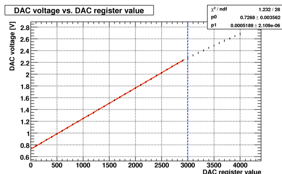
FIGURE 5.47: Lissage de la valeur de V_{DAC} en fonction de la valeur de registre du DAC.
