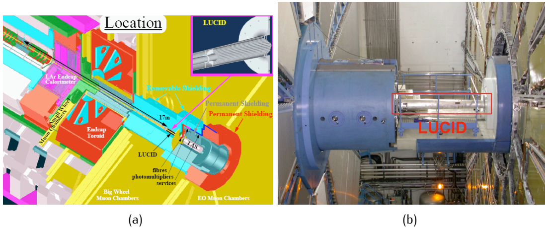
FIGURE 1.27: Le détecteur LUCID est inséré entre les deux grandes roues des chambres à Muons dans les parties avant et arrière du détecteur ATLAS à \pm 17 m du point d'interaction.
