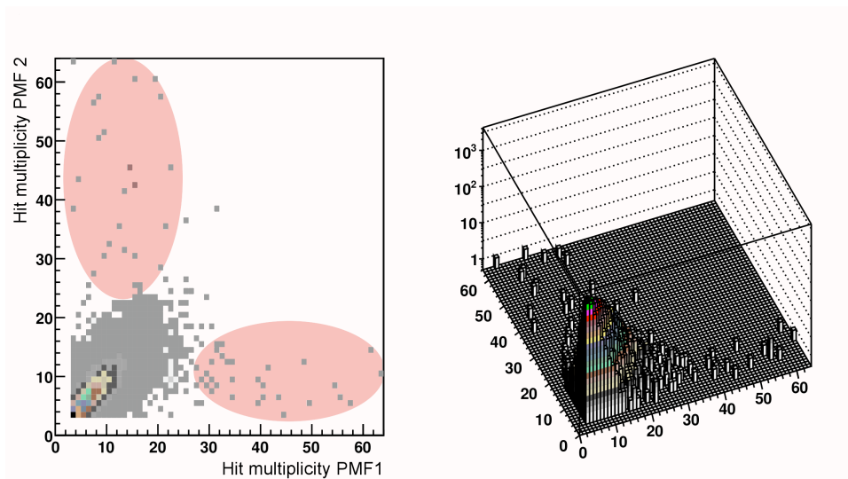
FIGURE 6.3: Multiplicité de la PMF1 en fonction de la PMF2. Les événements dans les ellipses rouges montrent que les grandes multiplicités ne sont pas observées pour tous les plans en même temps.
