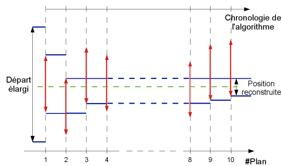
FIGURE 6.22: Méthode utilisée pour la reconstruction des événements. Les traits horizontaux bleus représentent la surface de recouvrement des fibres qui diminue suivant l'information apportée par chaque nouveau plan. La position reconstruite est le centre de la surface de recouvrement lorsque les dix plans de fibres ont été utilisés.
