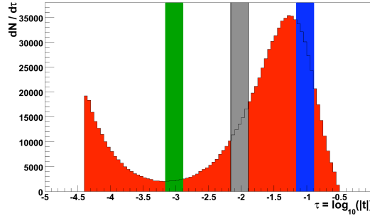
FIGURE 3.5: Spectre généré au point d'interaction. Les bandes de couleurs représentent les intervalles en t visibles sur la figure 3.6. Les paramètres de génération sont : \sigma_{tot} = 100 mb, b = 18 \text{ GeV}^{-2} et \rho = 0.13 .
