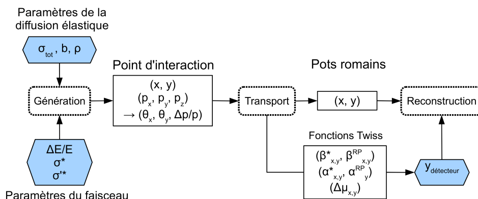
FIGURE 3.1: Schéma de la simulation complète d'un événement de diffusion élastique.
