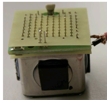
FIGURE 4.15: Vue de la carte haute tension seule et une fois montée sur le MAPMT. Des plaquettes isolantes sont introduites entre le MAPMT et la carte haute tension et entre cette dernière et la carte passive.
