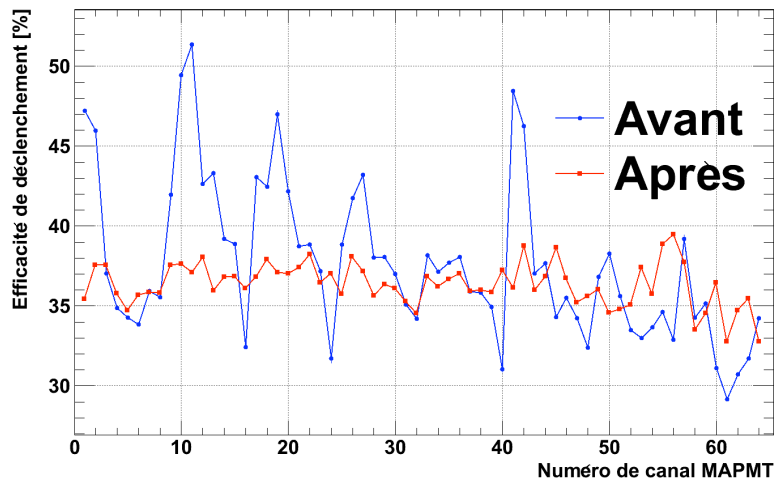
FIGURE 5.29: Efficacité de déclenchement pour les 64 canaux du MAPMT avant et après égalisation des gains avec DAC=1100, HV=950 V et V_{Diode}=1.98 V.
