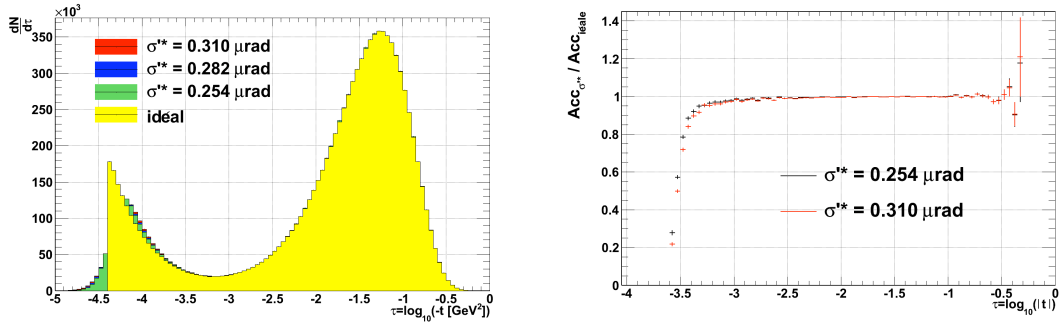
(a) Spectres générés pour différentes valeurs de (b) Rapport des acceptances avec divergence angulaire sur l'acceptance nominale.
