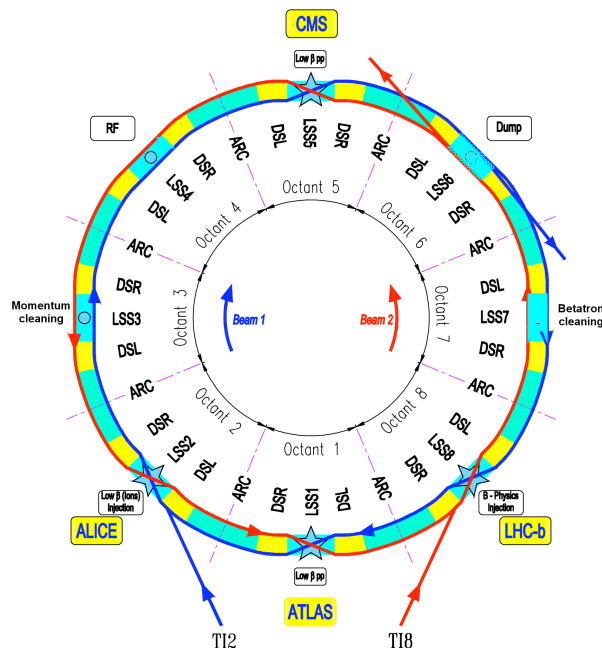
FIGURE 1.2: Schéma du LHC. Le faisceau 1 circule dans le sens horaire et le faisceau 2 dans le sens trigonométrique.
