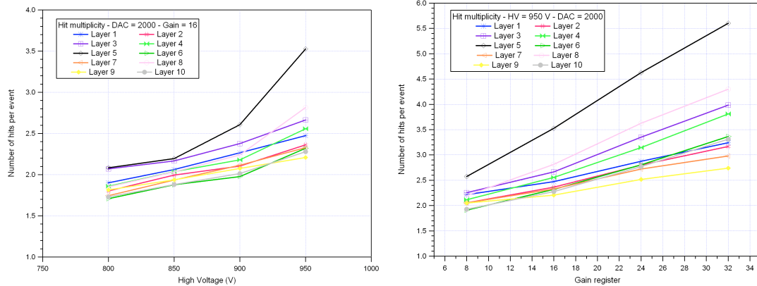
(a) Balayage de la haute tension avec tous les gains MAROC2 à 16 et DAC=2000. (b) Balayage du gain MAROC2 avec HV=950 V et DAC=2000.
