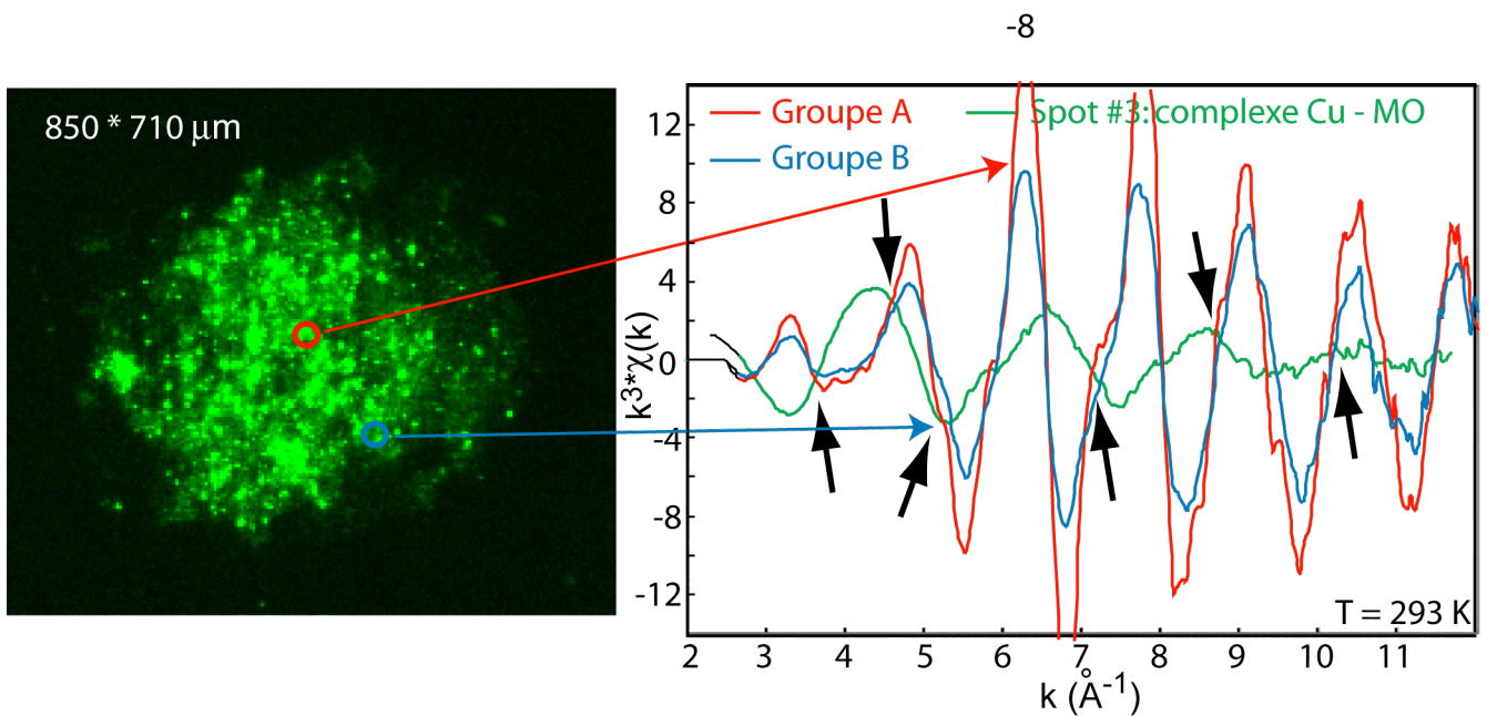
FIGURE 10.10 Comparaison entre un spectre de groupe A, un spectre du groupe B et le spectre du spot #3 correspondant au complexe Cu - MO. L'existence de points isobestiques indique que le groupe B est combinaison linéaire du groupe A et du complexe Cu -MO.
