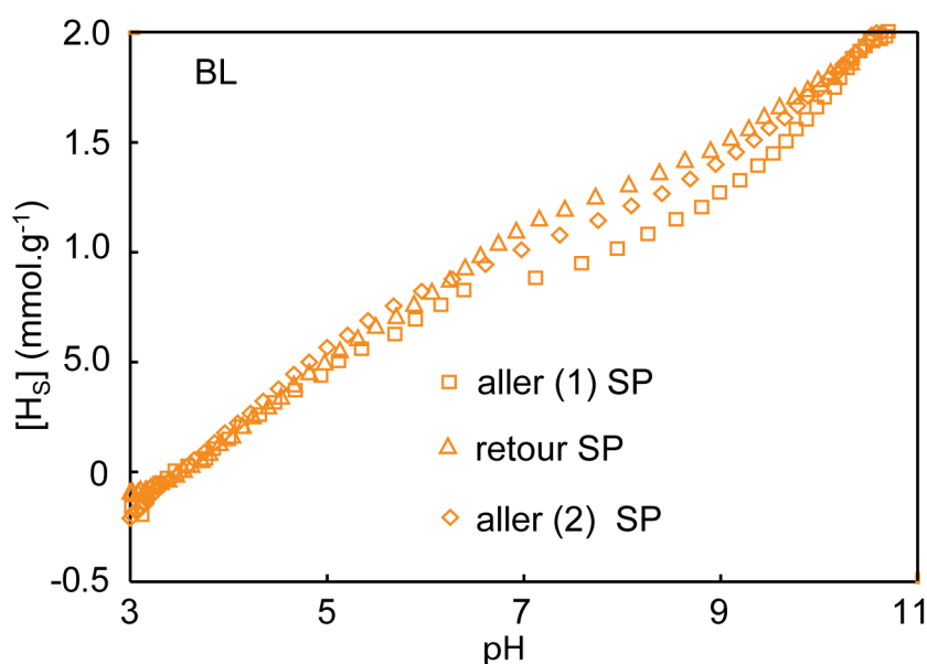
FIGURE 5.11 Concentration des protons relâchés [\text{H}_s] de la tourbe blonde (SP) pour un titrage aller (1), retour et aller (2) en fonction du pH.
