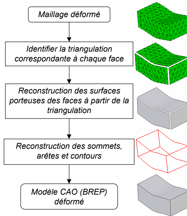
FIG. 3.3 – Algorithme de reconstruction
