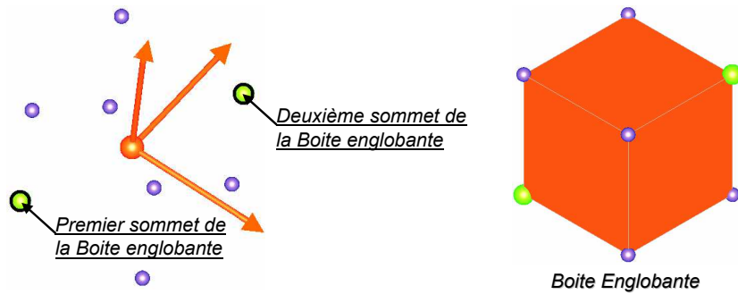
FIG. 3.51 – Les deux sommets de la boîte englobante suivant la grande diagonale
