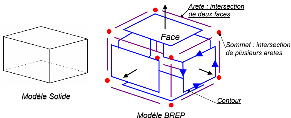
FIG. 1.3 – Modèle BREP
