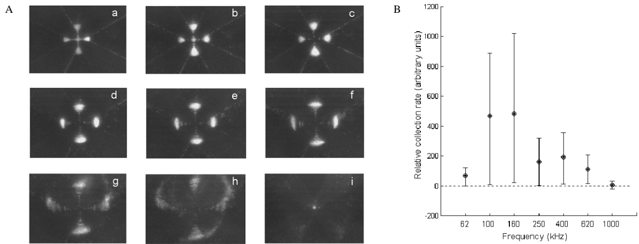
Figure I.31 : (A) Séquences d'images montrant le comportement de particules de latex à différentes fréquences (de 1MHz pour la 1 ère photographie à 2MHz pour la dernière avec un pas de 125 kHz) (B) Tracé du taux de collecte en fonction de la fréquence, les barres indiquent l'écart-type mesuré pendant les dix 1 ères secondes [94]
