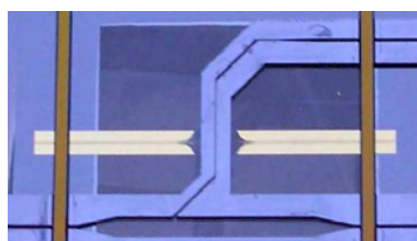
Figure I.33 : Prototypé de microcapteur combinant une partie microfluidique et une partie hyperfréquence [100]
