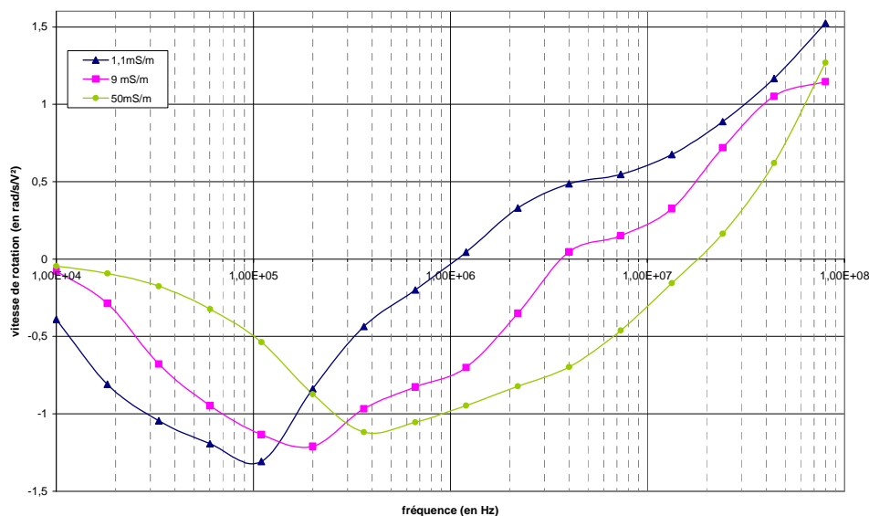
Figure IV.82 : Spectres d'électrorotation de levures dans des milieux présentant différentes conductivités
