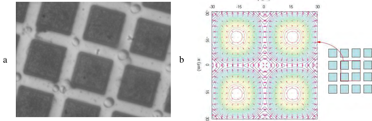
Figure I.17 : Micro positionnement sans contact de levures (a) matrice de micro aimants parallélépipédiques de CoPt (25 μm de côté et 10μm de gap) (b) cartographie des isovalues de l'énergie magnétique [55]
