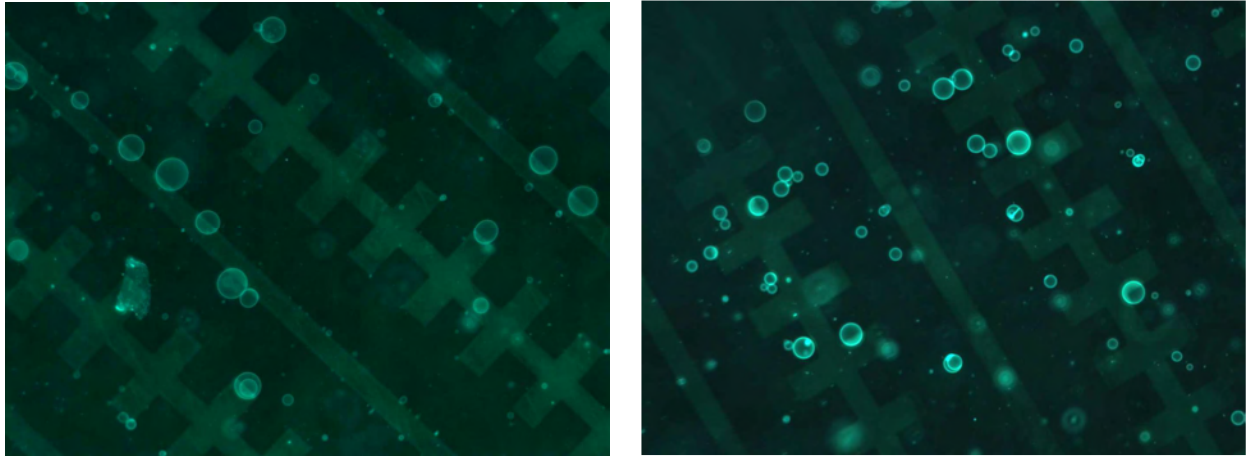
Figure IV.94 : à gauche, les liposomes électroformés sont soumis à la diélectrophorèse positive ; à droite, ils sont soumis à la diélectrophorèse négative
