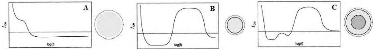
Figure I.40 : Différents types de réponse de la partie réelle du facteur de Clausius-Mossotti (A) sphère homogène (B) sphère monocouche (C) sphère à trois couches [41]
