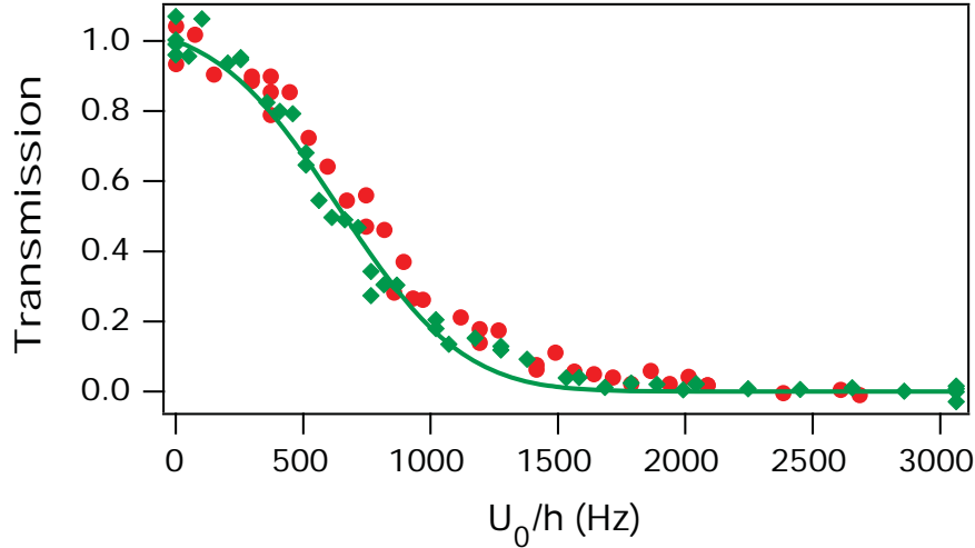
FIG. 3.21: Courbes de transmission du laser à atomes à travers la barrière fine de waist w_z = 1.36\mu\text{m} (point rouge) et la barrière épaisse de waist w_z = 3.8\mu\text{m} (losange vert) en fonction de l'amplitude U_0 des barrières. Le fait que les deux courbes se superposent prouve que l'effet tunnel est ici négligeable.
