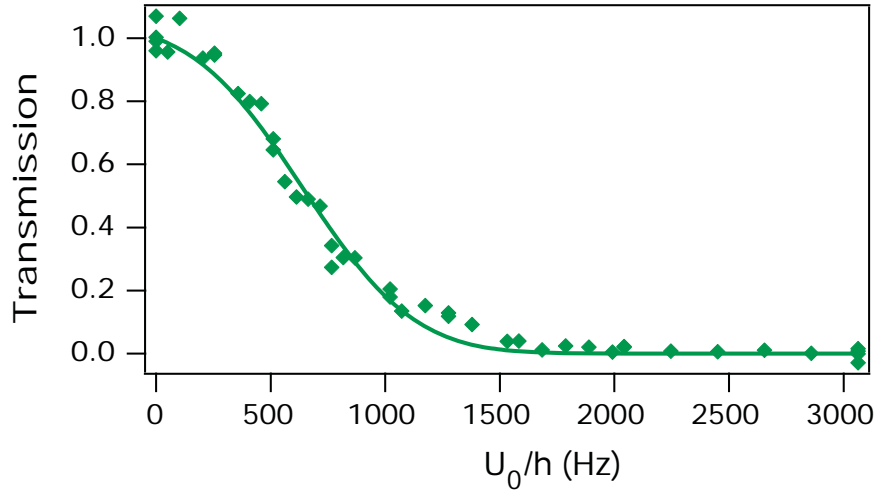
FIG. 3.20: Courbe de transmission du laser à atomes à travers la barrière épaisse de waist 3.8 \mu\text{m} suivant z et d'amplitude U_0 variable. Le laser à atomes se propage avec une longueur d'onde de Broglie constante autour de 1.5 \mu\text{m} , soit plus faible que l'épaisseur de la barrière. L'ajustement des points expérimentaux par l'équation (3.49) (trait plein) donne une énergie moyenne E_{\text{laser}} = 640 \pm 40 Hz et une largeur en énergie \sigma = 380 \pm 60 Hz pour le laser à atomes.
