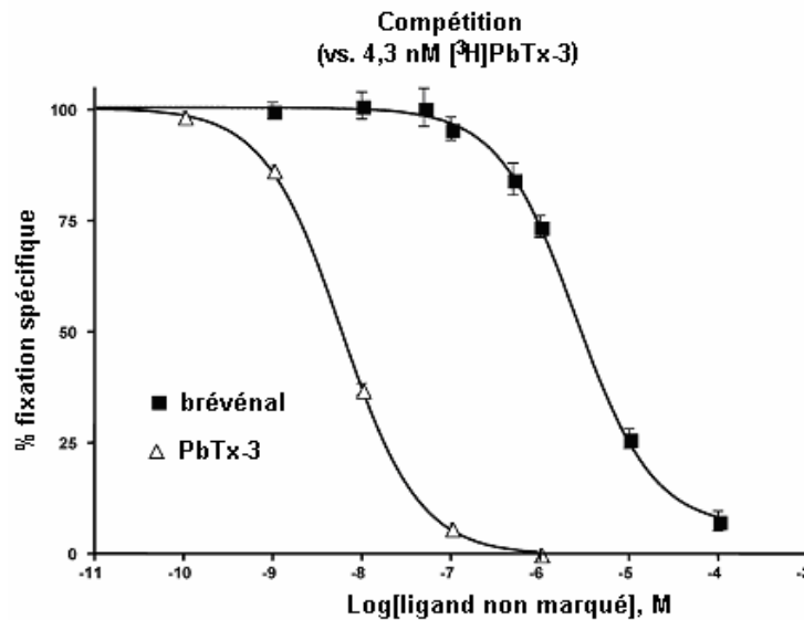
Figure I.3.2.3.a : Déplacement de la PbTx-3 tritiée ( ^3\text{H} ]PbTx-3) de synaptosomes de cerveau de rat par le brevénal
