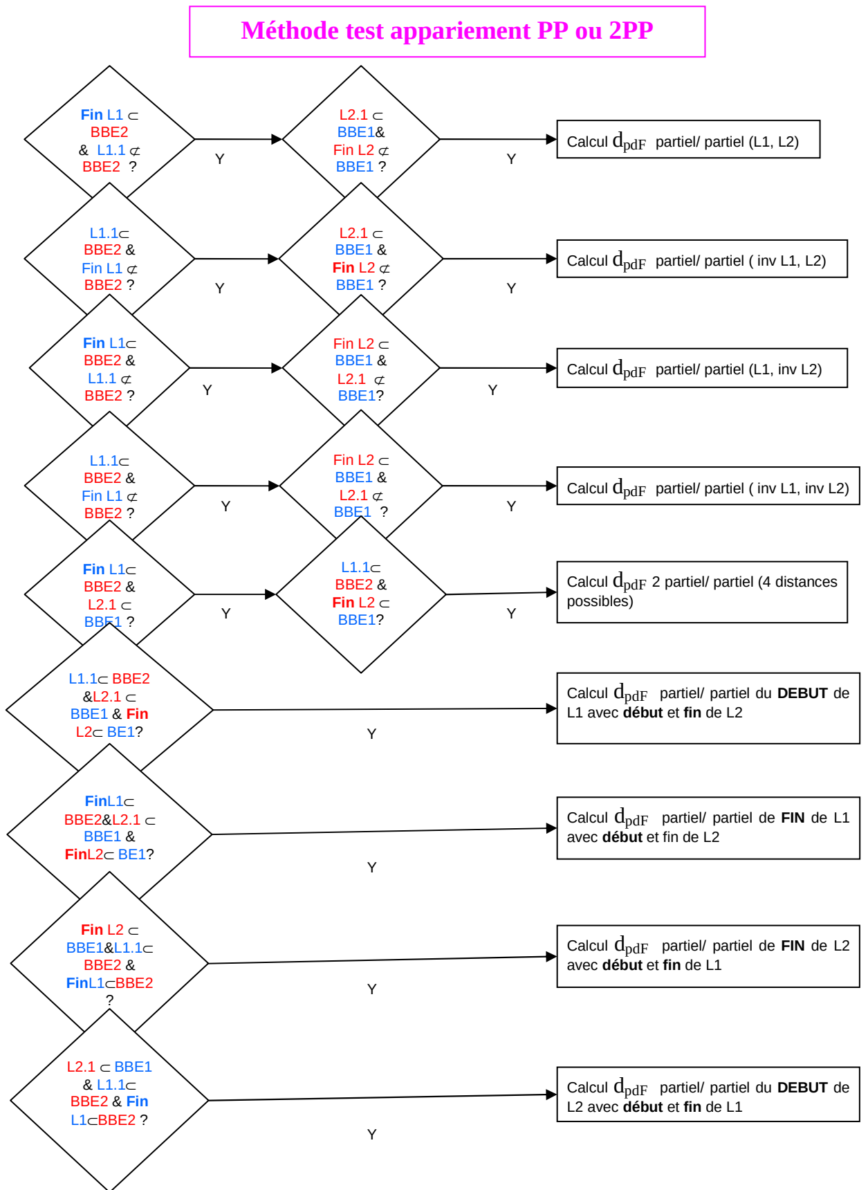
Figure 54 : Algorithme de test d'appariement partiel/partiel (PP) et deux partiel/partiel (2PP).
