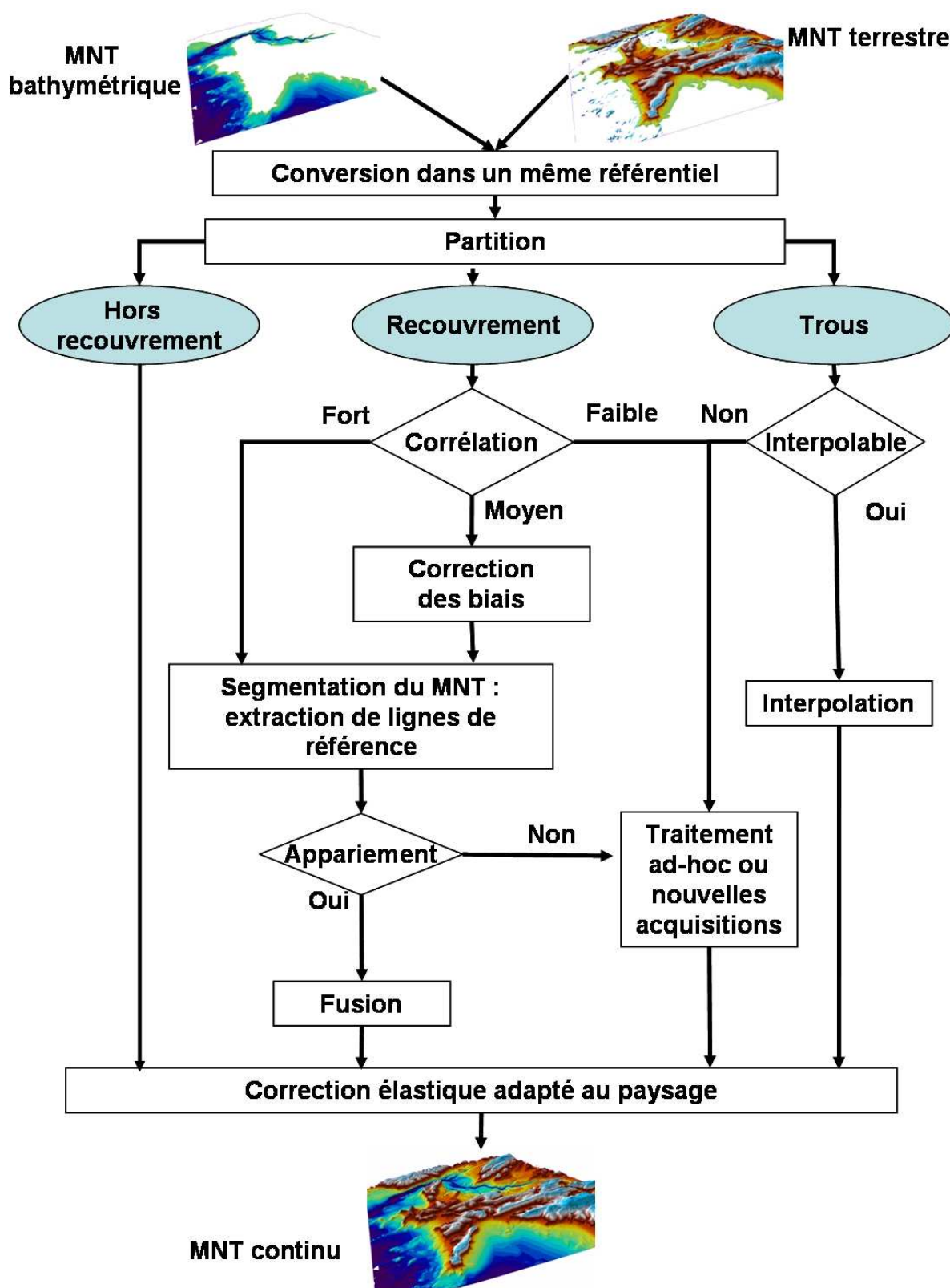
Figure 79 : Représentation de l'ensemble de la méthodologie d'intégration.
