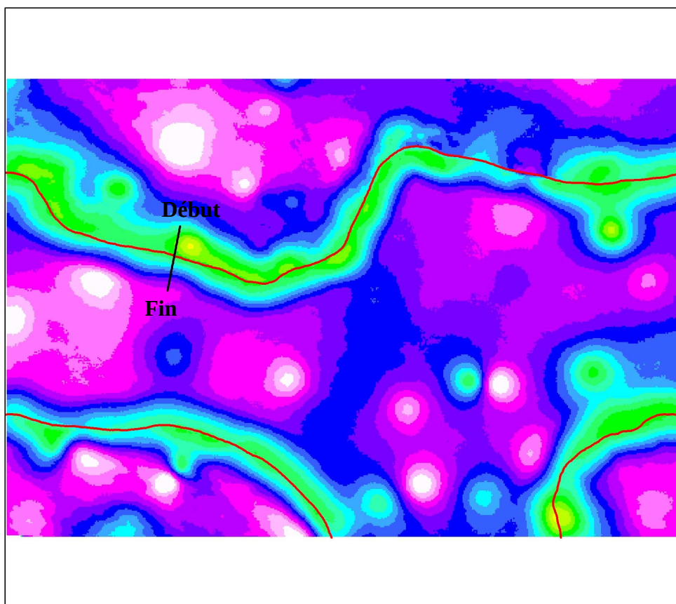
Figure 114 : Localisation du trait de coupe. La carte de soustraction entre le MNT de référence et le MNT DEL32 montre l'emplacement du trait vis-à-vis de la bande de déformation.
