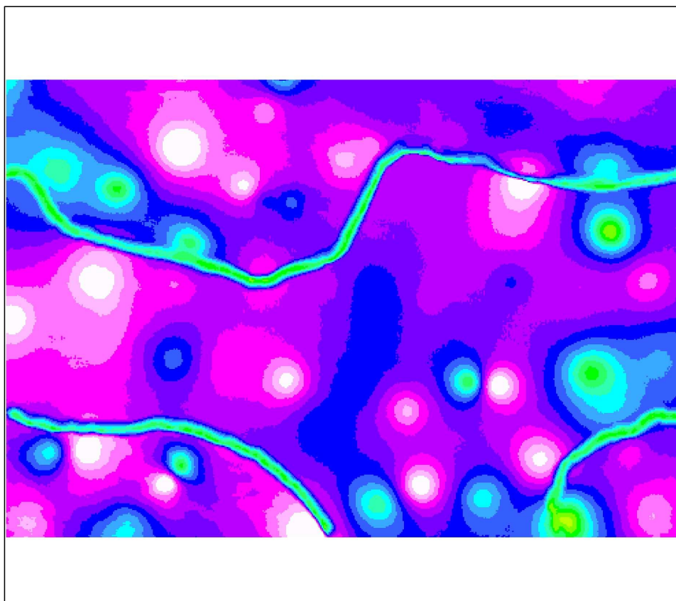
Figure 110 : Soustraction du modèle de référence avec le modèle topographique déformé élastiquement ( R=8 ).
