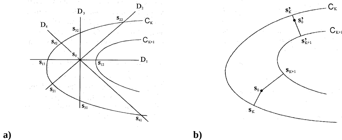
a) b) Figure 23 : Illustration des deux méthodes d'interpolation utilisant les lignes structurantes. En a) interpolation à partir des lignes de niveau C_k et C_{k+1} , et b) interpolation basée sur la ligne de plus grande pente. Source [Arnaud & Emery, 2000].
