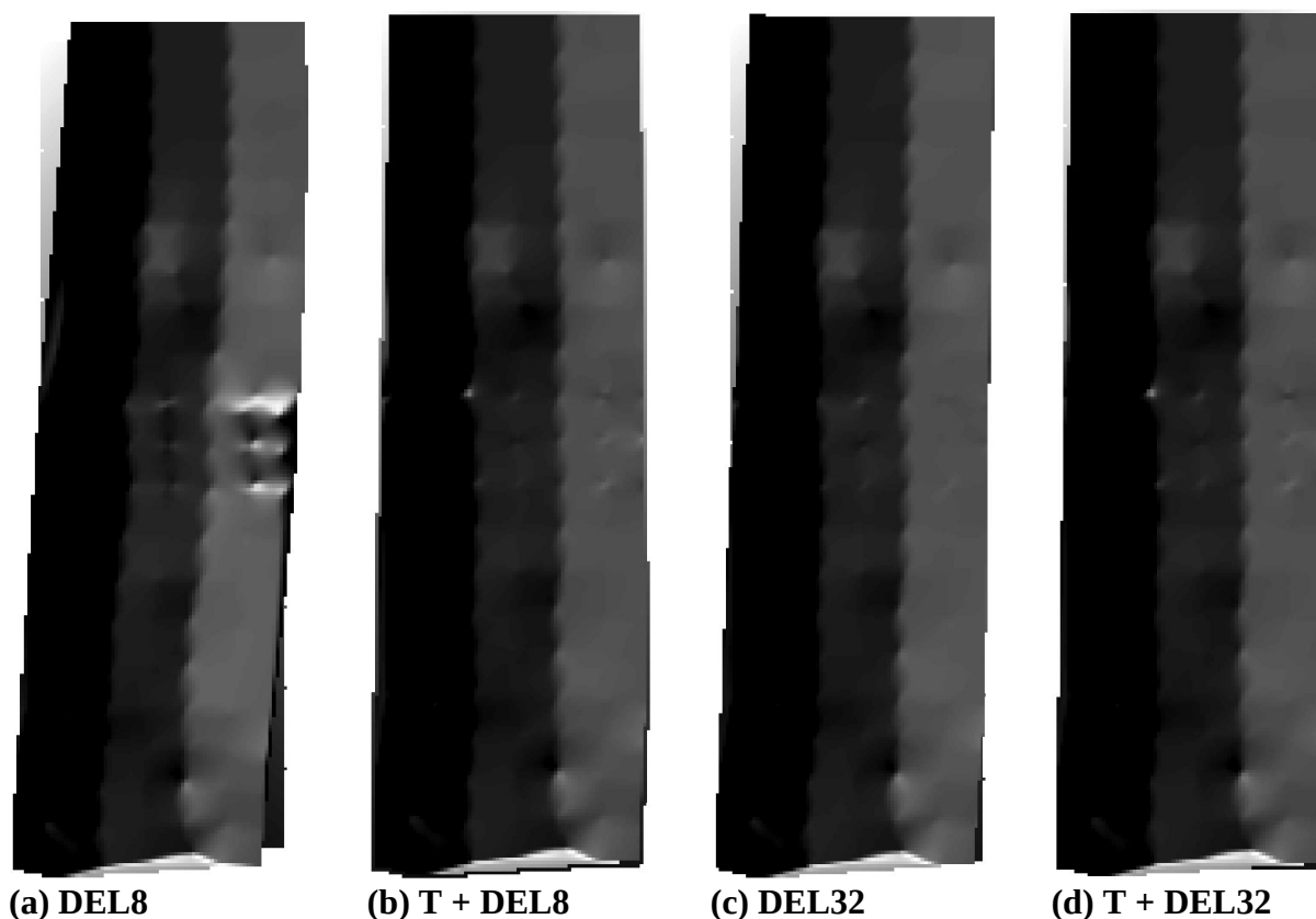
Figure 91 : Résultat de différentes méthodes de déformation élastique avec un rayon sur les modèles topographique et bathymétrique. En a) modèle déformé selon un rayon de 8 ; b) modèle translaté puis déformé selon un rayon de 8 ; c) modèle déformé selon un rayon de 32 ; d) modèle translaté puis déformé selon un rayon de 32.
