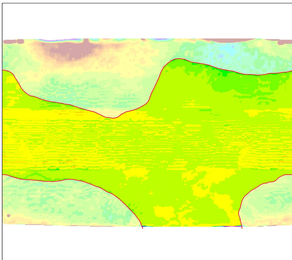
Figure 109 : Soustraction du modèle de référence et du modèle bathymétrique translaté.
