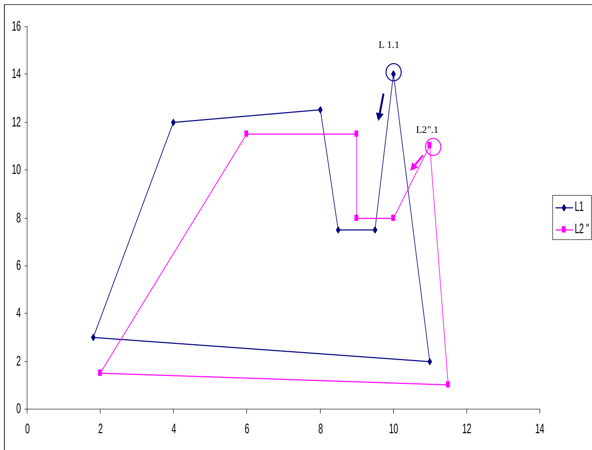
Figure 38 : Recherche du point homologue de L_{1,1} parmi les points de L_2 , et permutation du point trouvé de manière à ce qu'il devienne L_{2'',1} .
