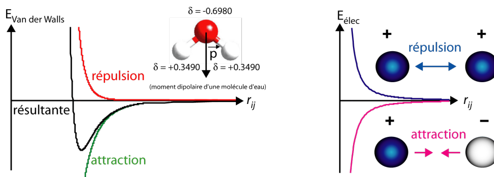
FIGURE 12.3 Représentation des termes non-liés de la fonction d'énergie potentielle.
