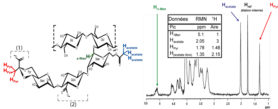
FIGURE 7.3 Structure chimique de l'unité répétitive du xanthane avec ses protons caractéristiques en RMN 1 H et spectre et données RMN 1 H. Dans notre échantillon de xanthane, l'acide glucuronique (2) -GlcA- est présent sur chaque monomère alors que l'acide pyruvique (1) -Pyr- n'est présent qu'un monomère sur deux.
