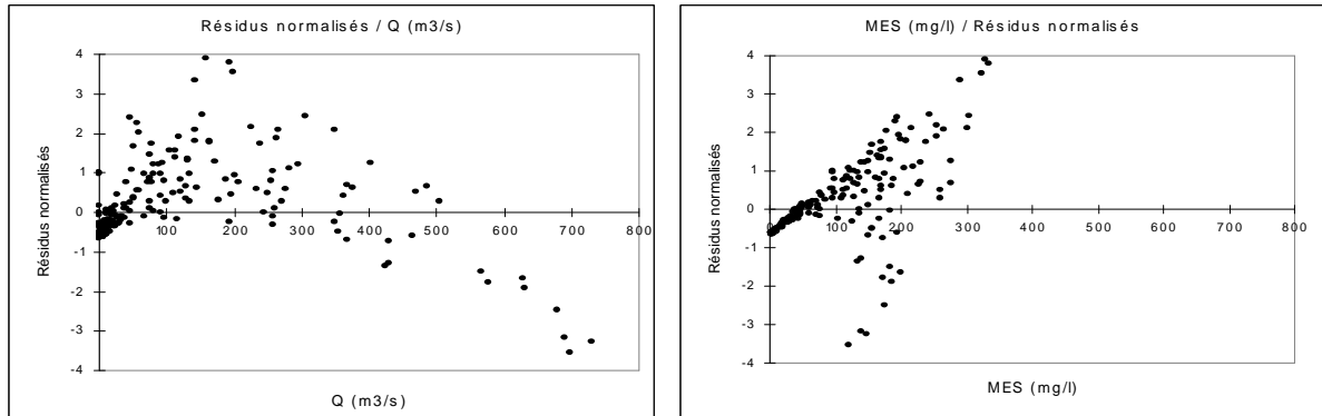
Figure 5.15 : Variation des résidus normalisés des débits et des MES de 1966 à 1967 dans le bassin-versant à Athiémé.
