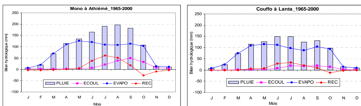
Figure 3.44 : Bilan hydrologique au pas de temps mensuel dans le bassin-versant du complexe Mono-Ahémé-Couffo.
