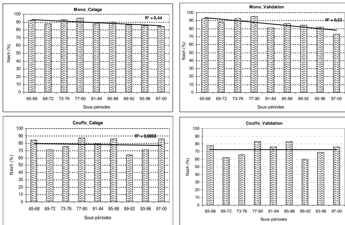
Figure 3.47 : Variabilité du Nash en calage et en validation sur les sous-périodes de 1965-2000 dans le bassin Mono-Couffo.
