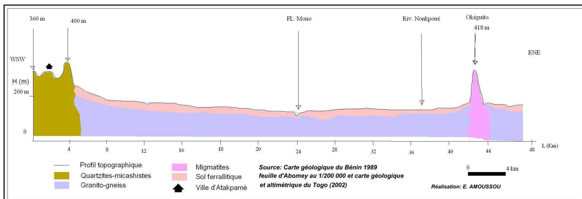
Figure 1.5 : Coupe de la pénéplaine cristalline entre le rebord montagneux (Atakpamé) et l'insertberg d'Okéguito.
