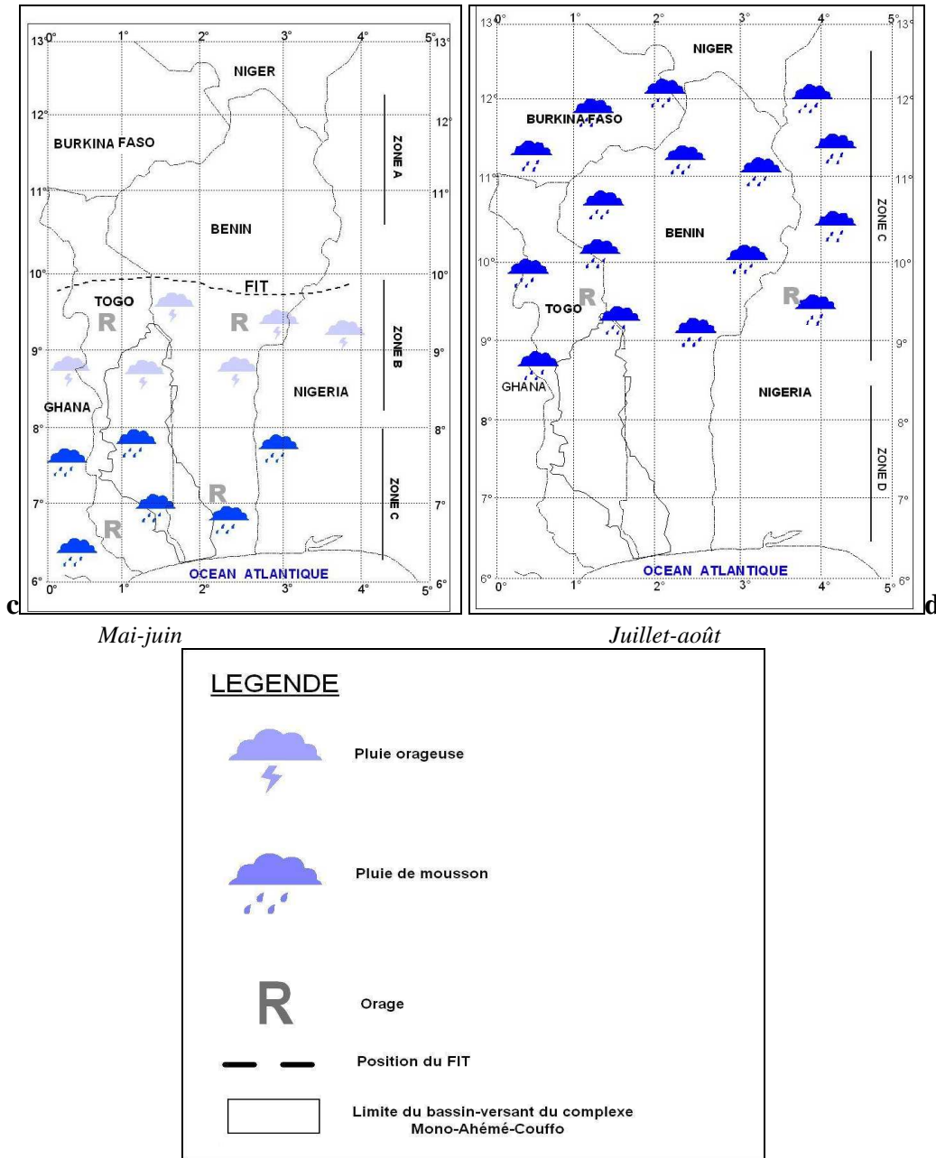
Figure 1.8 : Schéma de déplacement du FIT dans le bassin-versant.
