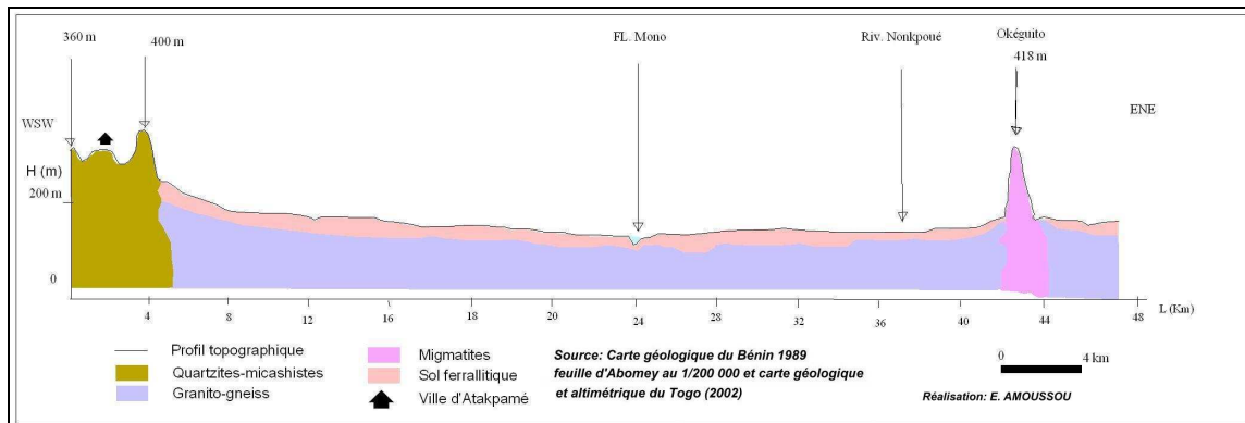
Figure 1.5 : Coupe de la pénéplaine cristalline entre le rebord montagneux (Atakpamé) et l'insertberg d'Okéguito.
