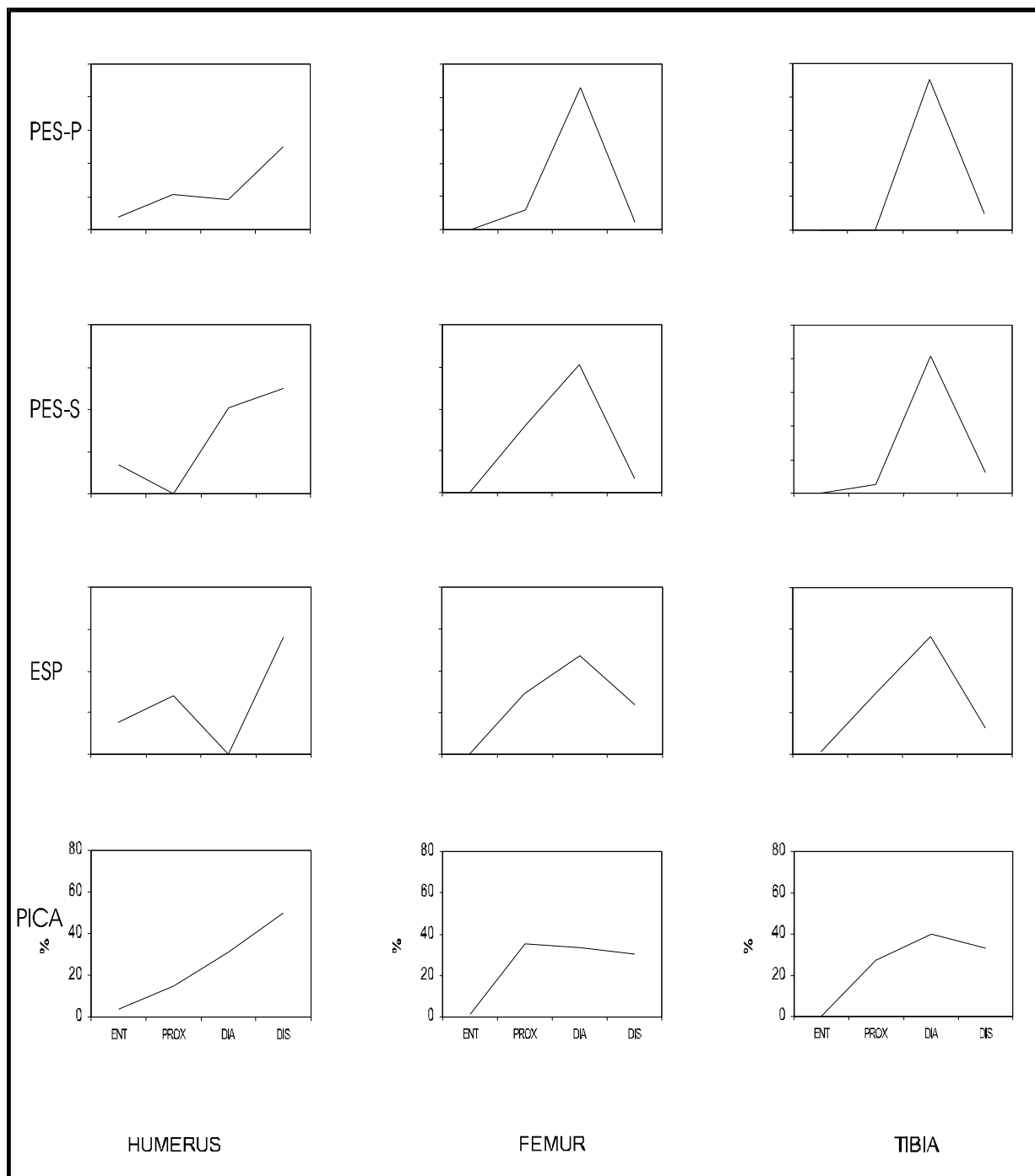
89 : Présentation des os longs (humérus, fémur et tibia) selon le modèle proposé par Perez-Ripoll (1992) des lapins de certains sites préhistoriques : Pas Estret salle terminale (PES-S), Pas-Estret Porche (PES-P), Esperit (ESP) et Picareiro (PIC).
