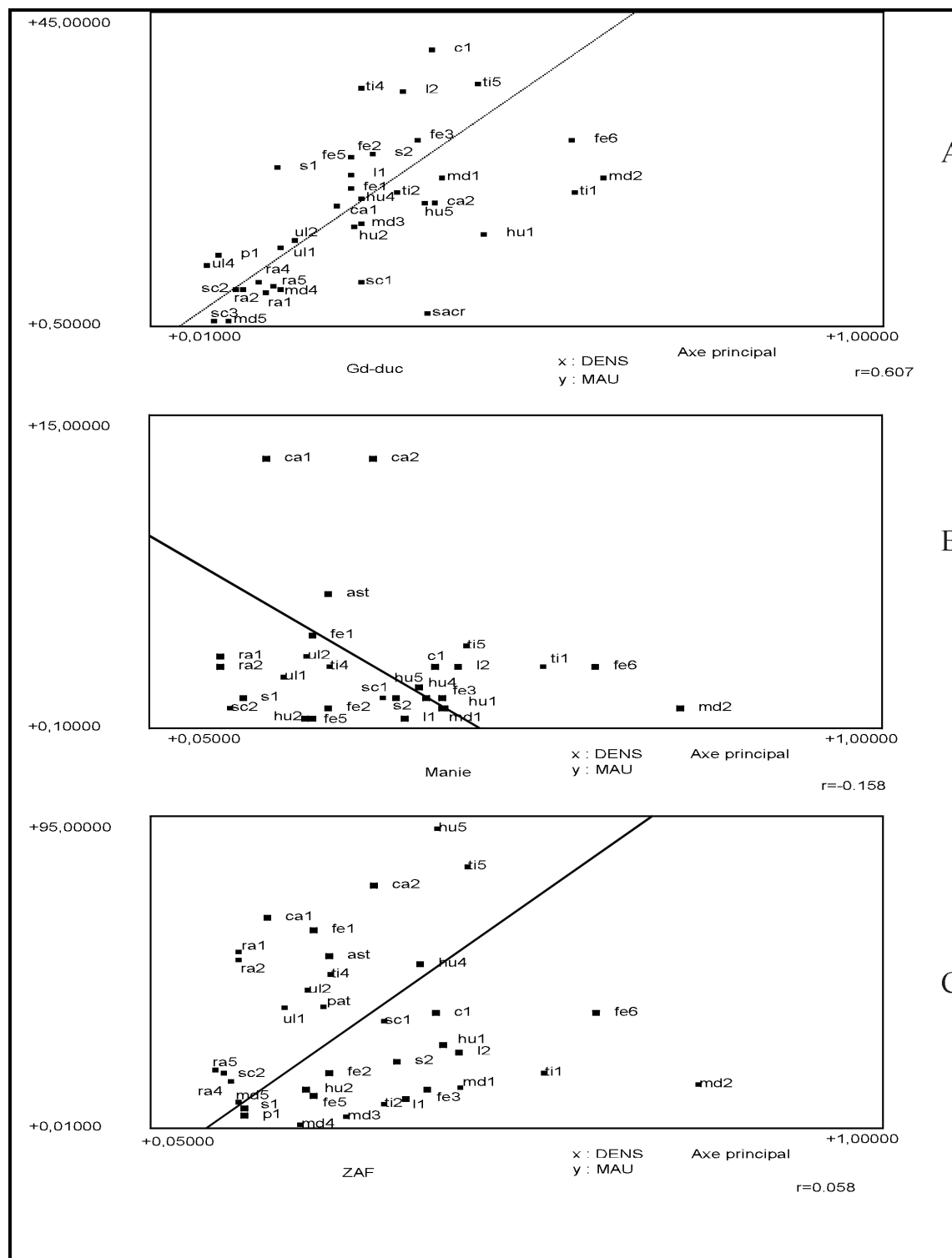
Fig. 93 : Relation entre l'abondance des éléments anatomiques des lapins et leur densité. A: Grand-duc, B: Arma delle Manie, C: Zaffaraya. Les valeurs de densité sont extraites de Pavao & Stahl (1999). Pour les abréviations, voir Fig. 92 a et b.
