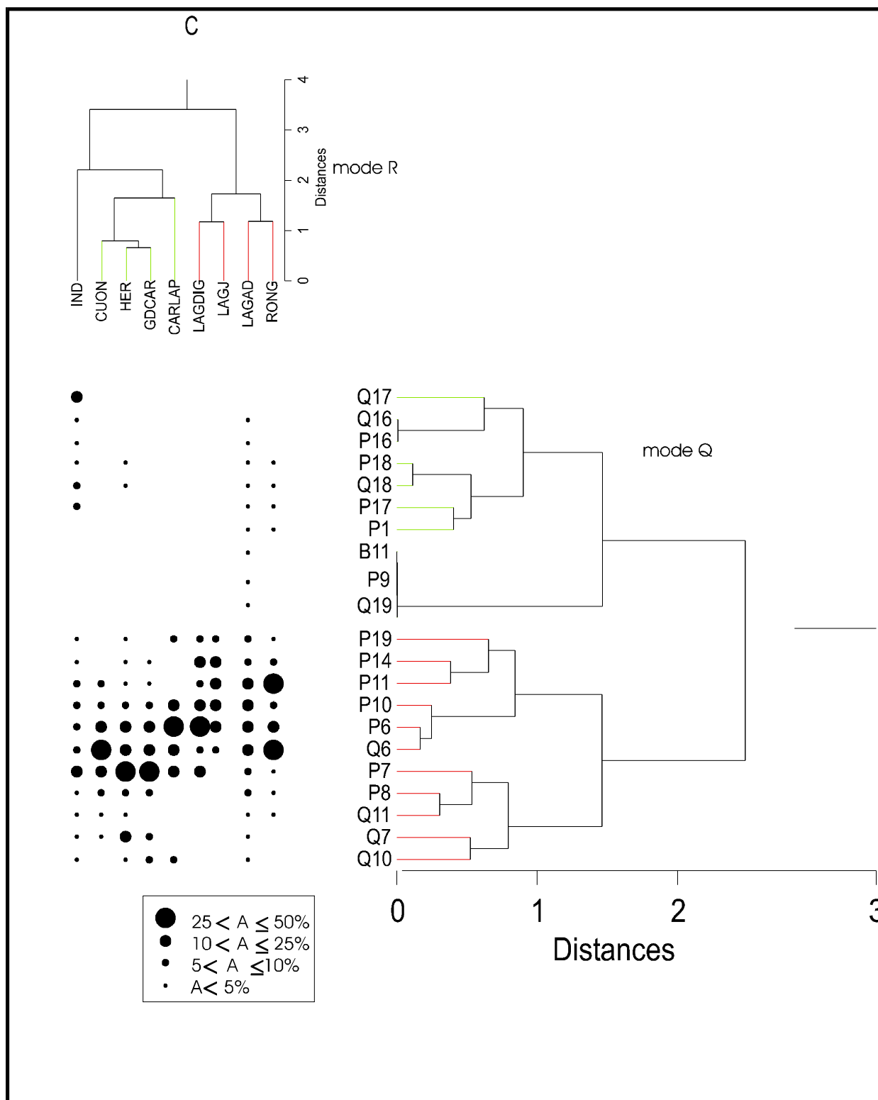
Fig. 64 : Analyse hiérarchique à double entrée (Two-way cluster) regroupant, selon les modes Q et R, les carrés et les objets archéologiques de l'unité archéostratigraphique C de Zafarraya. L'abondance relative des objets dans chaque carré est indiquée par des points proportionnels à leur effectif. Pour les abréviations, voir texte (paragraphe 3-6).
