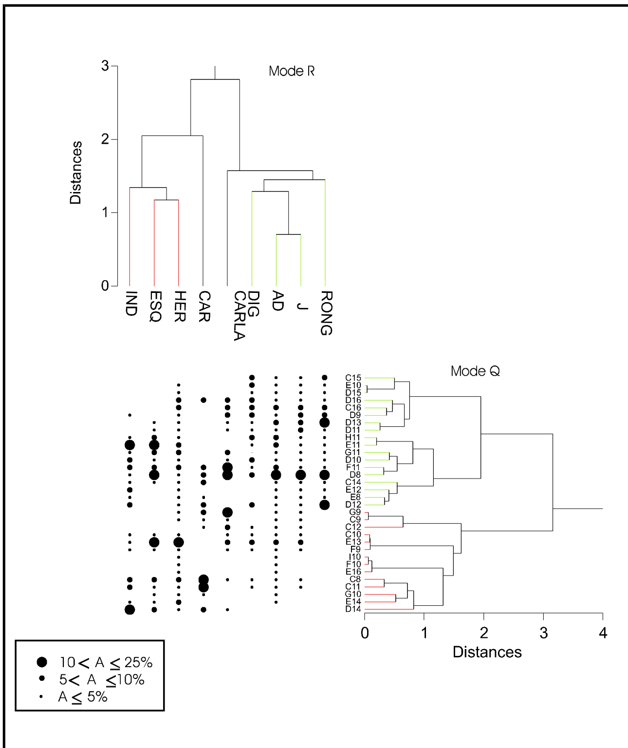
Fig. 50 : Analyse hiérarchique à double entrée (Two-way cluster) regroupant, selon les modes Q et R, les carrés et les objets archéologiques de la couche 7 d'Orgnac 3. L'abondance relative des objets dans chaque carré est indiquée par des points proportionnels à leur effectif. Pour les abréviations, voir texte (paragraphe 3-4).
