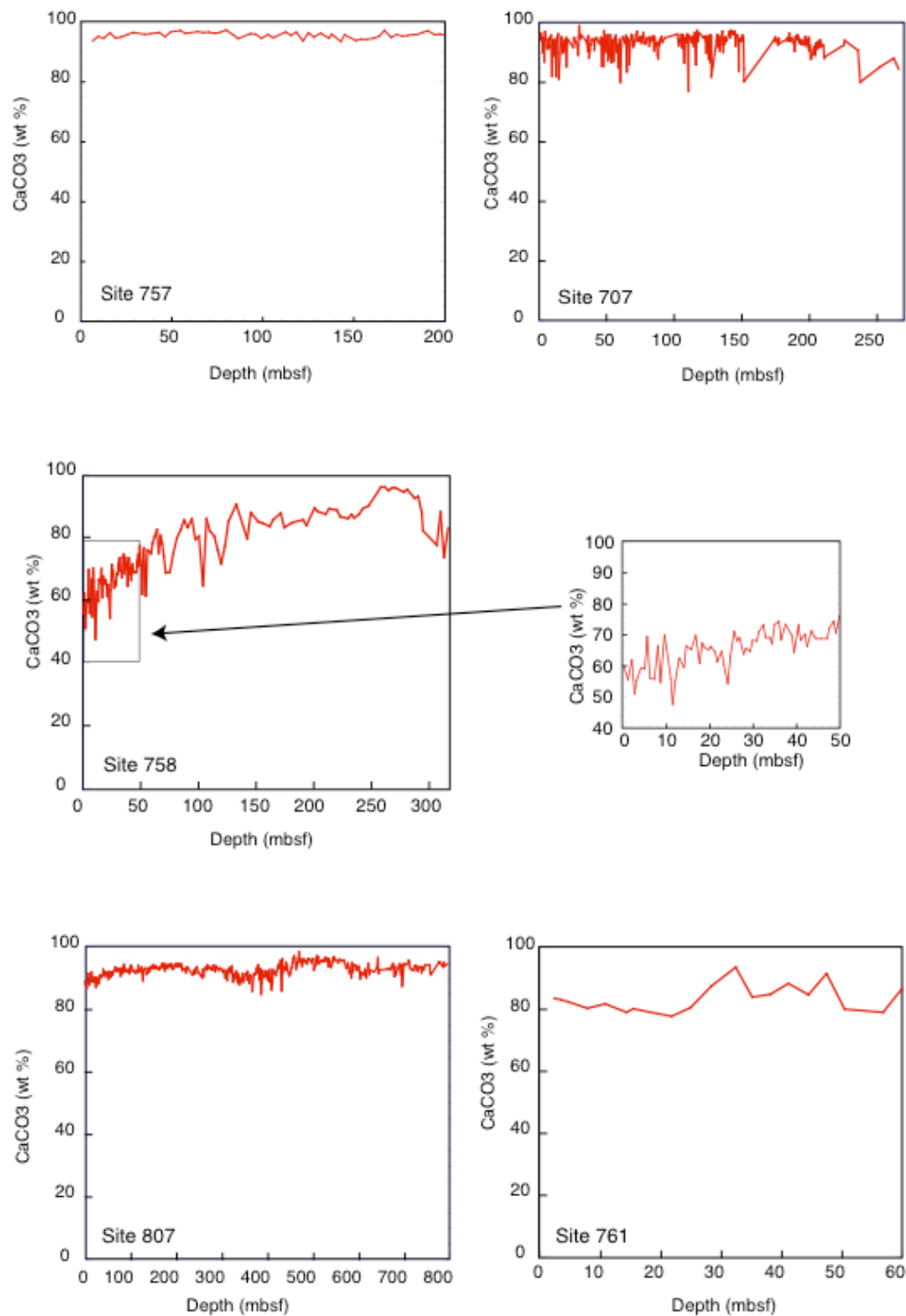
Fig □ Pourcentage en CaCO 3 des Sites 757,707,758, 807 et 761 en fonction de la profondeur. Les taux en carbonates sont élevés pour tous les Sites (> 80 %), sauf pour le Site 758 sur les 100 premiers mètres où l'on peut observer des taux diminuant jusqu'à 50 % (reflet d'une dilution par des apports détritiques importants liés à la formation de la chaîne Himalayenne).
