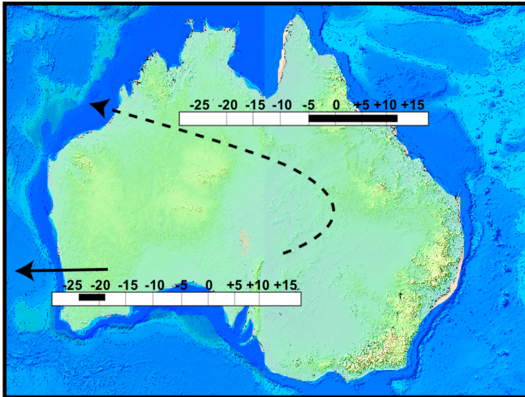
Fig 18: Carte topographique de l'Australie. Sont présentées les gammes de variations isotopiques en Nd des zones drainées par le fleuve Murchison (flèche noire □ Laboratoire de Géochimie-Cosmochimie, IPGP, données non publiées) et les zones balayées par les vents d'ouest (flèche noire en pointillée □ Grousset et al. , 1992 □ Rever-Rolland et al. , 2006 □ Hesse et al. , 2003). □
