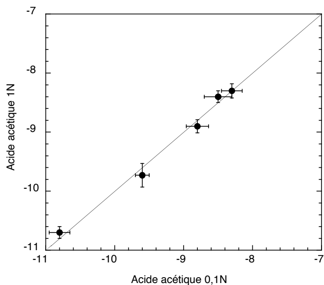
Fig 3 □ Comparaison de la composition isotopique en Nd obtenue par attaque en acide acétique 0,1 N et 1N pour 5 échantillons du Site 758 ayant des % en carbonates et des âges différents.
