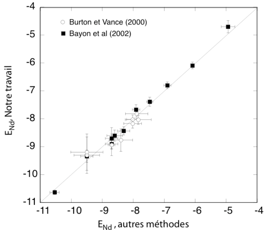
Fig 4 Comparaison des valeurs en ^{143}\text{Nd} de l'eau de mer obtenues par notre méthode (acide acétique) et ceux obtenues par la méthode de Bayon et al (2002), (carrés noirs) et Burton et Vance (2000), (ronds blancs) sur les mêmes échantillons.
