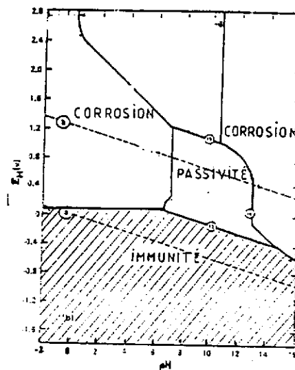
Fig. II.6 (à gauche) : diagramme potentiel-pH, du système Cu-Cl-H 2 O pour 355 ppm de chlorures, à 25°C [24;63].
