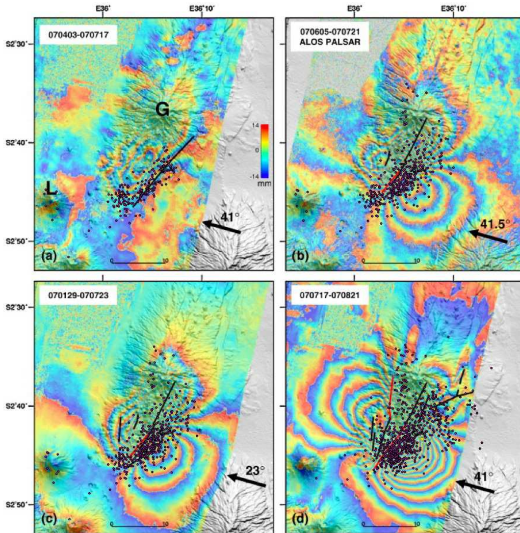
FIG. 3.4: Superposition de la sismicité (SEISMOTANZ'07, cercles roses) aux interférogrammes (périodes indiquées en haut à gauche de chaque cadre) et modèles calculés par Baer et al. (2008) (figure modifiée d'après Baer et al., 2008). Chaque frange représente un déplacement du sol de 2.8 cm dans la direction satellite-sol. Les flèches noires indiquent l'angle de vue du satellite, la valeur de l'angle d'incidence étant notée au-dessus. Les dykes et les failles déduits sont représentés respectivement par des traits rouges et noirs.
