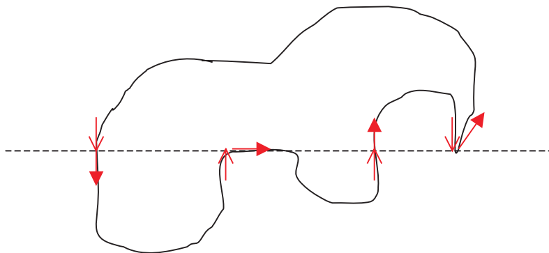
FIGURE 3.17 – Cas particuliers du test d'appartenance d'un point à une forme par une étude de position relative des pixels appartenant à la même ligne.
