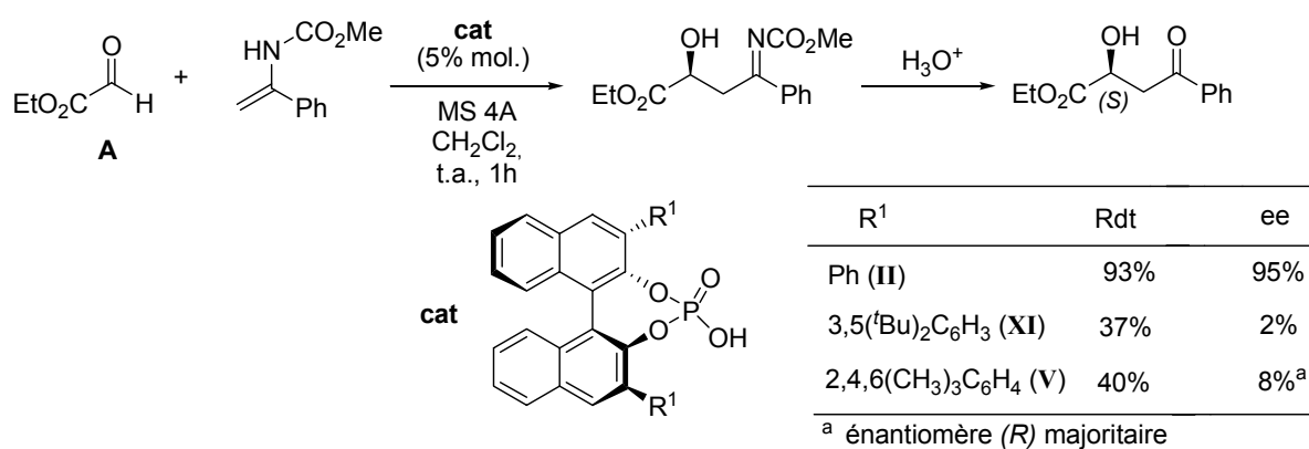
Schéma 10. Activation d'aldéhydes activés par des acides phosphoriques.
