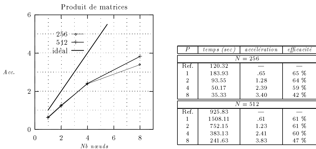
FIG. 6.1 - Produits de matrices distribuées par blocs
