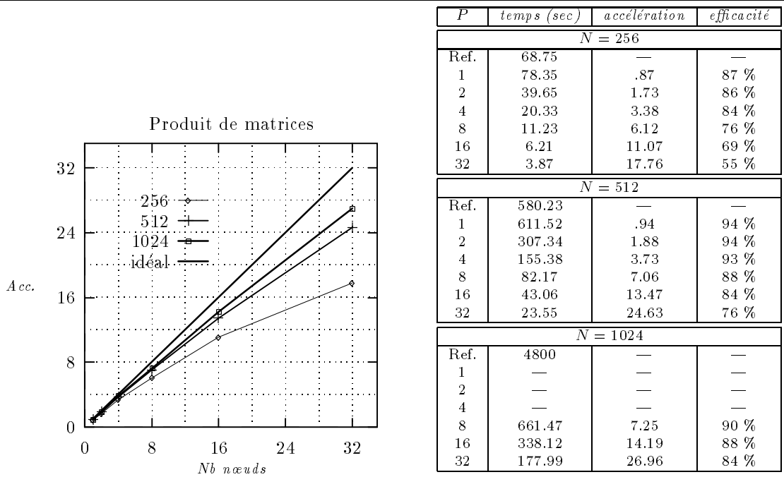
FIG. 6.6 - Produits de matrices distribuées par lignes et par colonnes
