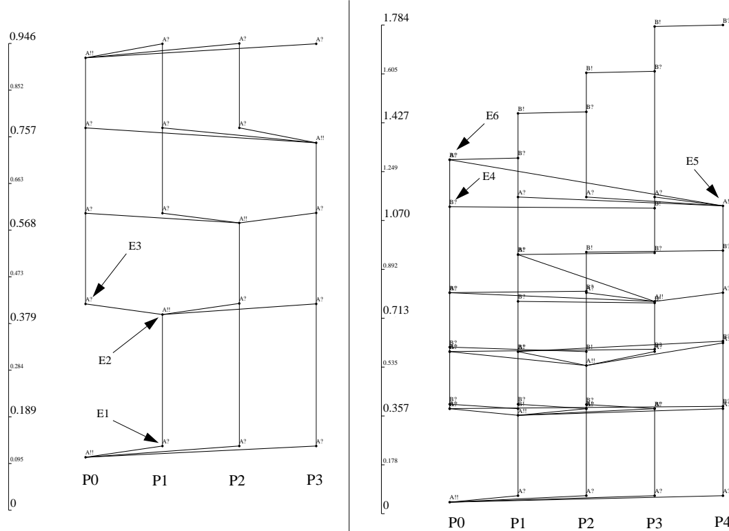
FIG. 4.5 - Comparaison du comportement temporel observé avec la distribution « idéale » (à gauche), et avec une distribution « non idéale » (à droite)
