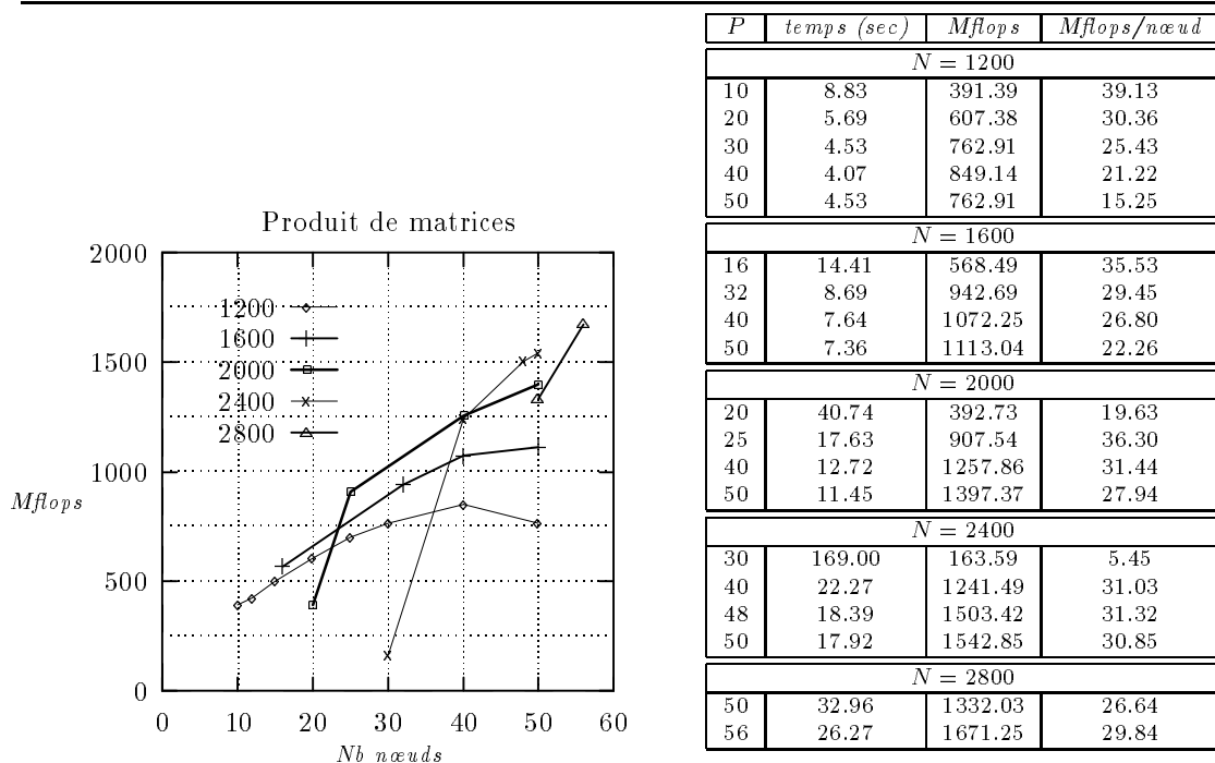
FIG. 6.8 - Produits de matrices distribués par blocs, avec appels à la routine DGEMM de BLAS-3
