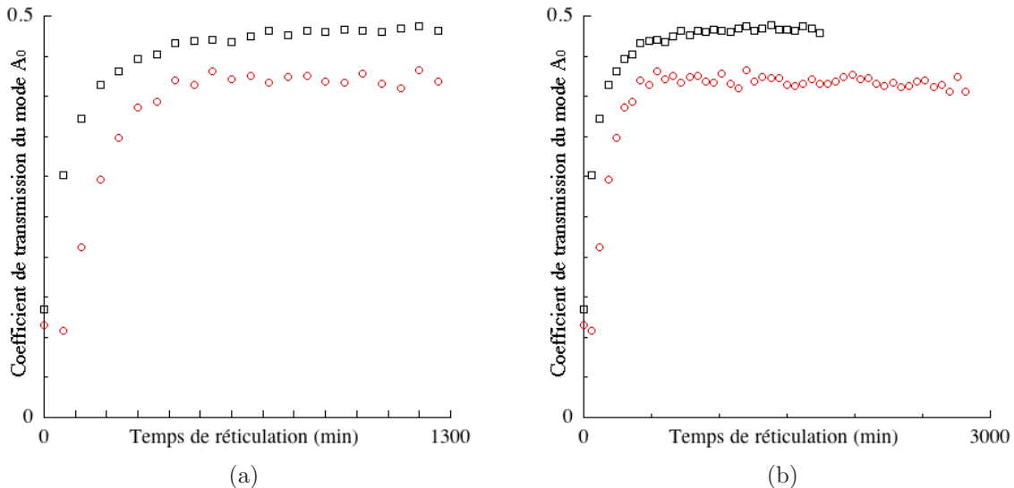
FIGURE 3.22 – Coefficient de transmission du mode A_0 mesuré expérimentalement à 0,4 MHz au cours du processus de réticulation d'un joint épais de 0,25^{\pm 0,05} mm collant une plaque d'aluminium sablée ( \square ) ou juste poncée ( \circ ) et un patch de 3,46 mm de plexiglas, (a) entre 0 et 1300 min et (b) entre 0 et 2 jours.
