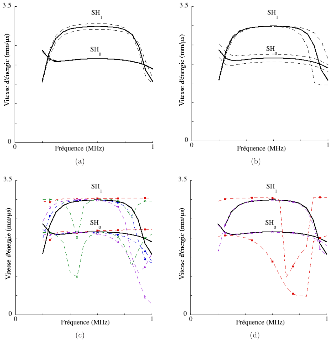
FIGURE B.1 – Prédictions numériques de la sensibilité de la vitesse d'énergie des modes SH_0 et SH_1 d'un assemblage collé (—) (a) à une variation de \pm 5\% du C_{44} = C_{55} de l'aluminium (---); (b) à une variation de \pm 10\% des C_{44} et C_{55} du patch (---); (c) à une chute de 27% (—●—), 50% (—□—), 90% (—○—) et 99% (—■—) du C_{44} = C_{55} de la colle et (d) à une chute de 50% (—□—) et 99% (—■—) du k_T de l'interface.
