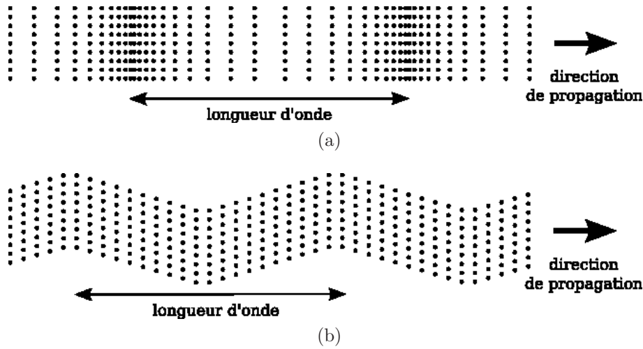
FIGURE 2.2 – Déplacements induits par (a) une onde longitudinale (ou onde de compression) et (b) une onde transverse (ou onde de cisaillement).
