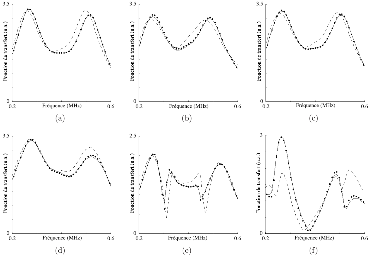
FIGURE 1.11 – Fonctions de transfert simulées (●) et calculées avec des C_{ij} optimisés (—) et non optimisés (– –) du champ transmis à travers un carbone époxy [0^\circ / 90^\circ]_{8s} et pour un angle d’incidence de 0^\circ (a), 15^\circ (b), 20^\circ (c) et 30^\circ (d) dans le plan principal P_{12} ainsi que de 6^\circ (e), 13^\circ (f) dans le plan P_{45^\circ} .
