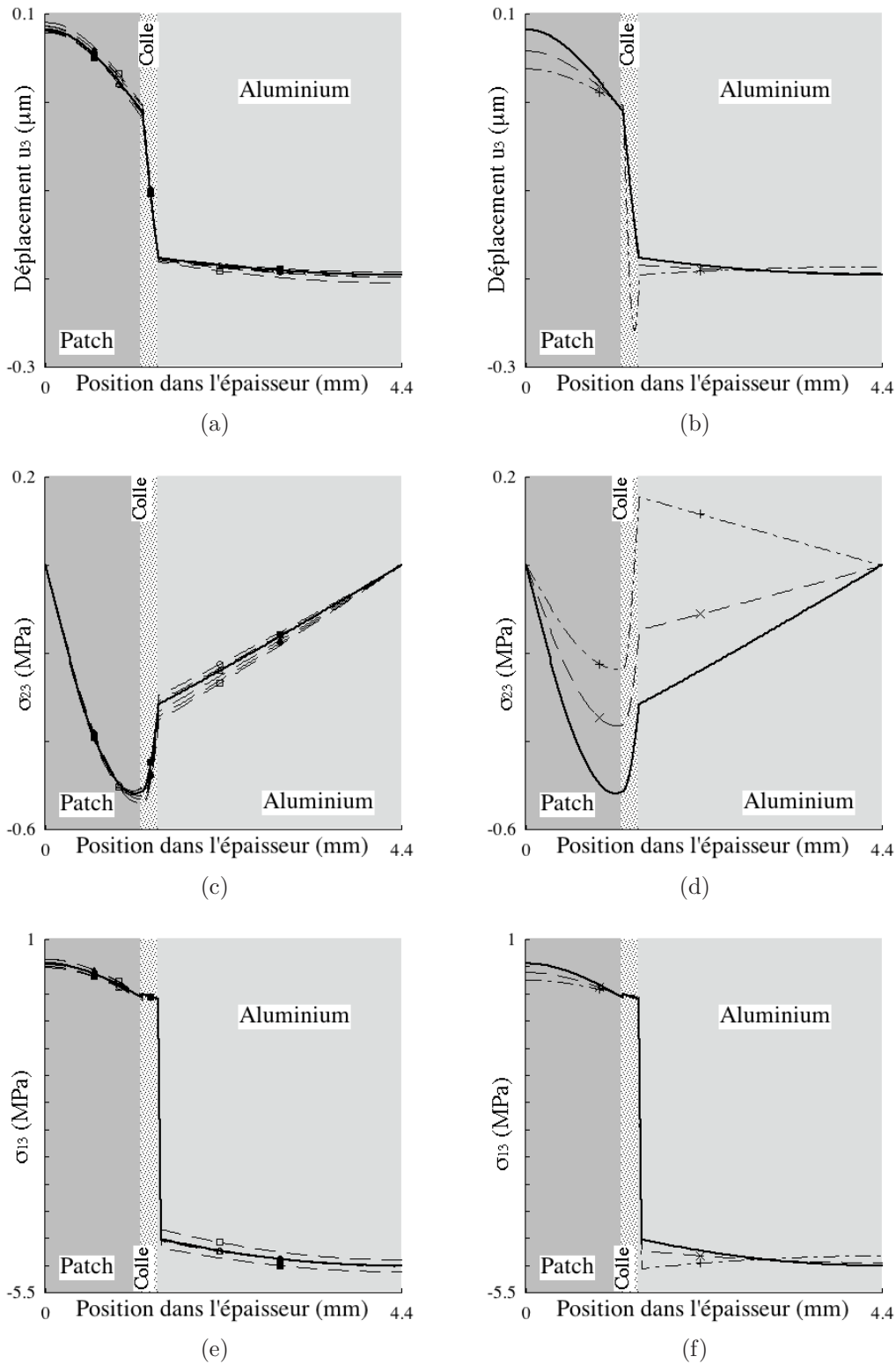
FIGURE 2.10 – Prédictions numériques de la distribution dans l'épaisseur des déplacements (a) et (b), de la contrainte \sigma_{23} (b) et (d), et de la contrainte \sigma_{13} (e) et (f), normalisés en puissance, (—) pour un assemblage de propriétés nominales; colonne de gauche pour les variations de propriétés des substrats : +5% (—■—) et -5% (—□—) du C_{44} de l'aluminium, +10% (—▲—) et -10% (—△—) du C_{44} et +10% (—●—) et -10% (—○—) du C_{55} du patch composite; colonne de droite pour les variations de propriétés de la colle : -40% (—×—) et -85% (—+—) du C_{44} de la colle. Mode SH_1 à 500 kHz.
