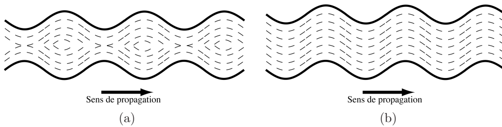
FIGURE 3.1 – Type de déplacements induits par des ondes de Lamb symétriques (a) et antisymétriques (b).
