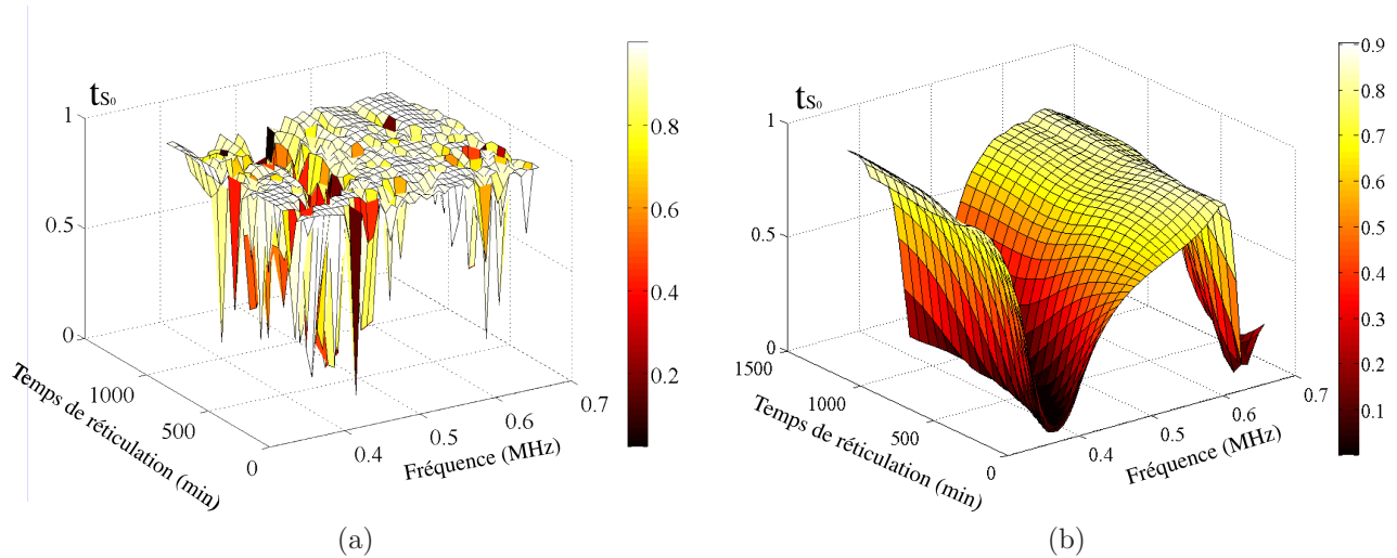
FIGURE 3.14 – Evolution du coefficient de transmission du mode guidé S_0 se propageant le long d’un assemblage aluminium / colle / plexiglas (a) élastique et (b) viscoélastique, pendant la réticulation du joint de colle et pour des fréquences variant de 0,3 à 0,6 MHz .
