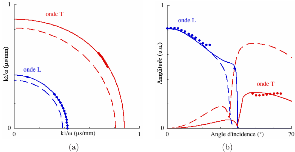
FIGURE 1.6 – Lenteurs de phase (a) et amplitudes (b) mesurées (●) et calculées avec des C_{ij} initiaux (---) et optimisés (—) des ondes longitudinales et transverses se propageant dans le plan P_{12} d'un plexiglas épais de 1 mm.
