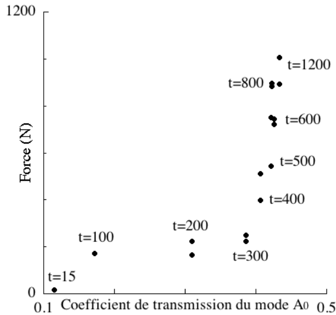
FIGURE 3.27 – Confrontation entre les résultats des essais de traction uni-axiale et des mesures ultrasonores ( A_0 incident à 0,4 \text{ MHz} ) réalisés sur un assemblage aluminium / colle / plexiglas de 3,46 \text{ mm} .
