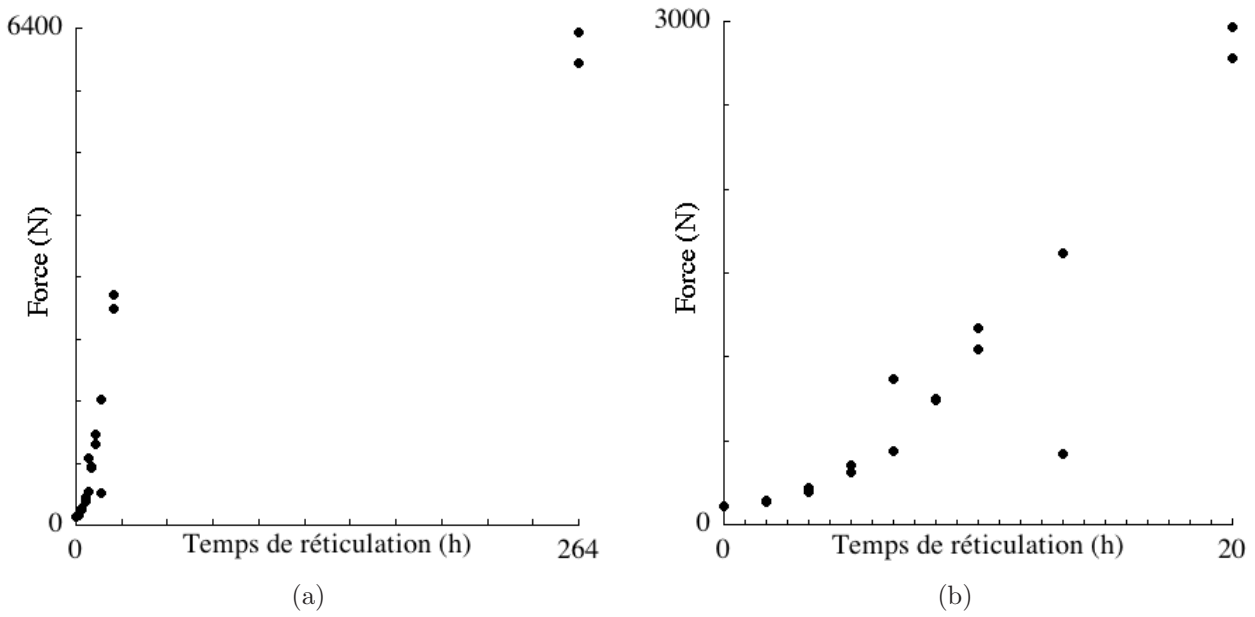
FIGURE 3.28 – Forces d’arrachement obtenues lors d’essais de traction uni-axiale sur un assemblage aluminium / joint n°1 / composite / joint n°2 / aluminium, pour différents temps de réticulation du joint de colle n°2 des éprouvettes, (a) pour l’ensemble des temps de mesures et (b) pour les temps allant de 15 à 1200 min .
