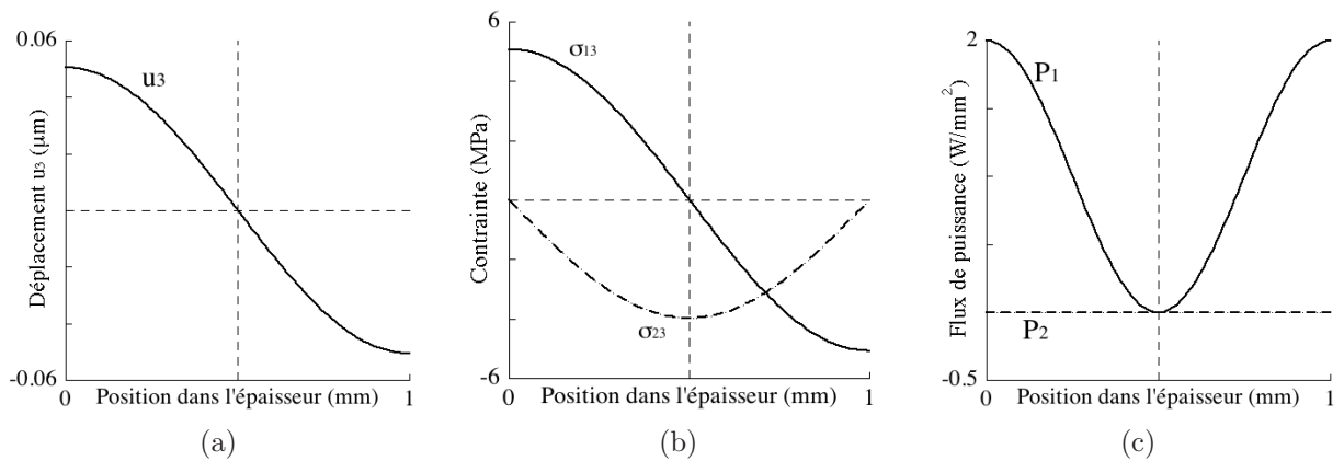
FIGURE 2.4 – Distribution des champs de déplacement (a), de contraintes (b) et du flux de puissance (c) du mode SH_1 dans l’épaisseur d’une plaque d’aluminium de 1\text{ mm} à 2,5\text{ MHz} .
