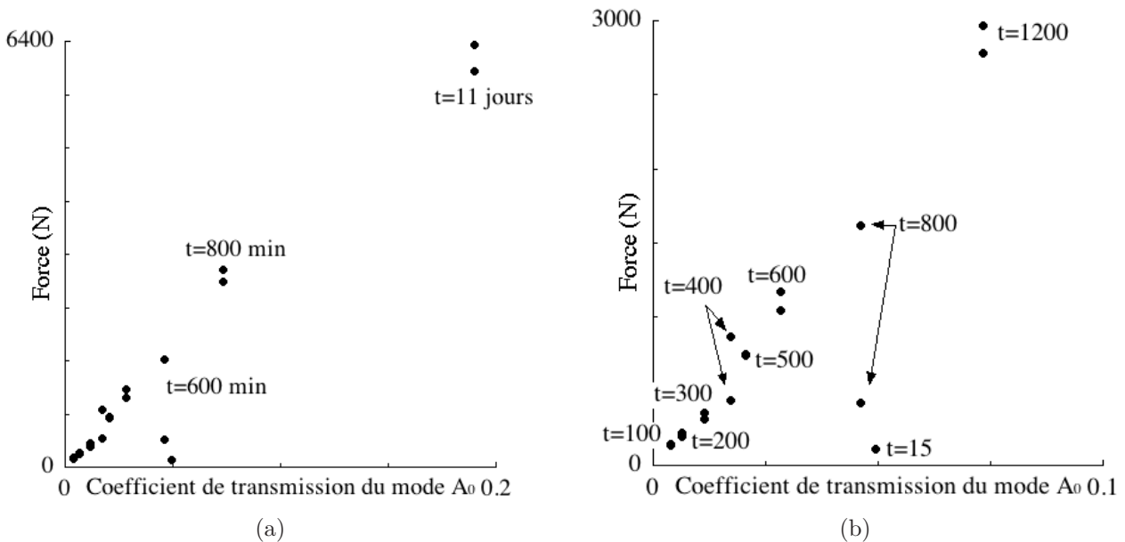
FIGURE 3.29 – Corrélation des essais de traction uni-axiale et des mesures ultrasonores réalisés sur un assemblage aluminium / colle / composite, (a) pour l’ensemble des temps de mesures et (b) pour les temps allant de 15 à 1200 min .
