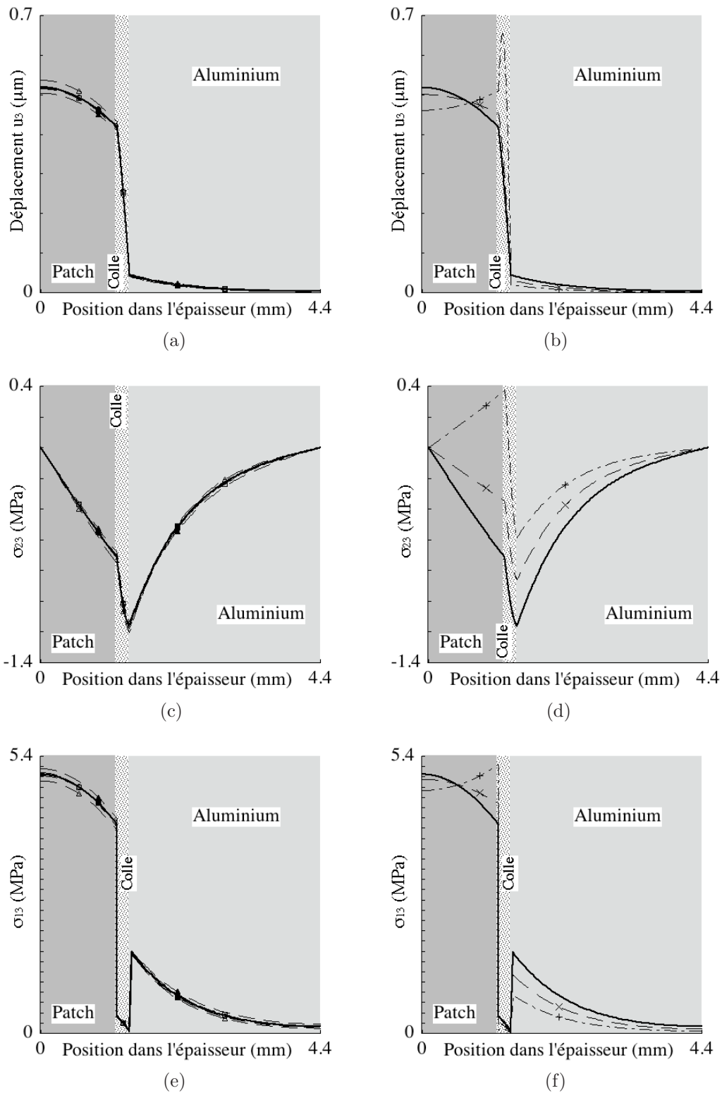
FIGURE A.2 – Prédictions numériques de la distribution dans l'épaisseur des déplacements (a) et (b), de la contrainte \sigma_{23} (b) et (d), et de la contrainte \sigma_{13} (e) et (f), normalisés en puissance. (—) pour un assemblage de propriétés nominales; colonne de gauche pour les variations de propriétés des substrats : +5% (—■—) et -5% (—□—) du C_{44} de l'aluminium, +10% (—▲—) et -10% (—△—) du C_{44} et +10% (—●—) et -10% (—○—) du C_{55} du patch composite; colonne de droite pour les variations de propriétés de la colle : -40% (—×—) et -85% (—+—) du C_{44} de la colle. Mode SH_0 à 500 kHz.
