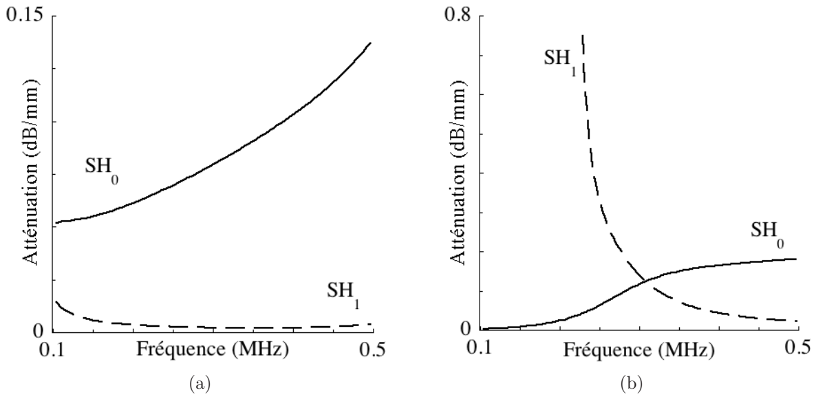
FIGURE 2.16 – Atténuation des modes SH_0 et SH_1 se propageant le long d’un assemblage aluminium/colle/patch (a) pour une colle non réticulée i.e. 45 min après la réalisation du collage et (b) pour une colle réticulée, i.e. plusieurs jours après la réalisation du collage.
