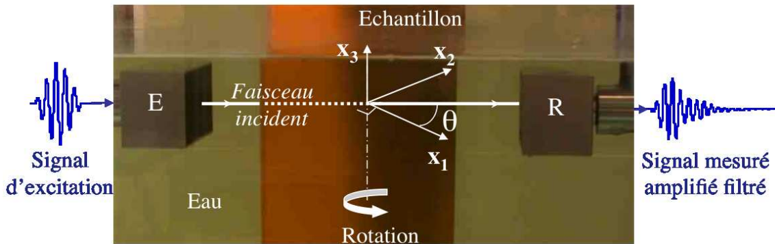
FIGURE 1.3 – Dispositif expérimental utilisé lors des caractérisations de matériaux par les méthodes ultrasonores à immersion.
