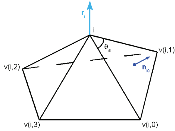
FIG. 5.5 – Définition de la normale au sommet i en fonction des normales unitaires \mathbf{n}_{i,k} des facettes voisines et des angles adjacents au sommet \theta_{i,k} .
