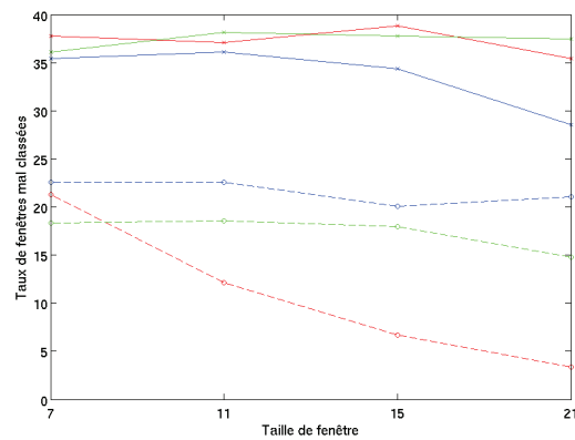
FIG. 7.10 – Taux de fenêtres mal classées pour l’ensemble des images utilisées pour l’apprentissage (courbes pointillées), et l’ensemble des images test (courbes continues), en se basant sur les moments de Krawtchouk (vert), Legendre (rouge) ou Zernike (bleu) en fonction des tailles de fenêtres.
