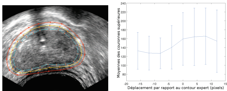
FIG. 3.15 – Evolution des moyennes et écarts-types sur le contour expert (jaune) rétréci et dilaté sur une coupe centrale bien contrastée. Le contour rouge (resp. cyan) représente le contour expert dilaté (resp. rétréci) de 16 pixels.
