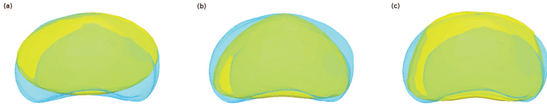
FIG. 5.9 – Vues 3D des maillages initiaux (jaune) correspondant aux différentes configurations du placement des points initiaux de la figure 5.8 superposées à la référence expert (cyan).
