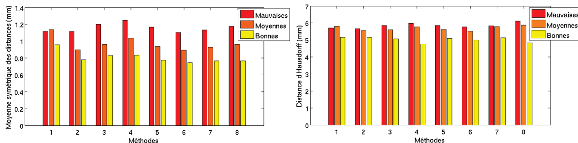
FIG. 6.16 – Evolution des distances moyennes et maximales en fonction de la qualité de la base de données.
