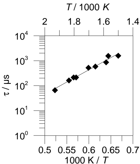
Figure 3.36 : Mesure des délais d'auto-inflammation du mélange 90% CH 4 / 10% H 2 , \phi = 1 , p_5 = 10 \pm 1 bar, ◆ expérience / ligne : courbe de tendance
