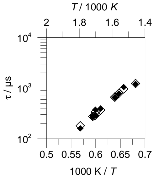
Figure 3.35 : Confrontation corrélation / expérience des délais d'auto-inflammation du méthane pur, \phi = 0,2 , p_5 = 10,1 \pm 1,01 bar, expérience (◆), corrélation (◇)
