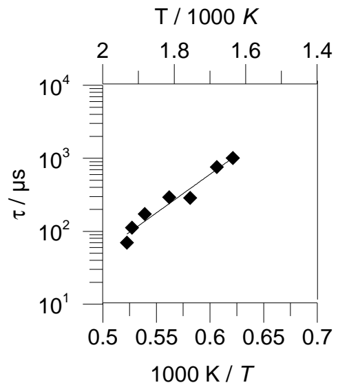
Figure 3.37 : Mesure des délais d'auto-inflammation du mélange 90% CH 4 / 10% H 2 , \phi = 2 , p_5 = 10 \pm 1 bar, ◆ expérience / ligne : courbe de tendance.
