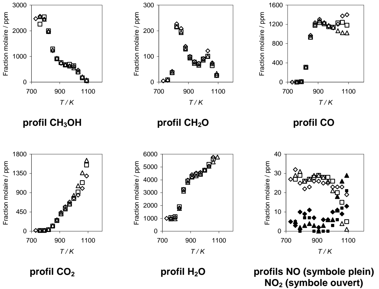
Figure 3.7 : Effet de \text{NO}_2 sur l'oxydation du méthanol en RPA. Conditions expérimentales : 2500 ppm de \text{CH}_3\text{OH} , 25 ppm \text{NO}_2 , \tau = 0.8 sec, p = 10 bar. \phi = 1 ( \Delta ) \phi = 0.6 ( \square ) \phi = 0.3 ( \diamond )
