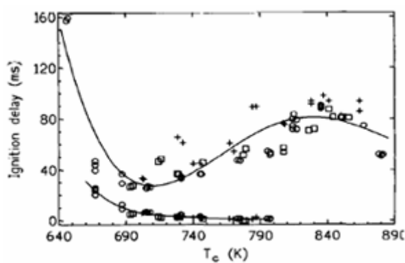
Figure 3.20 [27] : influence du temps de compression sur les délais du n-heptane. La flamme froide (ligne du bas) n'y est pas sensible
