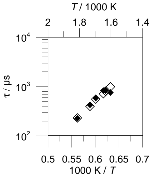
Figure 3.34 : Confrontation corrélation / expérience des délais d'auto-inflammation du méthane pur, \phi = 1 , p_5 = 10,4 \pm 1,04 bar, expérience (◆), corrélation (◇)
