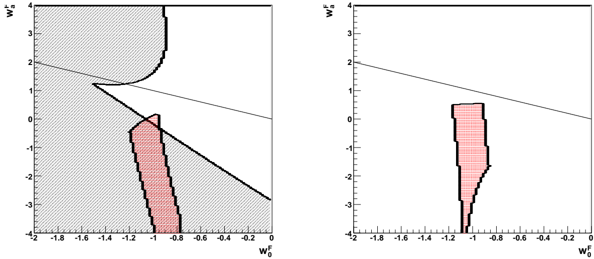
FIGURE 4.9 – Résultats de l'analyse dans le plan (w_0^F, w_a^F) . A gauche : \Omega_M^F = 0.35 , à droite : \Omega_M^F = 0.3 . Zone hachurée en noir : zones de biais (si l'un au moins des deux paramètres est mal reconstruit). Zone blanche : zone de validité (les deux paramètres sont bien reconstruits). Zone hachurées en rouge : zone de confusion avec le modèle \Lambda CDM (si w_0 est compatible avec -1 et w_a compatible avec 0 , l'équation d'état reconstruite correspond à celle de la constante cosmologique).
