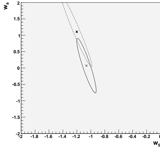
FIGURE 6.5 – Ellipses de Fisher à 1\sigma illustrant les résultats, dans le scénario à court terme, des ajustements du modèle \Omega_M^F = 0.3 , \Omega_X^F = 0.66 , w_0 = -1.2 , w_a = 1.1 , avec l’hypothèse de platitude (trait plein) ou sans (pointillés). L’astérisque signale le modèle simulé.
