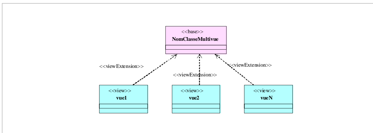
Figure III.10. Structure statique d'une classe multivue [Nassar, 05]
