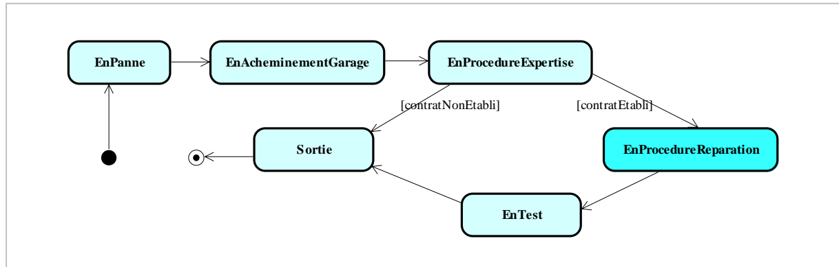
Figure IV.3. Machine-base associée à la classe Voiture
