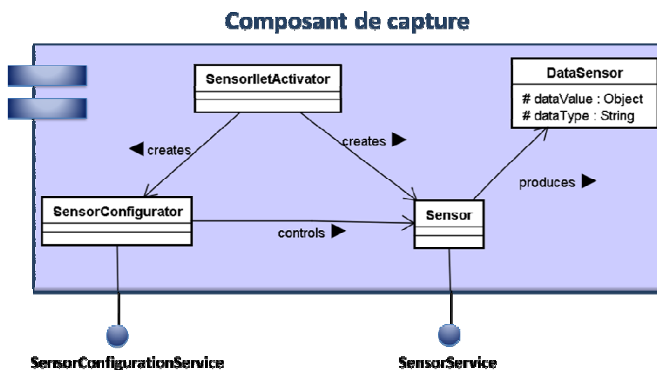
Figure 88 - Organisation interne d'un composant de capture de contexte (composant du type Sensor ).
