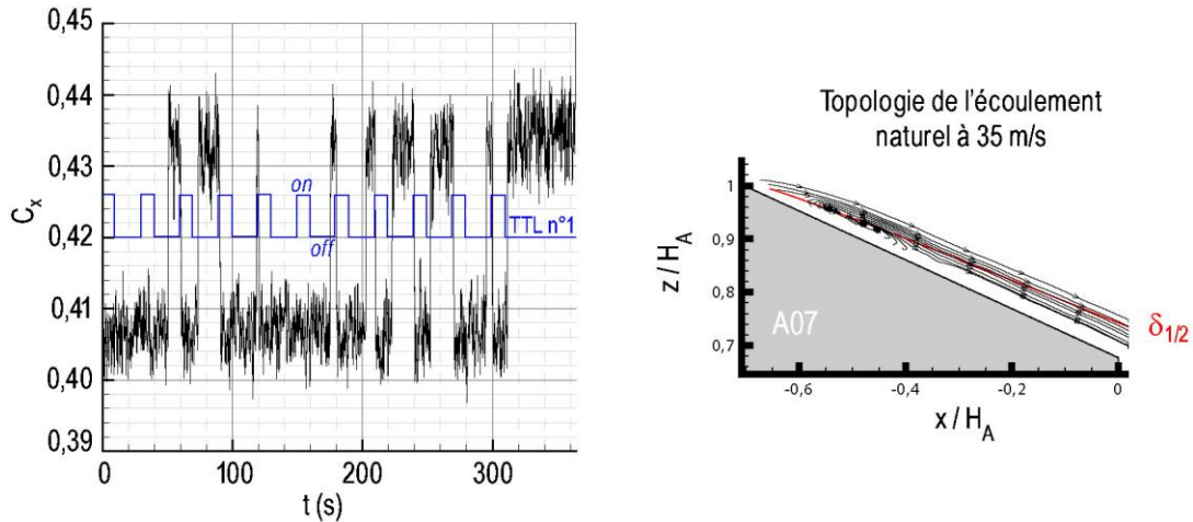
Figure 4.23 – Phénomène d’hystérésis sur la traînée observé pour U_\infty = 35 m/s (A0,7, n^\circ_{act1} , V_{HV} = 16 kV, f_{HV} = 1 kHz)
