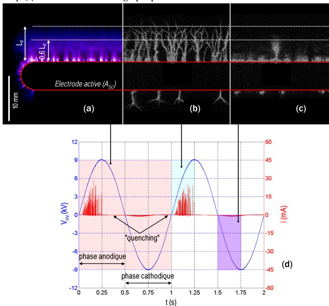
Figure 2.6 – (a) Visualisation intégrée en temps comparée à l'imagerie ICCD ( 250 \mu\text{s} ) pour (b) la phase anodique et (c) la phase cathodique, corrélée au (d) courant de décharge pour A_{SC} ( V_{HV} = 9 kV, f_{HV} = 1 kHz)
