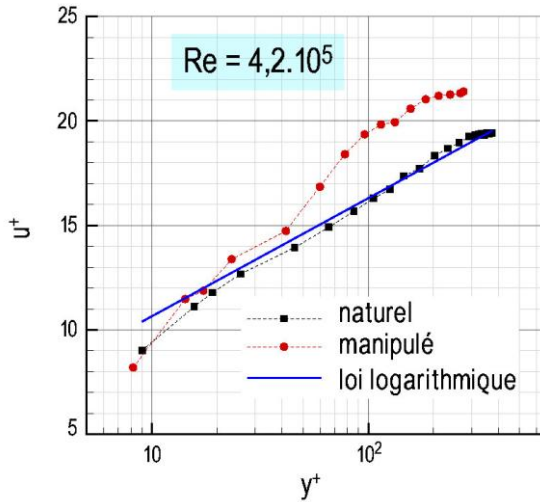
Figure 3.22 – Comparaison des profils de vitesse à la loi logarithmique pour Re = 4,2 \cdot 10^5 ( V_{HV} = 12 \text{ kV} , f_{HV} = 1 \text{ kHz} )
