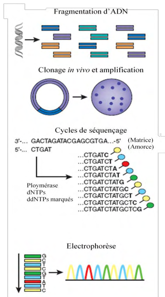
Figure 6. Etapes du séquençage Sanger (Shendure, 2008)
