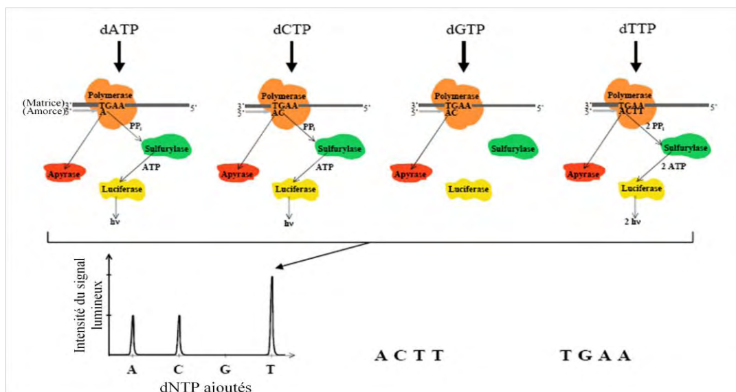
Figure 7. Etapes du pyroséquençage (Ahmadian et al. , 2006).
