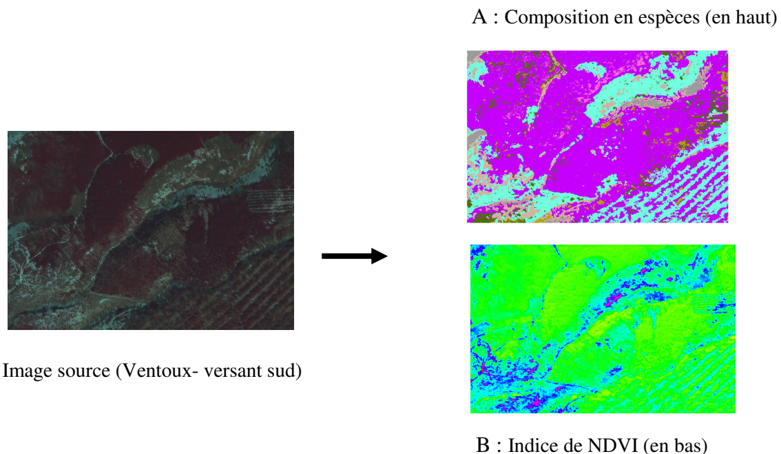
Figure 28. Données utilisées pour la mesure de biodiversité.
