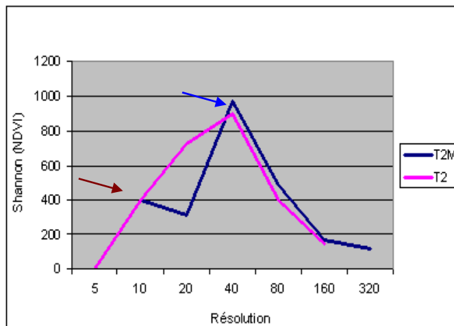
Figure 60. Perte relative de diversité (%) calculée avec l'indice de Shannon à travers des échelles (m) pour deux images de différentes formes (T2M= Carré, T2= rectangulaire) : cas du NDVI.
