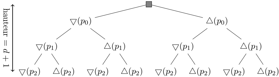
FIGURE 3.2.: Différentes combinaisons d'arrondi pour p^* de degré d = 2
