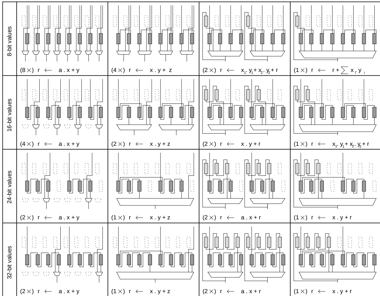
FIGURE 2.3.: Cellule linéaire et de multiplication de FPOP et quelques configurations possibles.
