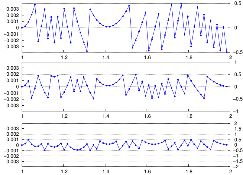
FIGURE 2.11.: Courbes d'erreur pour f = 1/x , n = 6 et différents nombres de bits de garde : g = 1 (haut), g = 2 (milieu) et g = 3 (bas).
