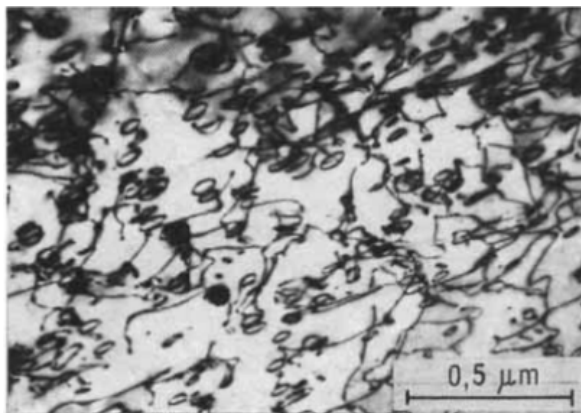
Fig. 0.1. Boucles d'Orowan autour de précipités non cisillables
