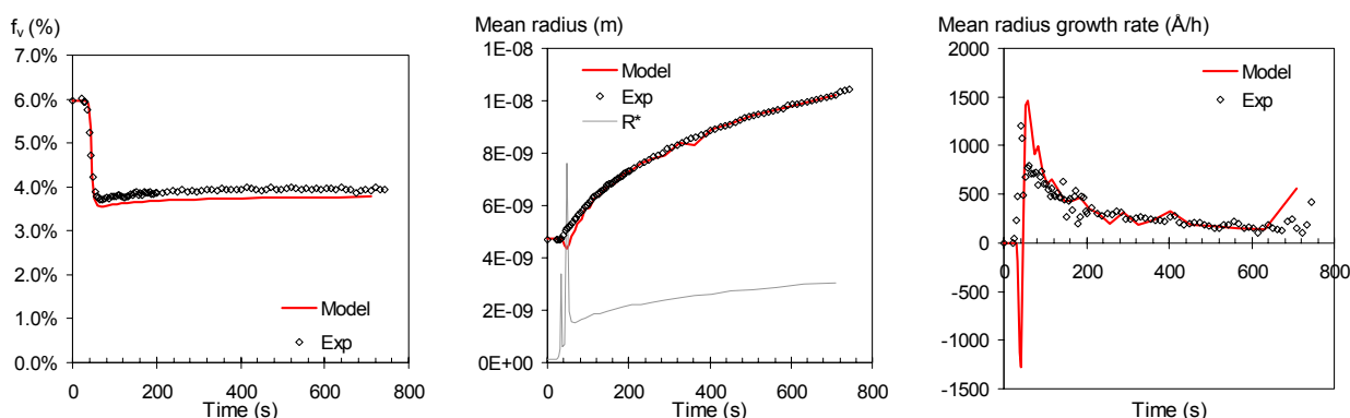
Fig. 0.18. Cinétique de précipitation sous l'effet d'un traitement isotherme à 240°C
