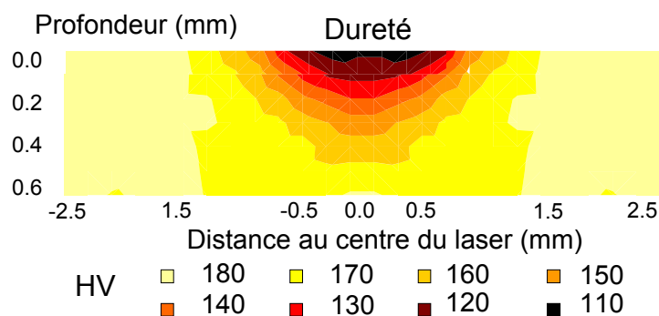
Fig. 0.14. Cartographie de dureté après traitement laser
