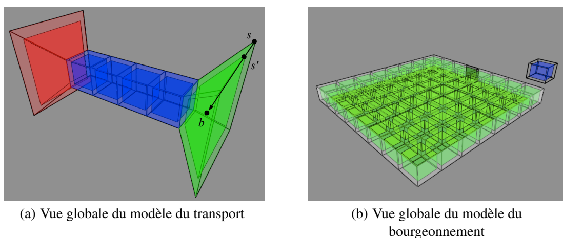
FIGURE 7.16 – Visualisation simultanée des compartiments et des membranes
