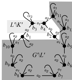
(b) Une 2-G-carte G'
