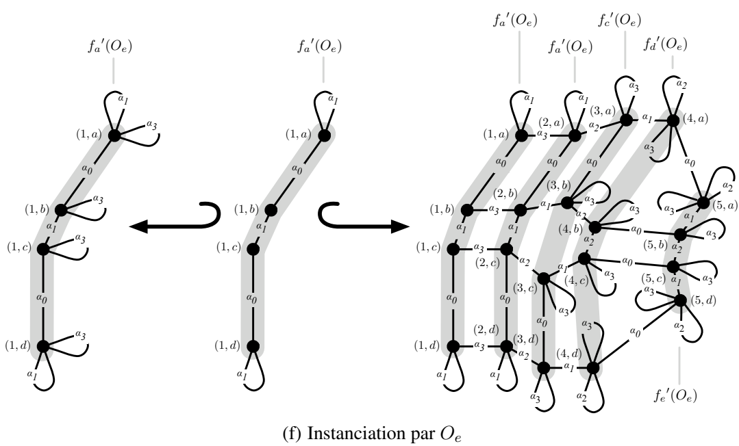
FIGURE 3.21 – Règles de cône avec renommages d'orbites
