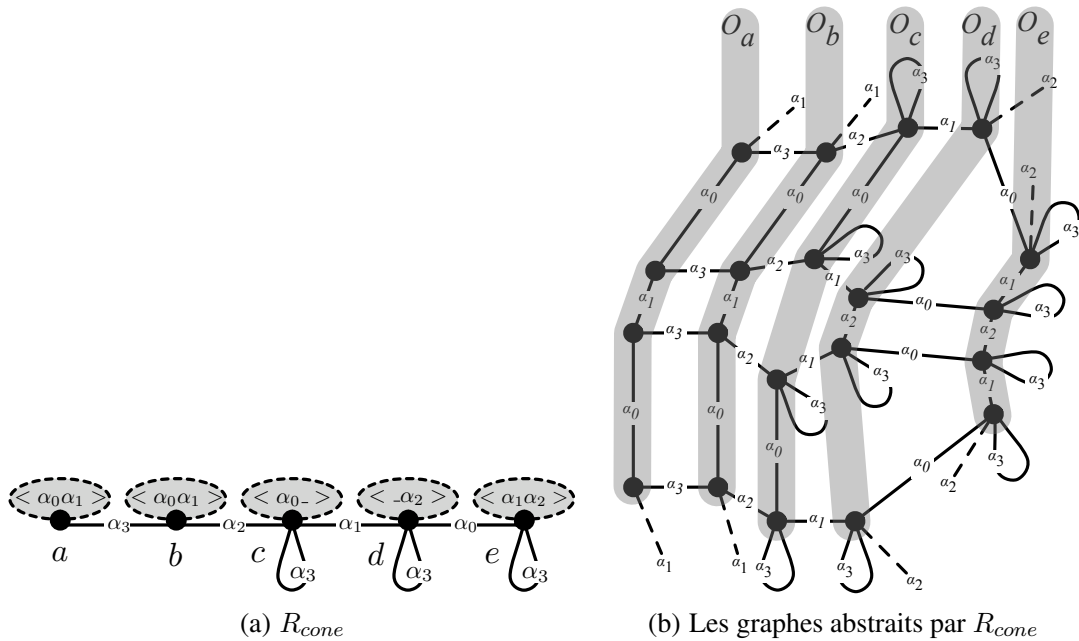
FIGURE 3.25 – Un graphe avec renommages R_{cone} et les graphes qu'il abstrait
