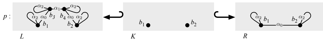
FIGURE 2.17 – Règle de fusion de deux arêtes dans une 2-G-carte
