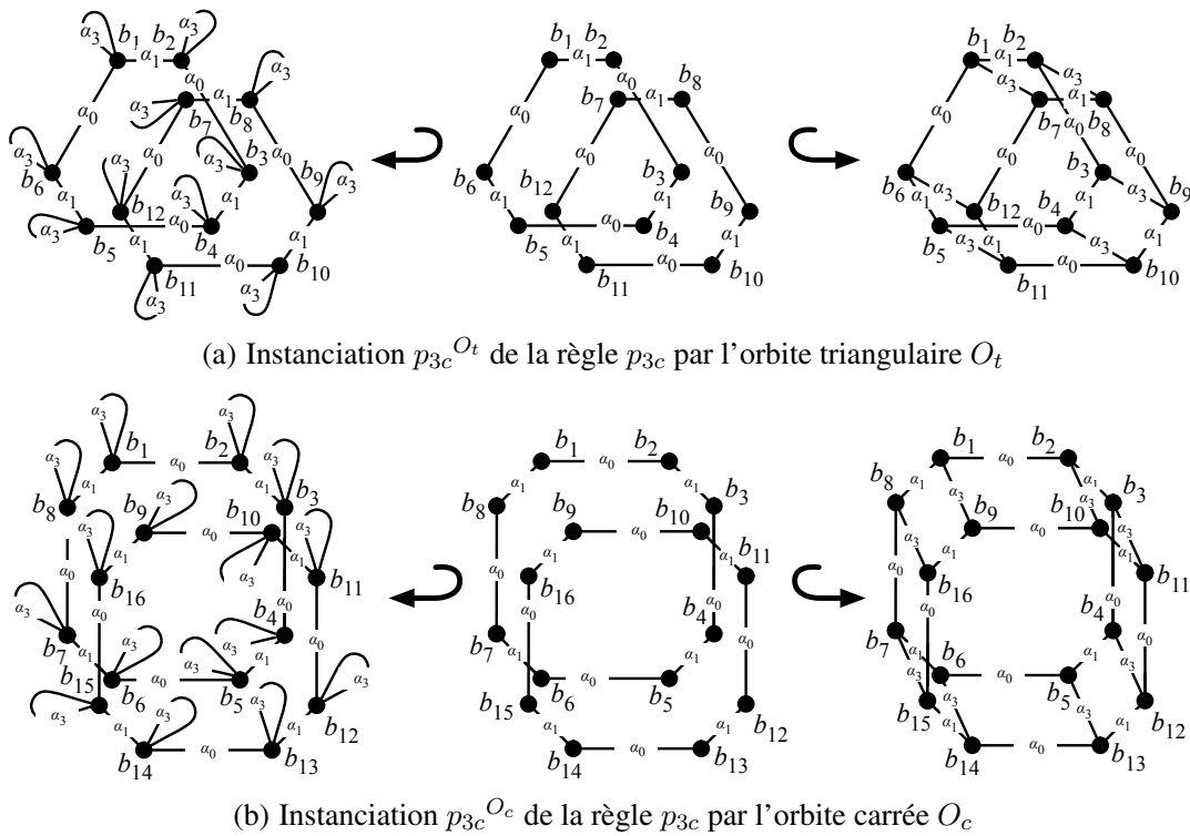
FIGURE 3.19 – Deux instanciations de la règle de transformation avec variable orbite p_{3c}
