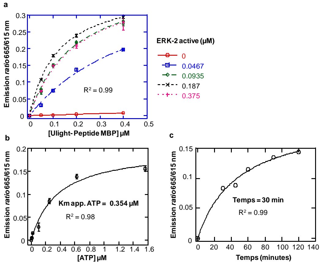
Figure 64 : Optimisation du test direct sur ERK-2 avec la méthode Lance Ultra™. Les coefficients de détermination R^2 et les barres d'erreurs représentant l'écart type obtenus après 3 essais sont indiqués. Les réactions kinase ont été arrêtées après 60 minutes à température ambiante par addition d'EDTA (40 mM). La phosphorylation du substrat Ulight_Peptide MBP est détectée après l'addition d'anticorps anti-phospho-Peptide MBP marqué à l'Europium (8 nM). Après 20 min d'incubation à température ambiante, les émissions de fluorescence sont enregistrées à 665 et 615 nm après une excitation à 340 nm avec un lecteur de plaque Victor V™. Les rapports des émissions de fluorescence 665/615 nm sont calculés pour chaque puits. (a) Optimisation de la concentration optimale de ERK-2 active. Les essais ont été réalisés en variant la concentration en ERK-2 active de 0 à 0,375 \mu\text{M} ainsi que la concentration en Ulight_Peptide MBP de 0 à 0,4 \mu\text{M} en présence de 10 \mu\text{M} d'ATP. (b) Titration de l'ATP. Les essais ont été réalisés aux concentrations fixes en ERK-2 active (0,187 \mu\text{M} ) et Ulight_Peptide MBP (0,1 \mu\text{M} ), en faisant varier la concentration d'ATP de 0 à 1.6 \mu\text{M} . (c) Vitesse de la réaction kinase. Les essais ont été réalisés aux concentrations optimisées d'ERK-2 active (0,187 \mu\text{M} ), d'Ulight_Peptide MBP (0,1 \mu\text{M} ) et d'ATP (0,354 \mu\text{M} ). Les réactions kinase ont été arrêtées aux temps indiqués par addition d'EDTA (40 mM).
