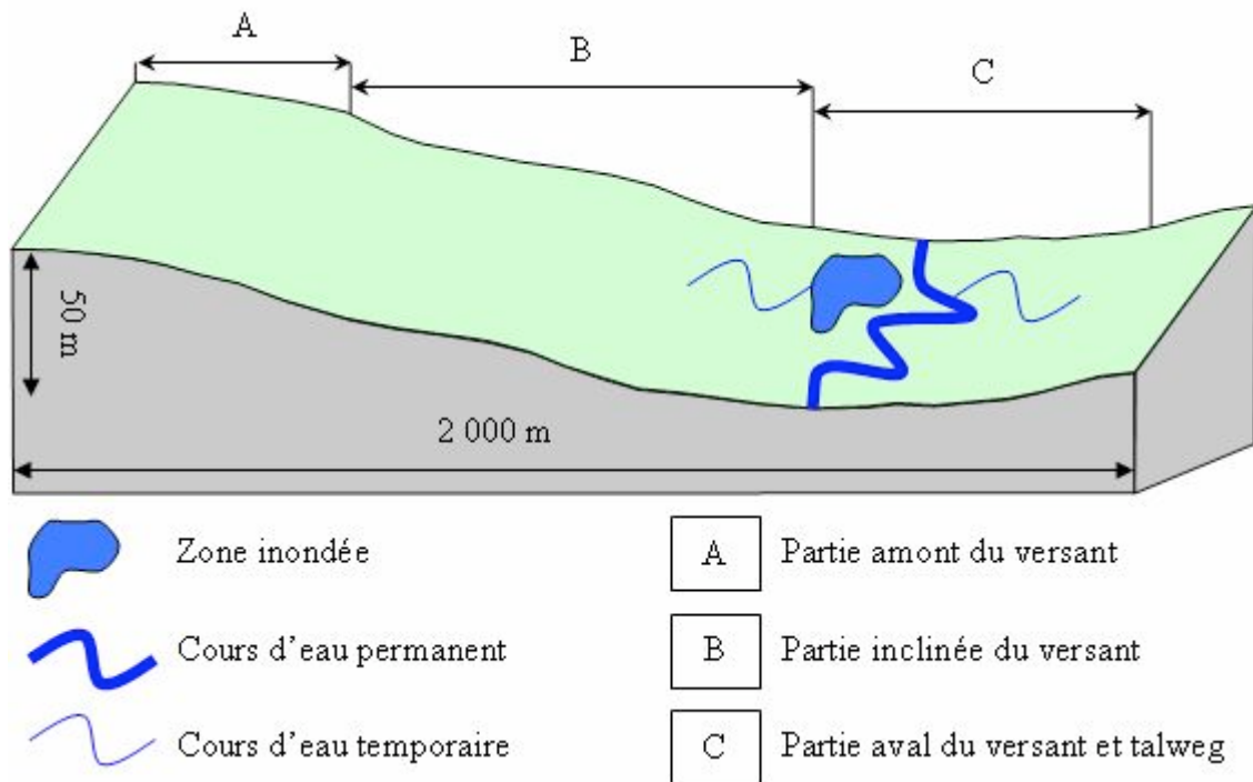
Figure 1.5 – Profil topographique d'un versant dans l'ensemble II de Benfica. Modifié de Maître d'Hôtel et Biri Kassoum (2002), et de Brand et Sicard (2003)
