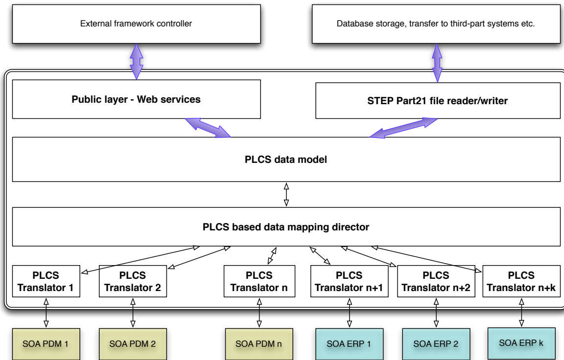
FIGURE 4.3.1.: Architecture fonctionnelle orientée Services
