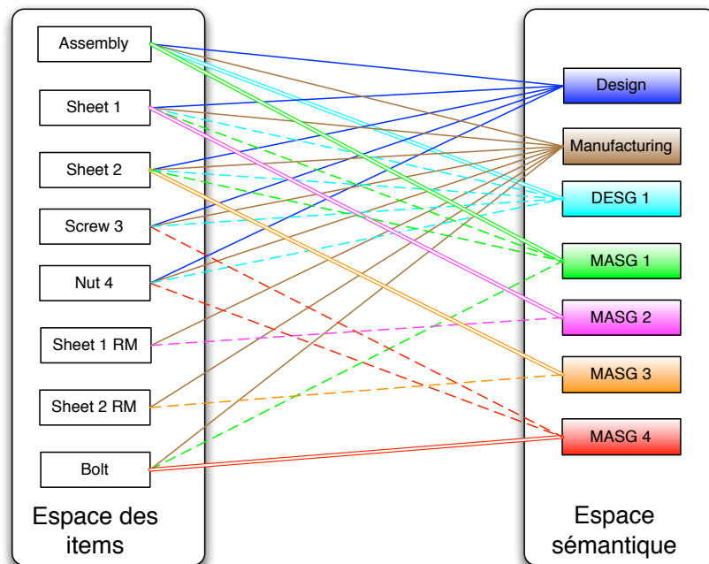
FIGURE 3.4.5.: Exemple d'instanciation du modèle de tags sémantiques
