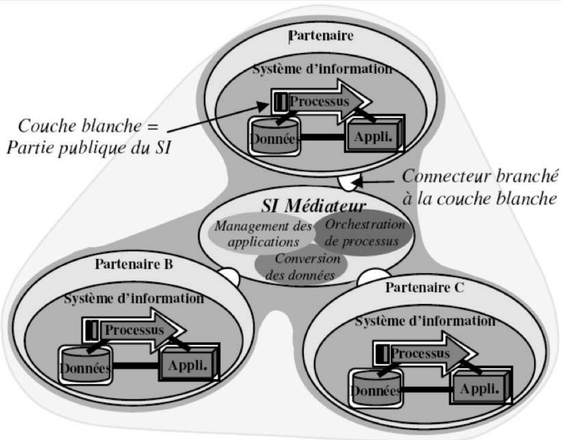
FIGURE 2.2.2.: Le médiateur d'informations orienté services selon [Bénaben et al., 2008]
