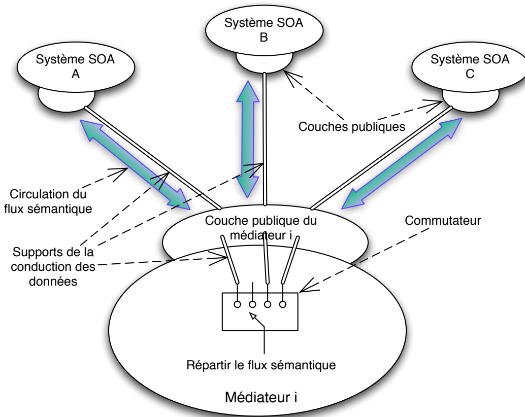
FIGURE 2.2.4.: Fonction de répartition d'un médiateur de la médiation multi-échelle
