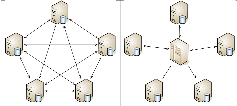
FIGURE 2.2.1.: Approches point-à-point/médiateur pour l'interopérabilité technique
