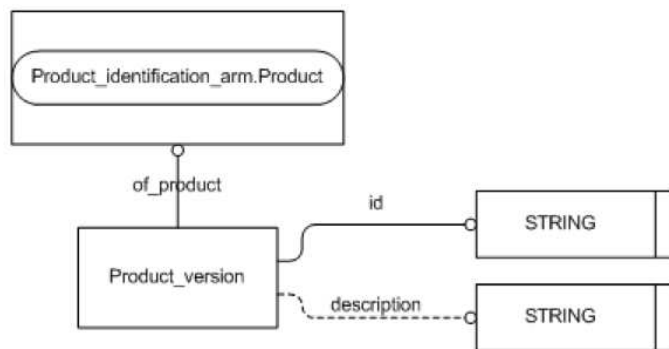
FIGURE 3.3.3.: Modélisation d'une version d'un produit
