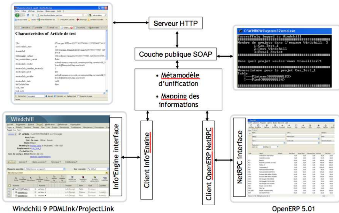
FIGURE 4.3.3.: Résultats de l'expérimentation pour l'interopérabilité PDM/ERP
