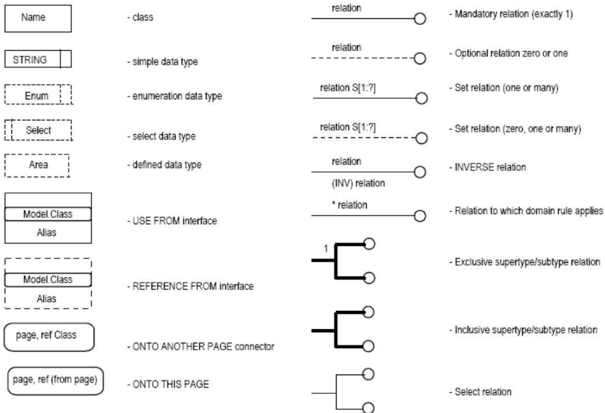
FIGURE B.6.1.: Syntaxe EXPRESS-G
