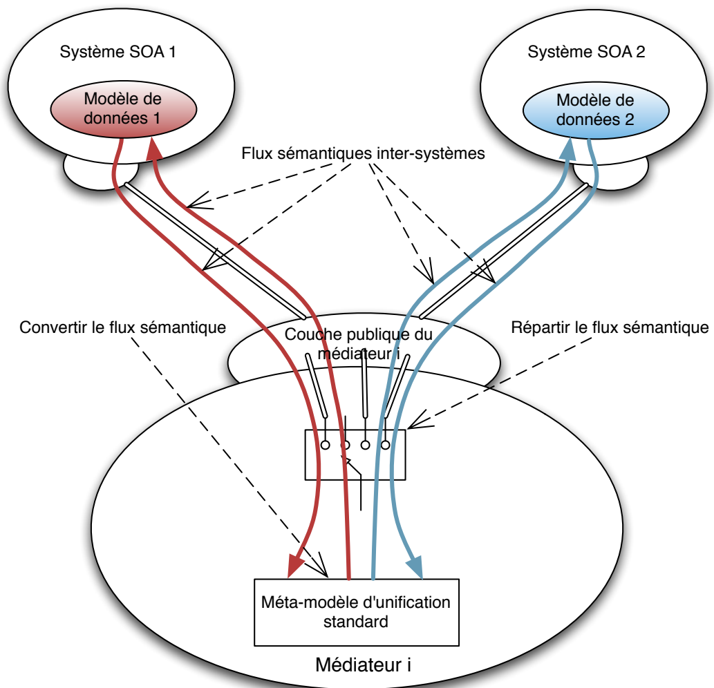
FIGURE 2.3.1.: Le médiateur multi-échelles orienté services - Unification des informations sémantiques
