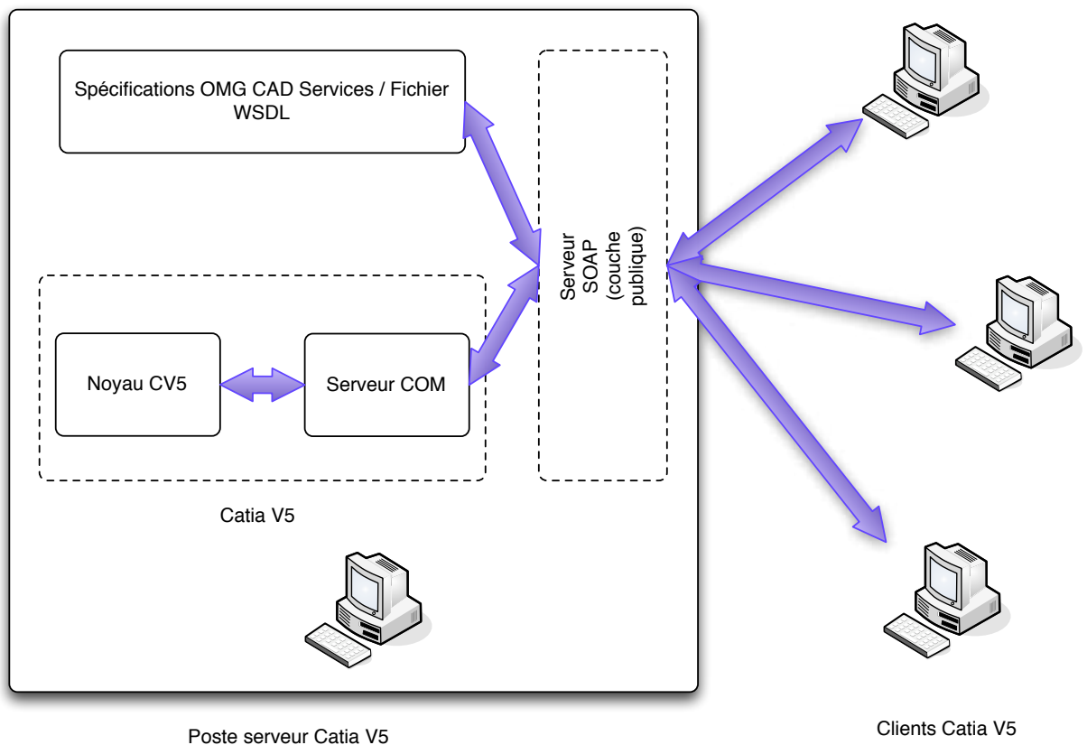
FIGURE 4.2.1.: Webservicisation du logiciel Catia V5
