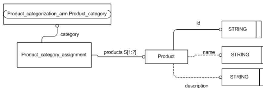
FIGURE 3.3.2.: Modélisation du produit dans STEP PLCS
