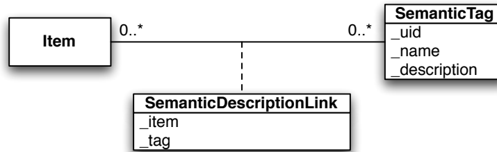
FIGURE 3.4.3.: Un premier modèle de données pour le tag sémantique
