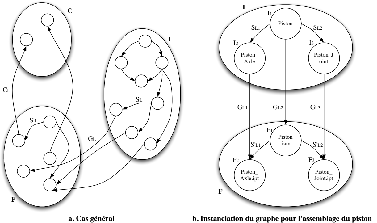
FIGURE 3.2.3.: Modèle graphe des dépendances entre fichiers CAO pour une maquette numérique
