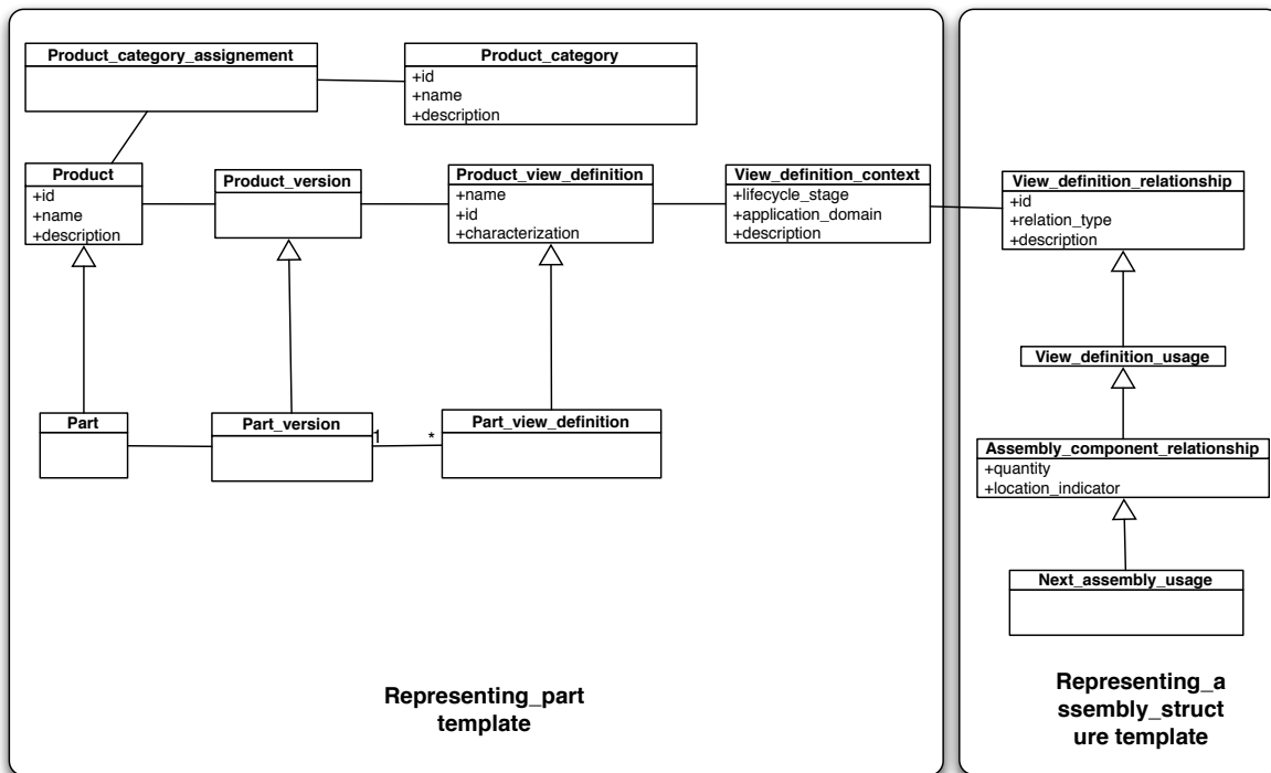
FIGURE 3.3.7.: Diagramme UML pour le méta-modèle d'unification
