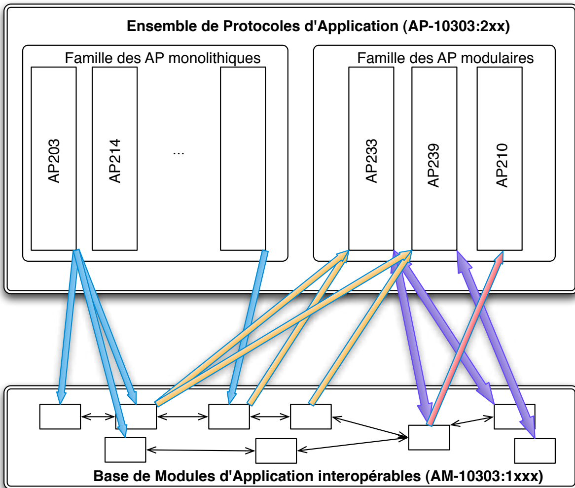
FIGURE 2.3.4.: La modularité de la norme STEP : Modules d'Application (AM) et Protocoles d'Application (AP)
