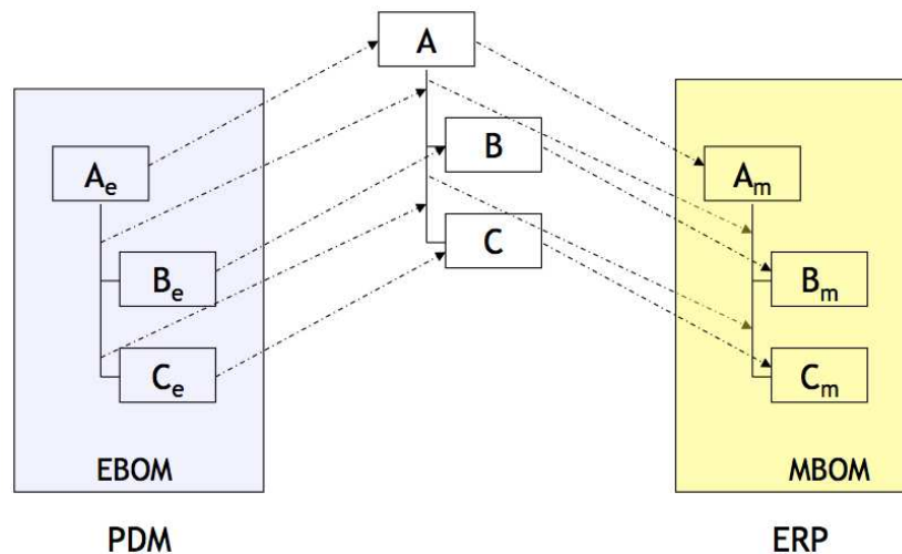
FIGURE 4.3.2.: Mapping entre les nomenclatures PDM et ERP
