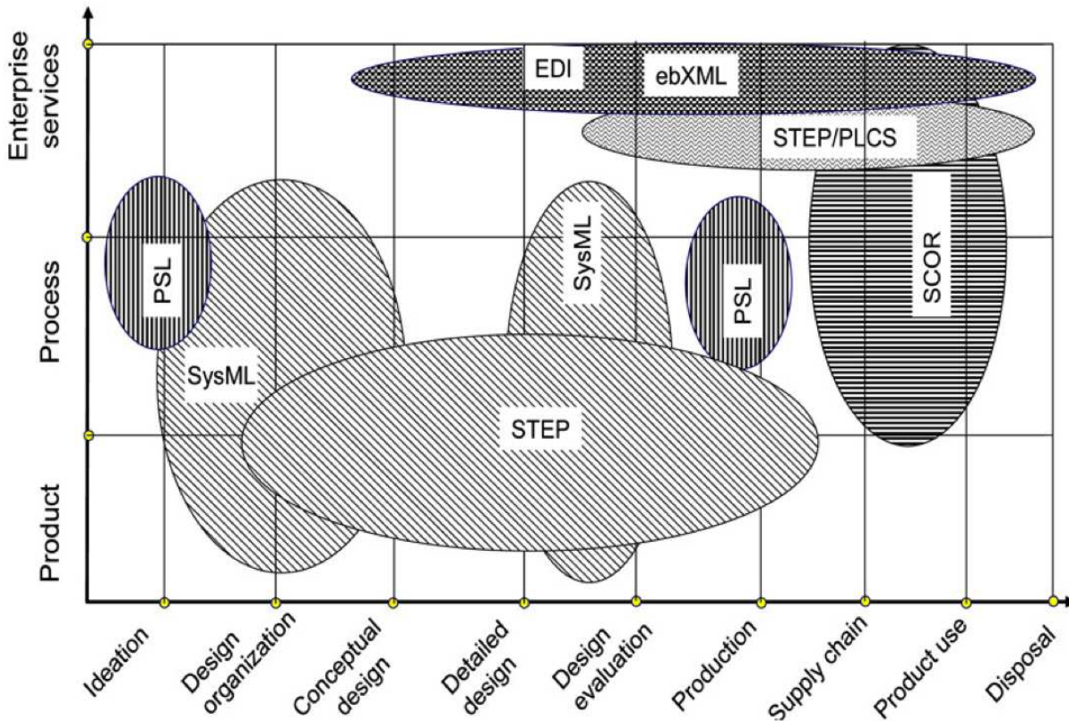
FIGURE 2.3.2.: Cartographie 2D des standards du PLM [Rachuri et al., 2008]
