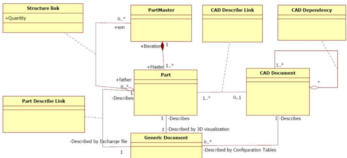
FIGURE 3.2.7.: Méta-modèle d'unification pour l'interopérabilité CAO/PDM
