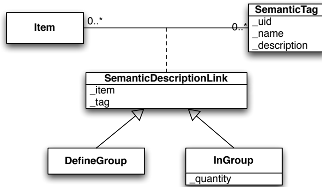
FIGURE 3.4.4.: Modèle de données pour le groupe sémantique
