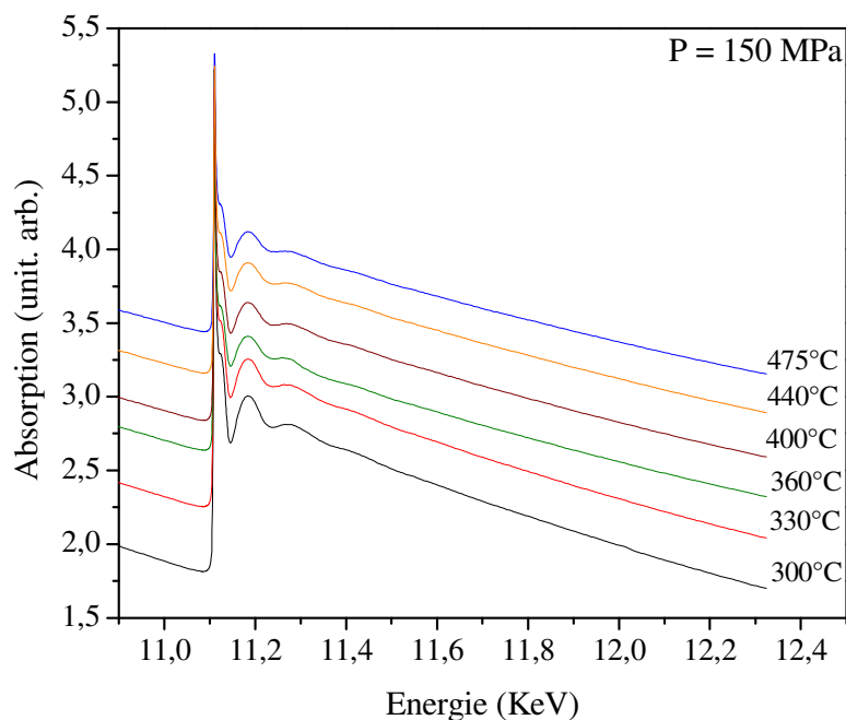
Figure IV.2. Spectres XAS bruts en transmission d'une solution de NaOH 0,5M en contact avec Si_{0,8}Ge_{0,2}O_2 type cristobalite à 150 MPa entre 300°C et 450°C. Par soucis de clarté, les spectres ont été arbitrairement décalés verticalement.
