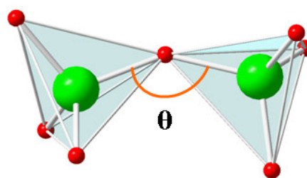
Figure I.2.b: Angle de pont \theta inter-tétraèdres
