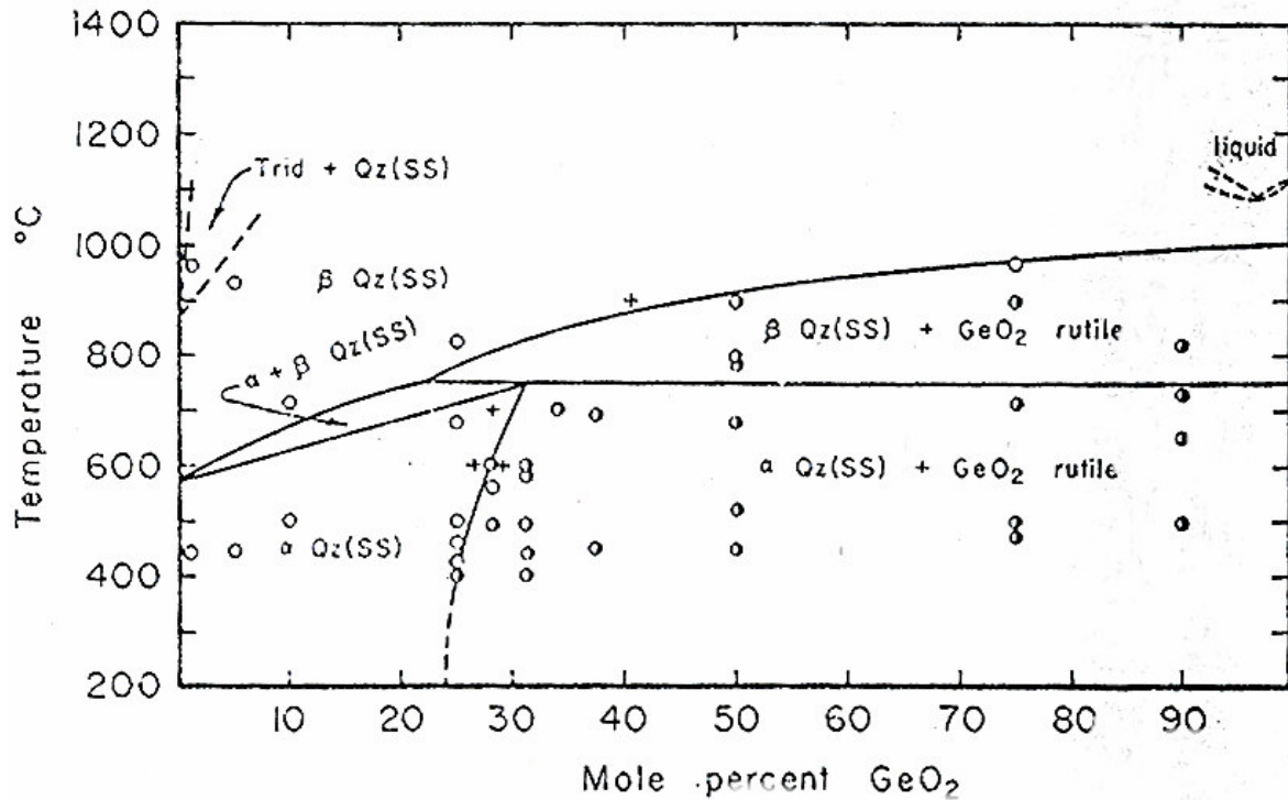
Figure I.7: Diagramme de phase T-x à 70 MPa du système \text{SiO}_2\text{-GeO}_2 proposé par Miller et al. 26
