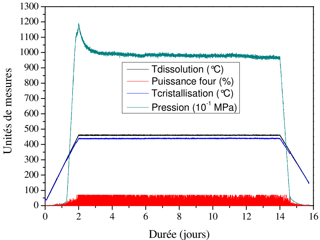
Figure III.7. Enregistrement des paramètres thermodynamiques d'un cycle de croissance
