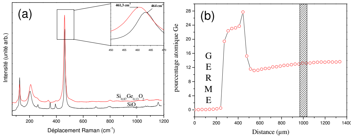
Figure V.6. (a) Spectre Raman du quartz- \alpha et de \text{Si}_{0,87}\text{Ge}_{0,13}\text{O}_2 de type quartz- \alpha (b) cartographie par microsonde électronique du cristal QVM15, l'éclat étudié par diffraction des RX est issu de la zone hachurée.
