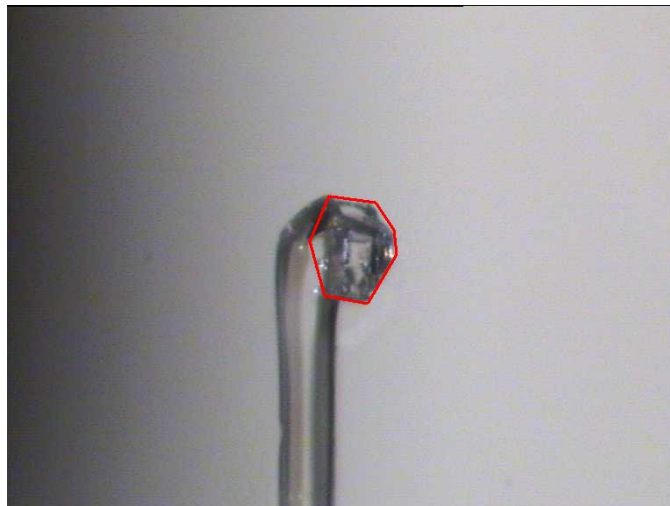
Figure II.12. Montage d'un éclat de monocristal sur un capillaire de silice. Les faces du cristal sont délimitées par un trait continu.
