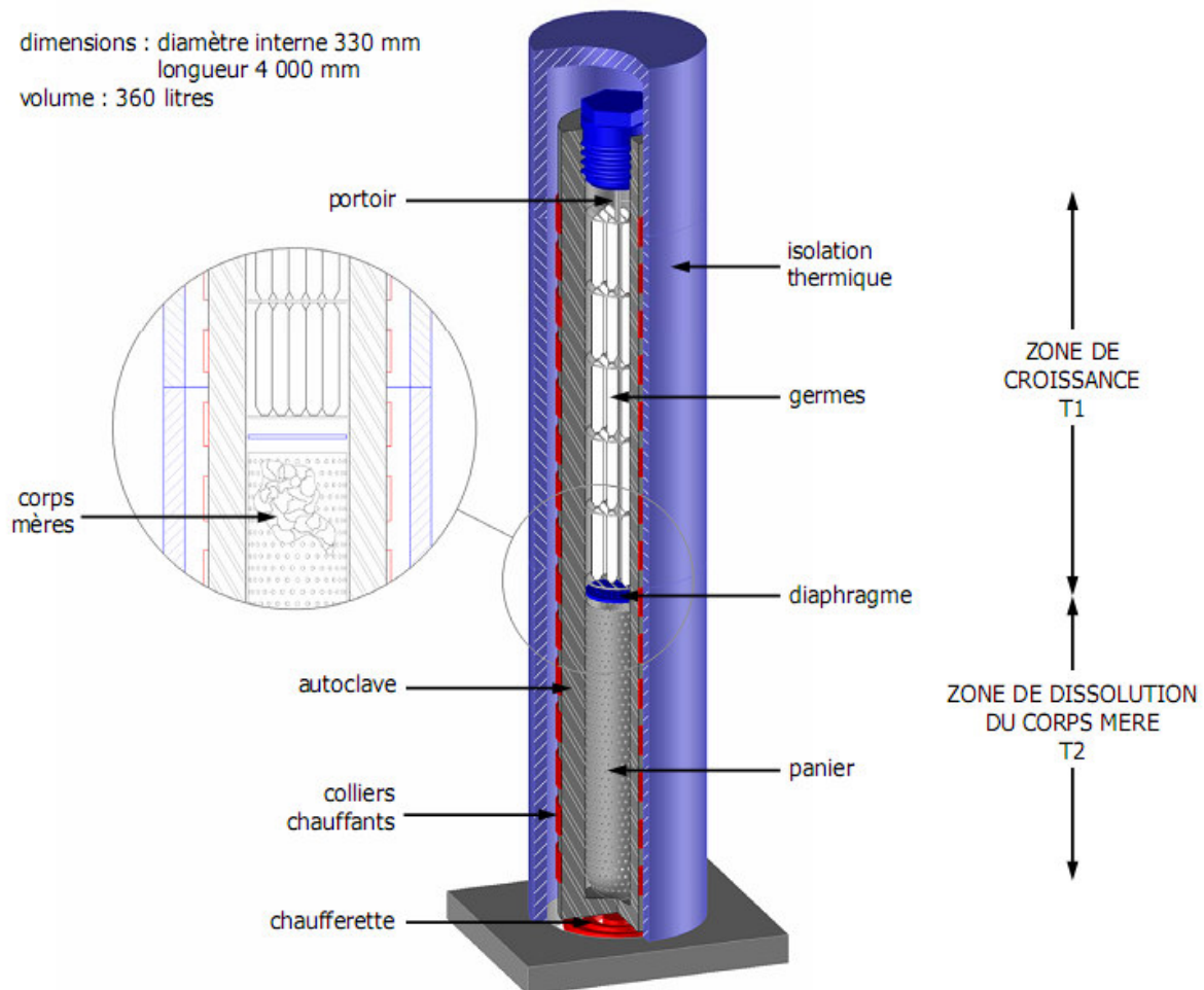
Figure II.1: Représentation schématique d'un autoclave
