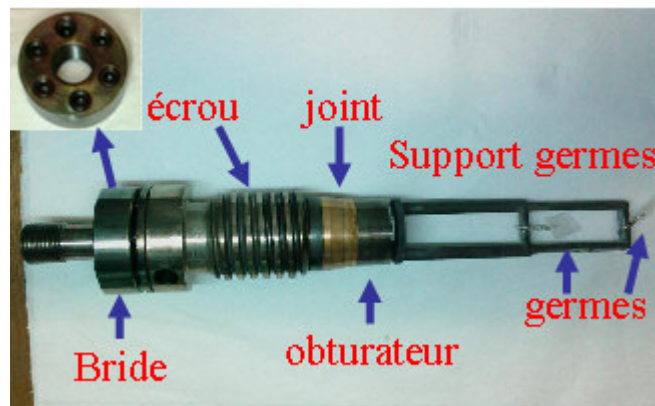
Figure II.3: Système de fermeture des autoclaves
