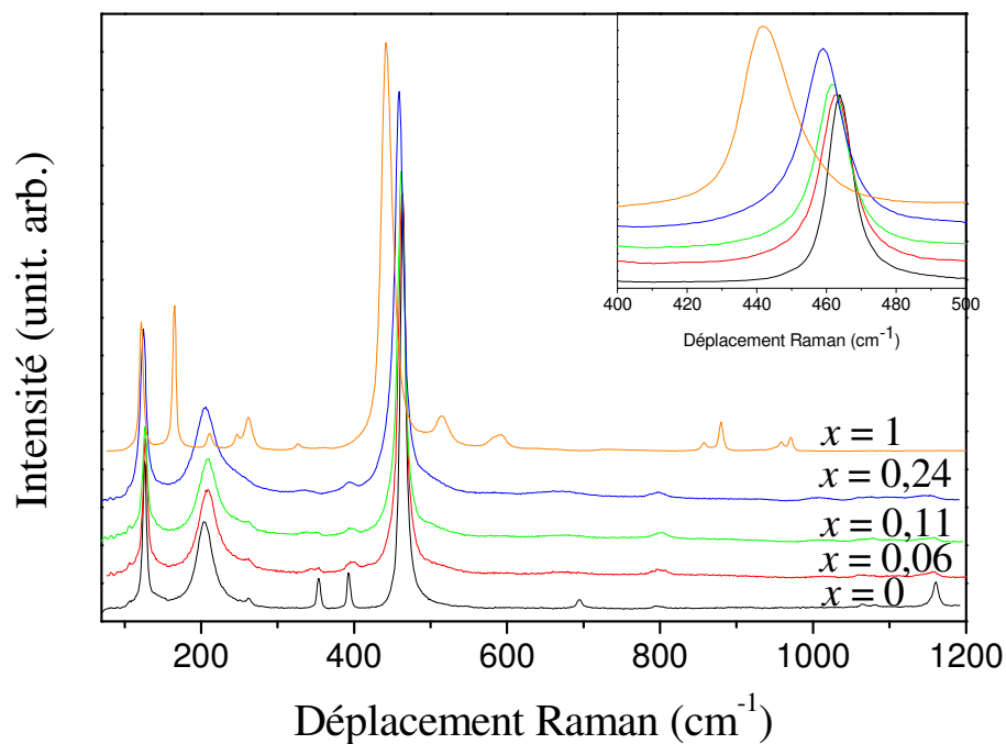
Figure V.2. Spectres Raman de \text{Si}_{1-x}\text{Ge}_x\text{O}_2 type quartz- \alpha en fonction de la composition
