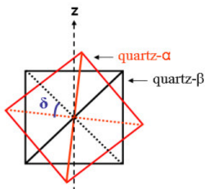
Figure I.2.a: Angle de rotation \delta des tétraèdres
