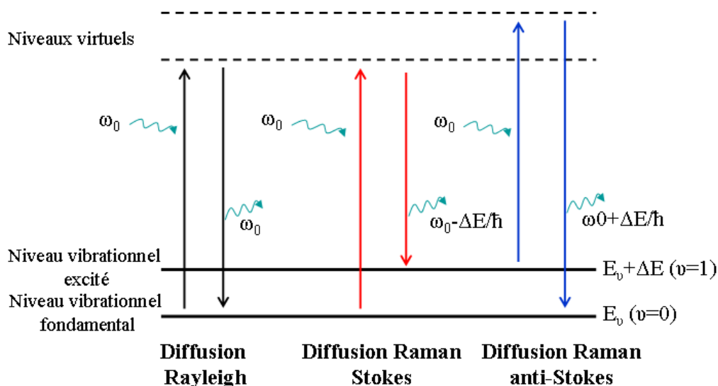
Figure II.13. Schéma de principe des processus de diffusion Rayleigh, Raman Stokes et Anti-Stokes
