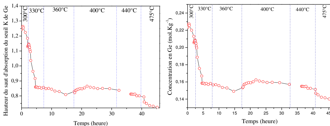
Figure IV.3. Hauteur du saut de seuil mesurée en transmission au seuil K de Ge à différentes températures en fonction du temps
