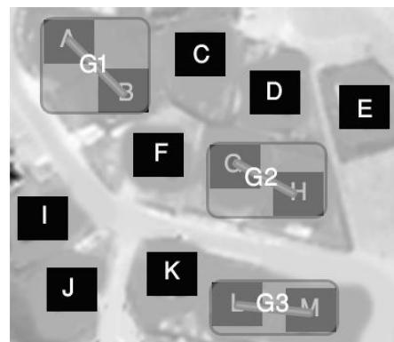
Figure III. 15. Première étape de construction du graphe de voisinage spatial
