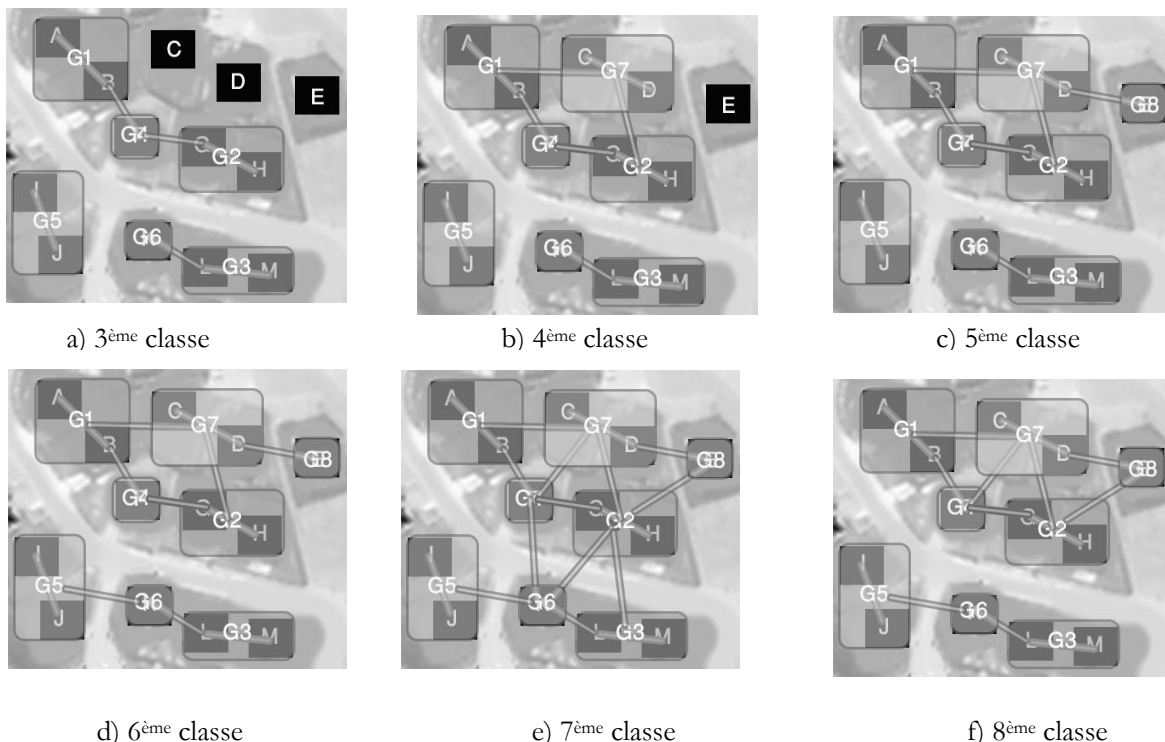
Figure III. 17. Étapes de construction du graphe de voisinage spatial
