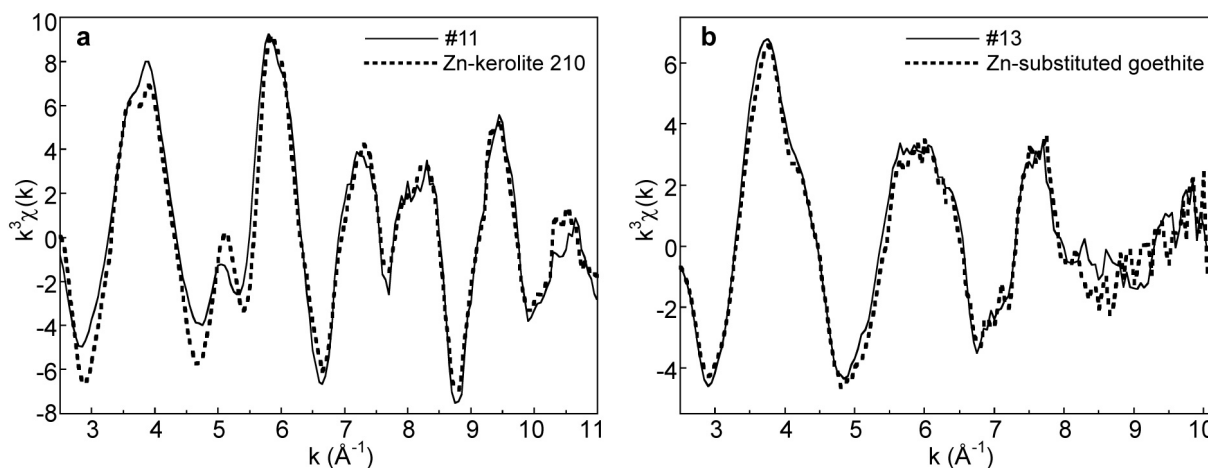
Figure V.5. Spectres \mu EXAFS au seuil K de Zn enregistrés dans les points 11 et 13 (trait plein) et les spectres des références (trait pointillé) de Zn-kérolite et de Zn-goéthite substituée (a,b).
