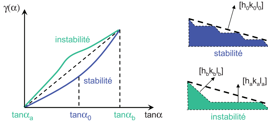
FIGURE 1.9 – Allure générale de l'énergie de surface dans le cas d'une surface vicinale stable (en bleu) et instable (en vert). (RAOUAFI et al., Phys. Rev. B 66, 045410 (2002); DESJONQUÈRES et al., Phys. Rev. Lett. 88, 056104 (2002)).
