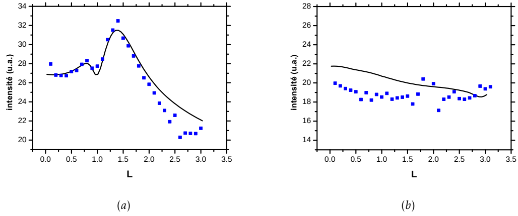
FIGURE 3.29 – Facteurs de structure suivant les tiges de diffusion (a) ( 2 \times 5 ) et (b) ( 8 \times 3 ) pour un dépôt d'argent de 8 minutes. Les points représentent les données expérimentales, les traits pleins les simulations QMD pour une monocouche d'argent sur une surface Ni(111), reconstruite (\sqrt{52} \times \sqrt{52})R13.9^\circ .
