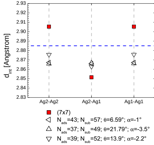
FIGURE 3.11 – Moyennes des distances premiers voisins en Å calculées pour une bicouche d’argent adsorbée formant les différentes reconstructions (7x7), (\sqrt{52} \times \sqrt{52})R13,9^\circ (avec N_{ads} = 39 et \alpha = -2,2^\circ ), (7 \times 7)R21,79^\circ (avec N_{ads} = 37 et \alpha = -3,5^\circ ) et (\sqrt{57} \times \sqrt{57})R6,59^\circ (avec N_{ads} = 43 et \alpha = -1^\circ ). Les distances Ag2-Ag2 correspondent aux distances calculées dans le plan de la surface (seconde couche d’argent), Ag1-Ag1 dans le plan de la couche d’argent à l’interface avec le substrat et Ag2-Ag1 entre les deux couches d’argent.
