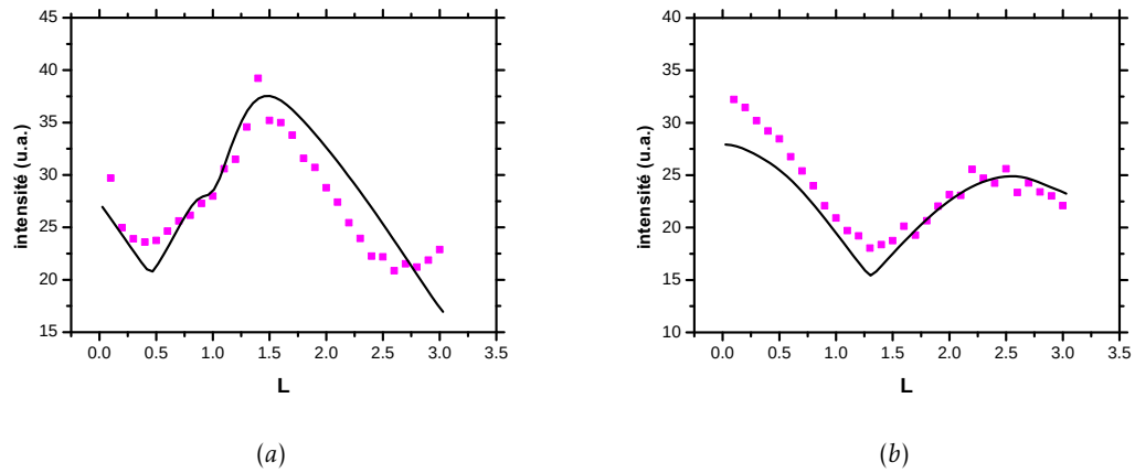
FIGURE 3.30 – Facteurs de structure suivant les tiges de diffusion (a) ( 2 \times 5 ) et (b) ( 8 \times 3 ) pour un dépôt d'argent de 20 minutes. Les points représentent les données expérimentales, les traits pleins les simulations QMD pour 0,7 monocouche et 0,3 bicouche d'argent sur une surface Ni(111) reconstruite (\sqrt{52} \times \sqrt{52})R13,9^\circ .
