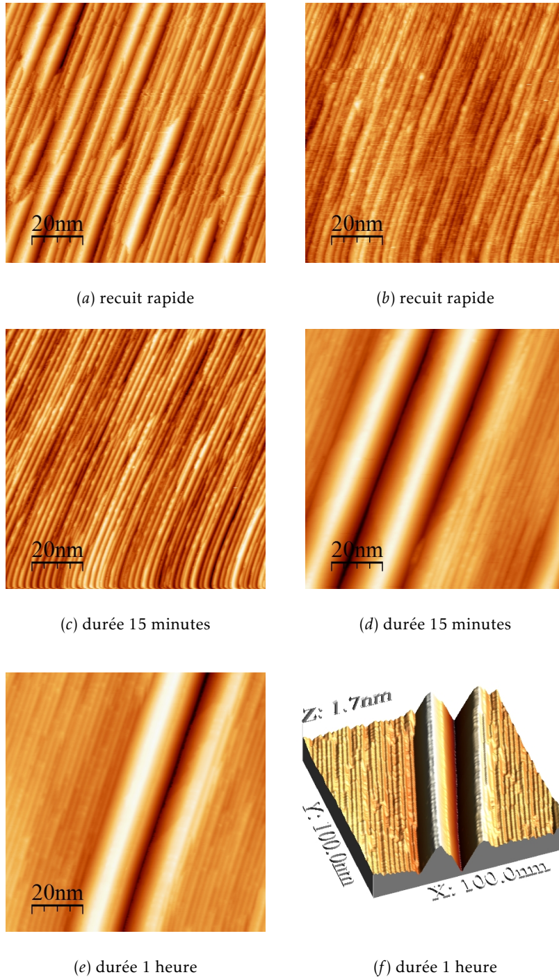
FIGURE 4.19 – Images STM ( 100 \times 100 \text{ nm}^2 ) de la surface Ni(322) après dépôt de 0,3 MC d'argent et recuit : (a) et (b) recuit rapide à 600 K, sur deux régions différentes de l'échantillon ; (c) et (d) recuit de 15 minutes à 600 K, sur deux régions différentes de l'échantillon ; (e) recuit supérieur à 1 heure à 600 K, (f) représentation en trois dimensions de l'image (e).
