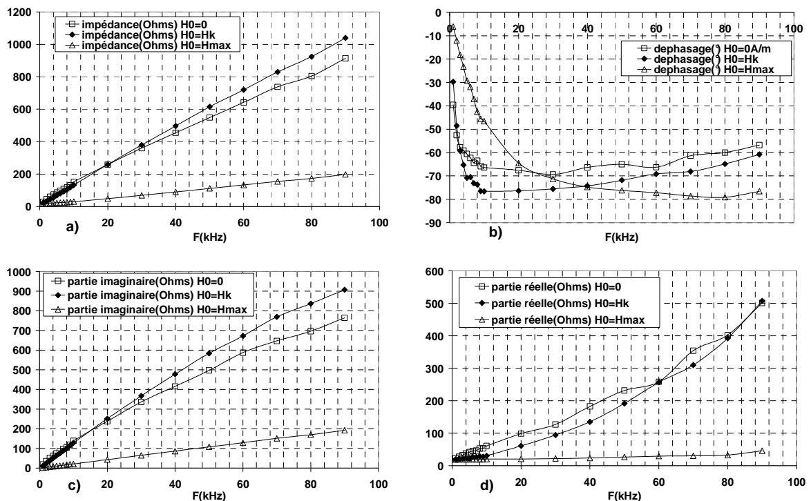
Figure 2.17 : Impédance GMI sandwich à bobinage longitudinal en fonction de la fréquence : a) Module, b) Phase, c) Partie imaginaire, d) Partie réelle.
