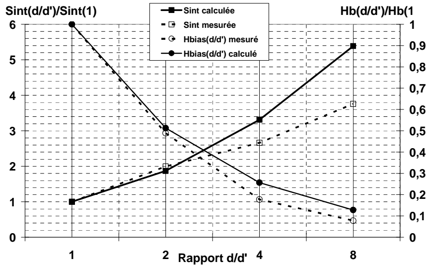
Figure 2.37 : Mesure de la sensibilité intrinsèque normalisée et du champ de polarisation normalisé en fonction du rapport d'amincissement des rubans mumetal.
