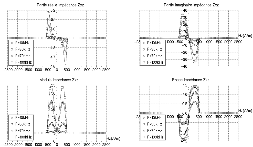
Figure 4.24 : Impédance GMI bobinée Z_{xz} en fonction du champ magnétique. Valeur des paramètres : \gamma=2.10^{11} m/A.s, \alpha=0.1 , M_s=1.6.10^6 A/m, N_x=30.10^{-5} , \sigma=1.10^6 S et H_{kx}=500 A/m.
