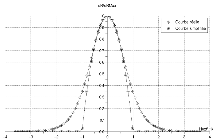
Figure 1.9 : Calcul de la variation de la résistance d'une AMR ( k_{\theta}=0.7 , H_k=550A/m ).
